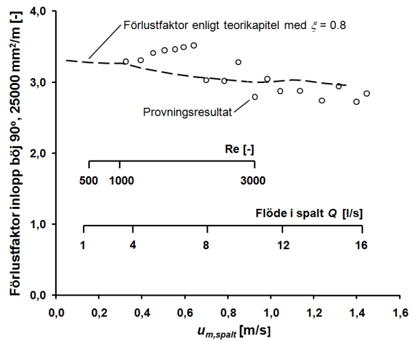
Figur 4-9 Förlustfaktor för inlopp med bøj 90° och tvärsnittsarea 25000 mm 2 /m.
