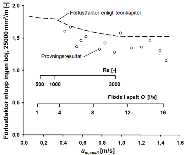
Figur 4-8 Förlustfaktor för inlopp utan bøj och tvärsnittsarea 25000 mm 2 /m.
