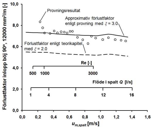
Figur 4-10 Förlustfaktor för inlopp med bøj 90° och tvärsnittsarea 12000 mm 2 /m.
