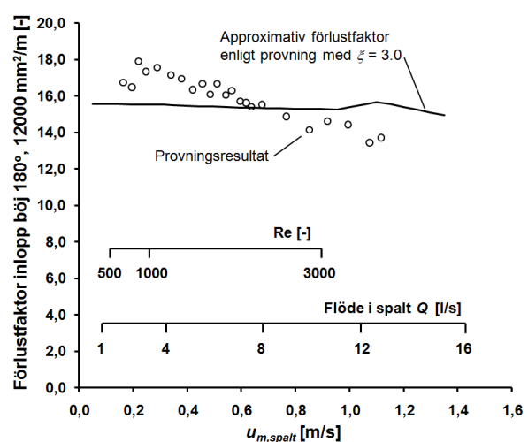
Figur 4-11 Förlustfaktor för inlopp med bøj 180° och tvärsnittsarea 12000 mm 2 /m.
