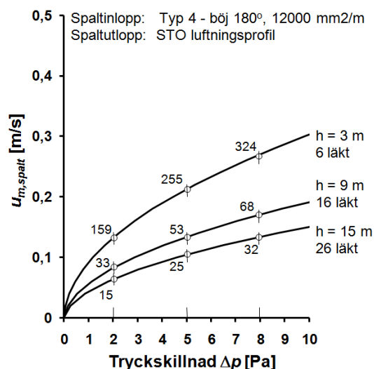
Figur 5-4 Spalt med läkt typ Lindab
