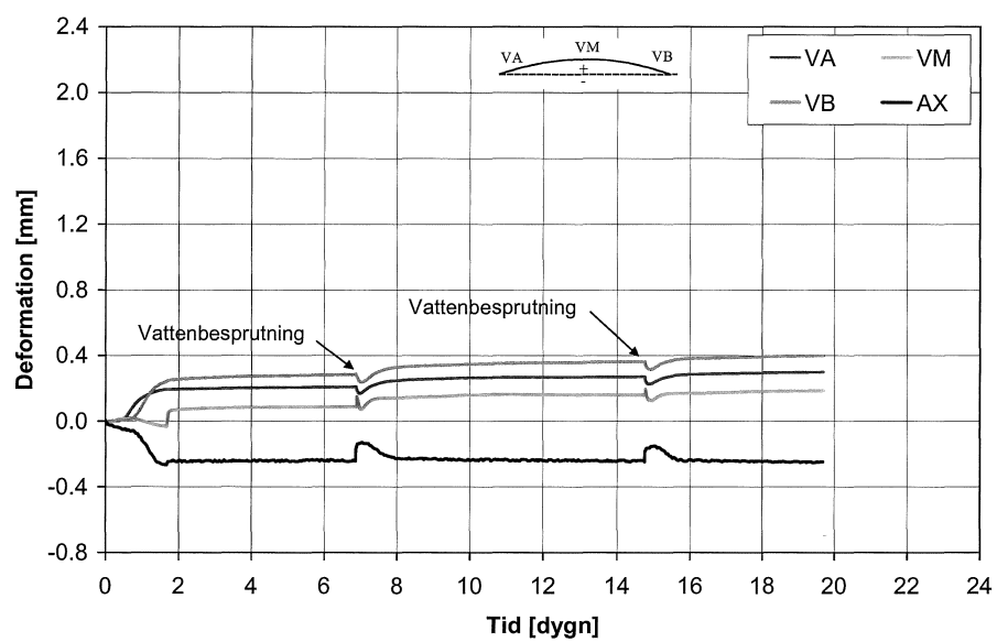
Figur 22 Deformationer hos förankrad 10 mm enkelarmerad putsremsa på isolering. Stålnät nära insidan.
