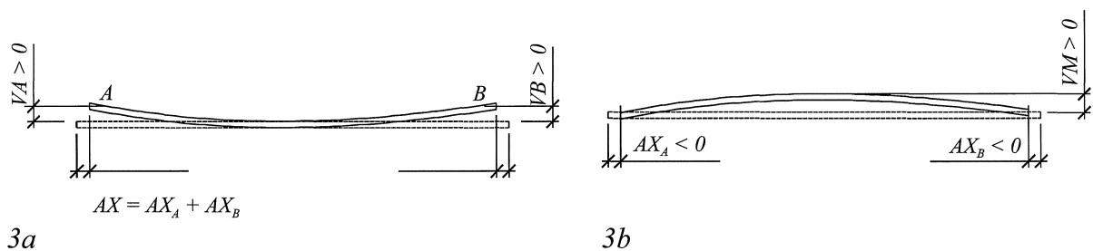
Figur 3 Axiell deformation ( AX ) och deformationer vinkelräta mot putsremsans längdaxel ( VA , VB och VM ).
