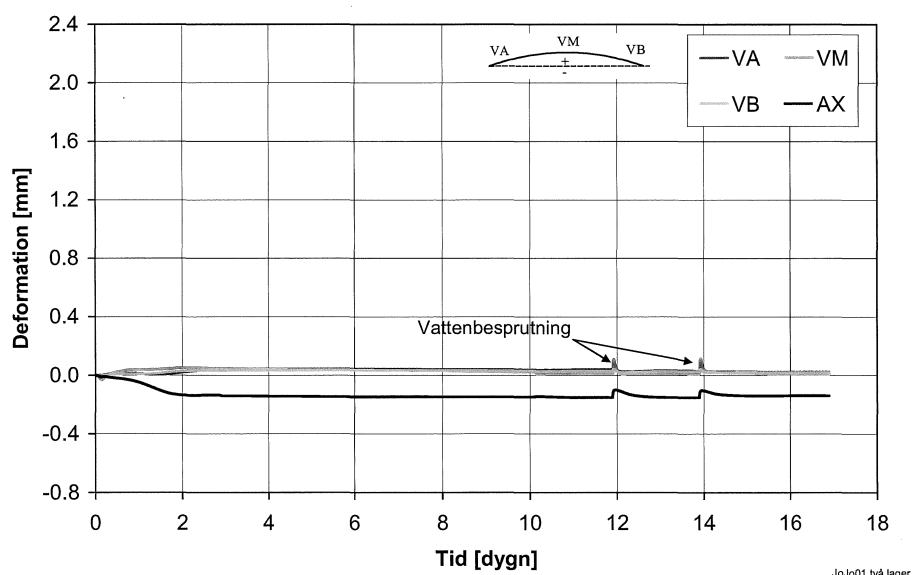
Figur 6 Deformationer hos 10 mm dubbelarmerad putsremsa. Stålnätarmering.
