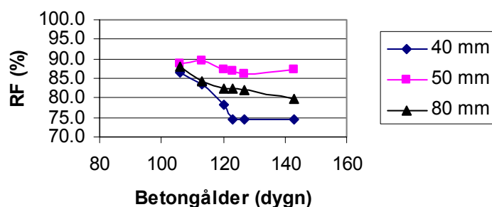
Betong-RF Rum 1:8
