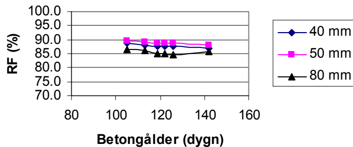
Betongtemperatur Rum 1:5
