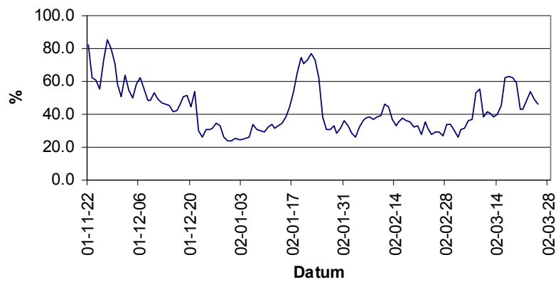
RF Rum 1:7
