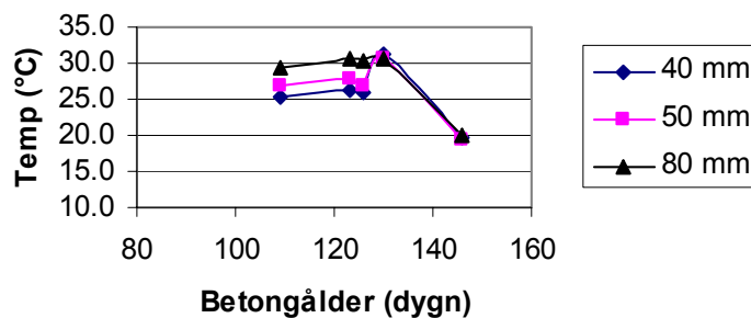
Betong-RF Rum 1:4
