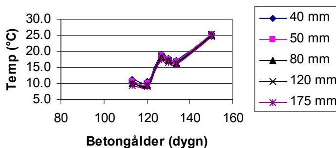
Betongtemperatur Rum 1:9 (vot)
