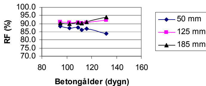
Betongtemperatur Rum 2:9
