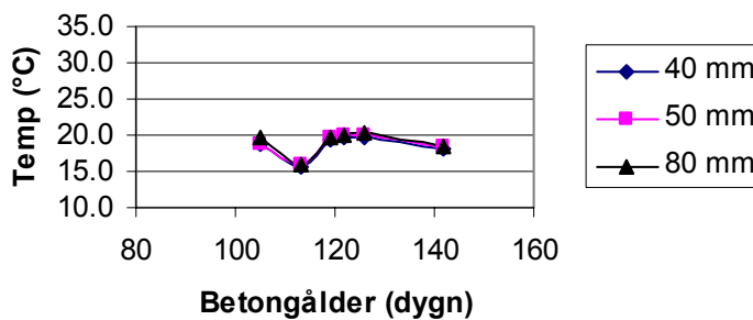
Betongtemperatur Rum 1:4
