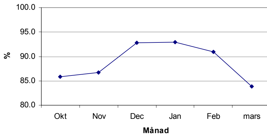
Figur 7.3. Månadsmedel-RF utomhus
