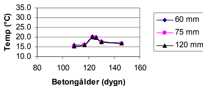
Betongtemperatur Rum 1:11
