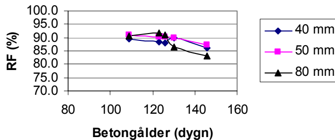
Betongtemperatur Rum 1:3
