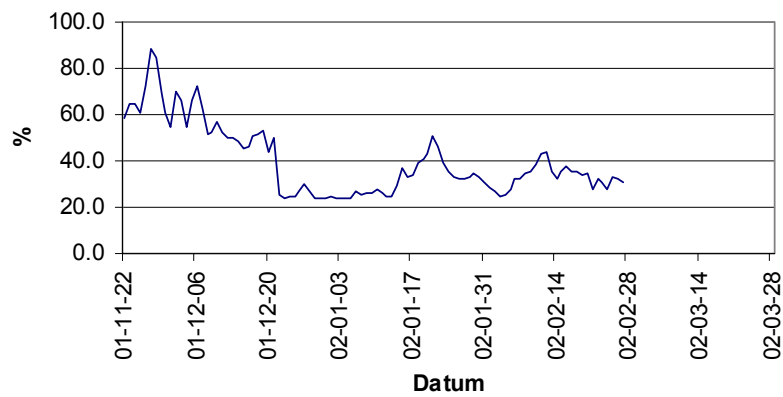
RF Rum 1:13
