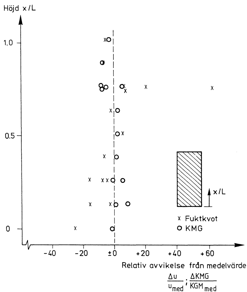
FIG 4. Exempel på mätning av fuktkvotsfördelning i en betongplatta där man erhåller en fuktkvotsgradient nedåt, utan att det pågår någon fukttransport nedåt. Mätning av KMG ger korrekt besked.
