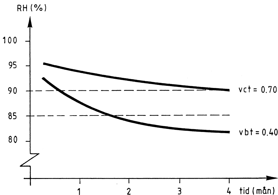
Figur 6.2. Uppmätta tidsförlopp för RH hos betongplattor med olika vattencementtal (vct)/vattenbindemedelstal (vbt). Betongerna är tillverkade med Slite standardcement. Betongen med vct = 0,70 har vattenhärdats i 28 dygn. Betongen med vbt = 0,40 (en s k självtorkande betong), vilken innehåller 5% silikastoft, har vattenhärdats i två månader. Efter härdningen har betongerna lagrats i klimatrums med 60% RH och 18°C. Torktiderna är som synes starkt knutet vct/vbt. (Hedenblad, 1994)
