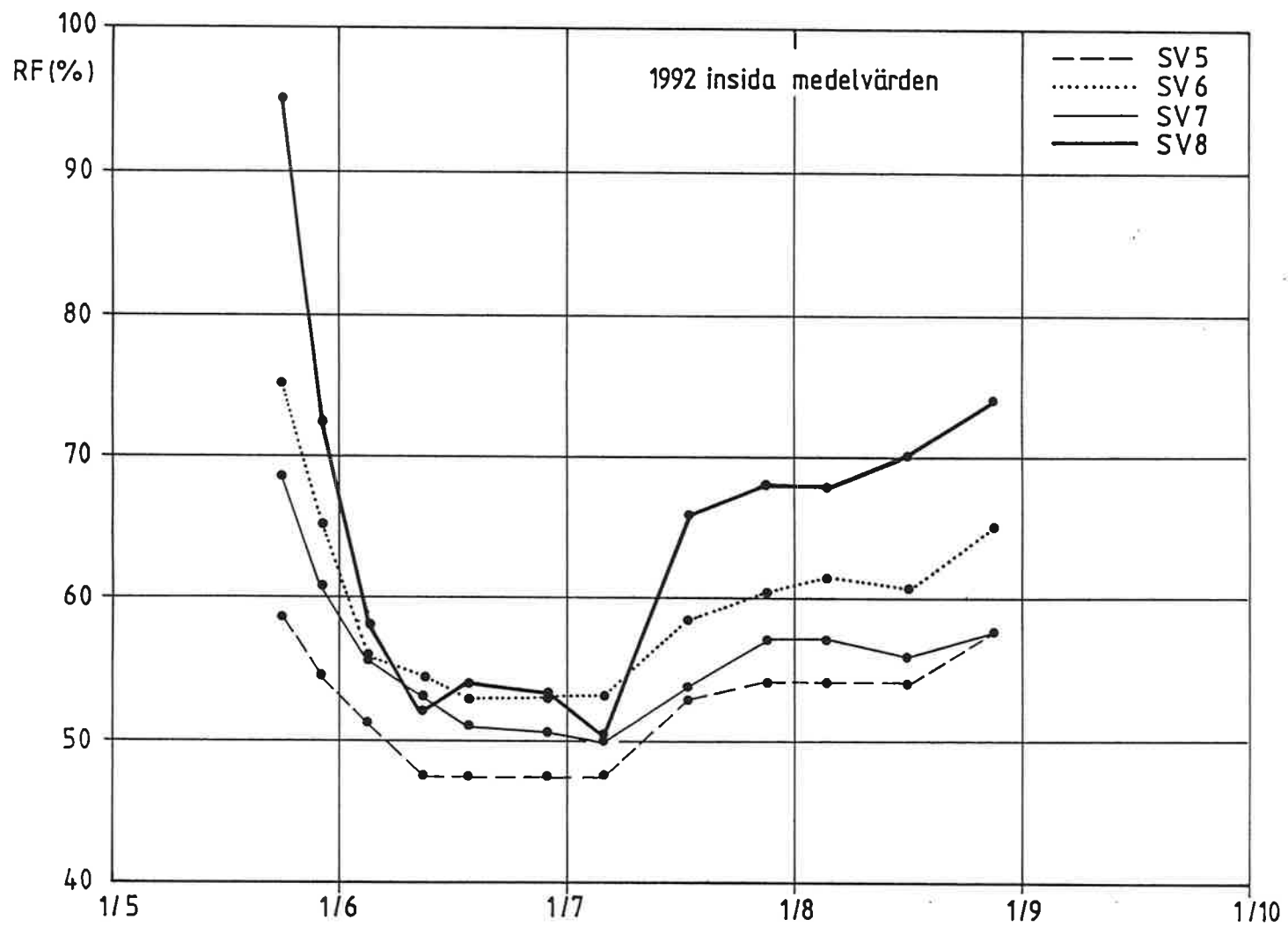
FIG 2. Medelvärden under 6-10 dygnsperioder. Inside 1992.
