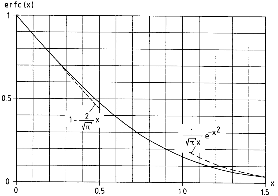
Figur 3.4. Funktionen \operatorname{erfc}(x) .
