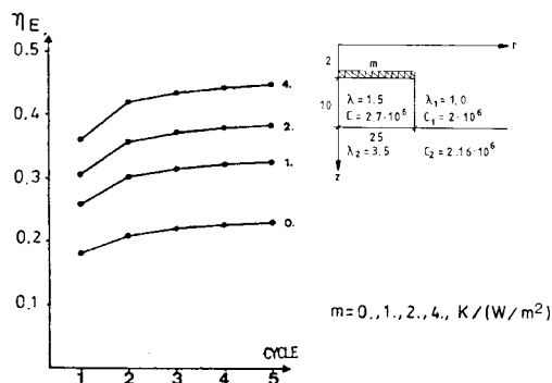
Figur 8.4.9-14. Energiverkningsgrad under de fem första års cyklerna för olika isoleringen m ( \text{K/(W/m}^2\text{)} ). Data enligt referensfallet fränsett tjockleken D på täckande skikt och höjden H på lagervolymen.
