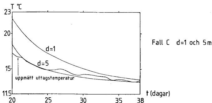
Figur 8.7.31. Uttagstemperatur för fall C.
