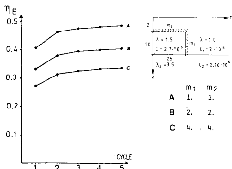
Figur 8.4.9-14. Energiverkningsgrad under de fem första års cyklerna för olika isoleringen m ( \text{K/(W/m}^2\text{)} ). Data enligt referensfallet fränsett tjockleken D på täckande skikt och höjden H på lagervolymen.
