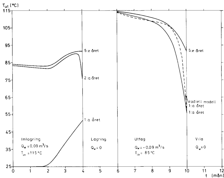
Figur 8.7.14. Uttagstemperatur för brunnspär enligt fall 10 med brunnsvståndet 120 m. Under 0 < t < 4 mån ges temperaturen från returbrunnen och under 6 < t < 10 mån temperaturen från lagringsbrunnen.
