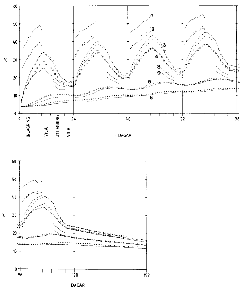
Figur 7.7.1. Uppmätta in- och utloppstemperaturer (kurvorna 1, 2; 8, 9) och uppmätta temperaturer i fyra punkter i berget på 13 meters djup (kurvorna 3, 4, 5, 6). Motsvarande beräknade värden ges av punkter.
