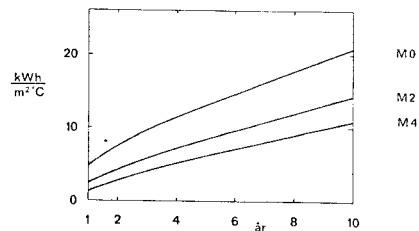
Figur 6.3.6.4 Ackumulerade värmeförluster för det större, långsträckta berggrummet.
