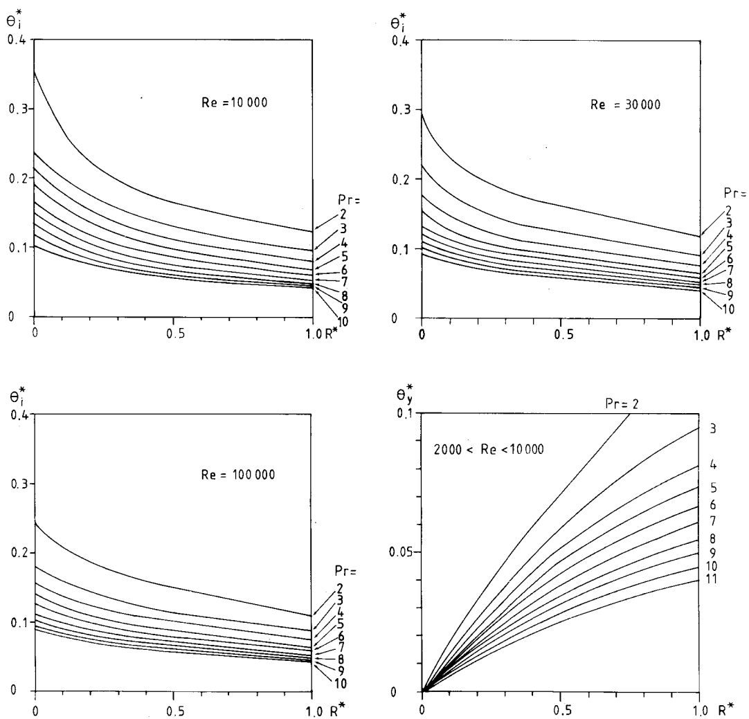
Figur 7.2.20 Influenstkoefficienten \theta_i^* i formel 7.2.106 för Re = 10\,000, 30\,000 och 100\,000 samt influenskoefficienten \theta_y^* i formel 7.2.107.
