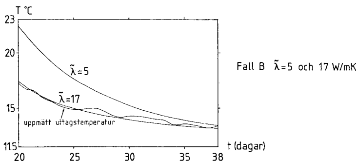
Figur 8.7.30. Uttagstemperatur för fall B.
