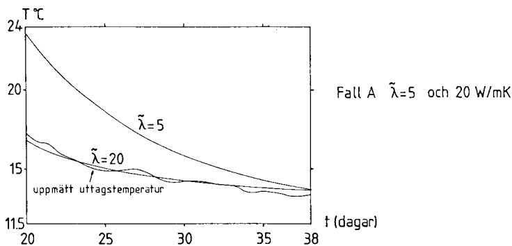
Figur 8.7.29. Uttagstemperaturen för fall A.
