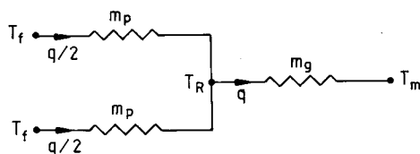
Figur 7.2.6 Värmeströmningskrets för markvärmesväxlare med två symmetriska värmesväxlarkana- ler.
