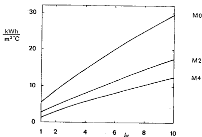
Figur 6.3.6.3 Ackumulerade värmeförluster för det mindre, långsträckta berggrummet.
