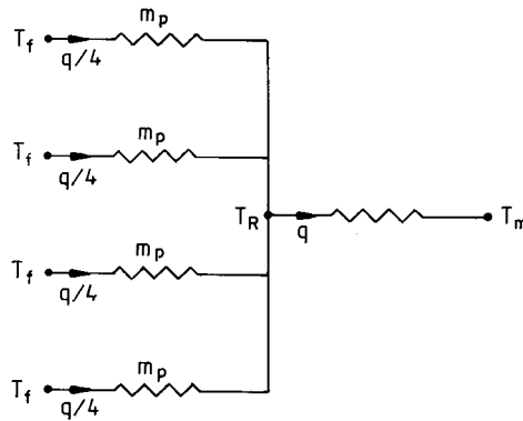
Figur 7.2.7 Värmeströmningskrets för markvärmesväxlare med fyra symmetriska värmesväxlarkanalerna.
