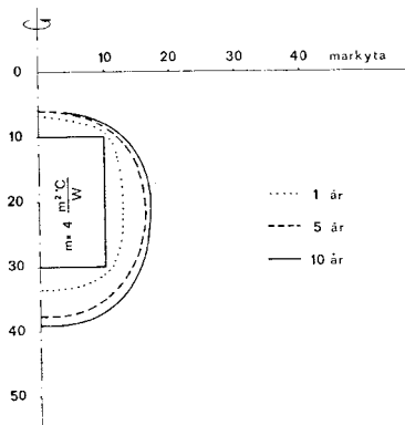
Figur 6.3.6.6 15 °C-isotermen som funktion av tiden. Lagret är isolerat med m = 4 \text{ K/(W/m}^2\text{)} .
