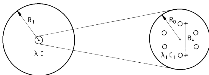
Figur 7.2.15 Trippelt U-rör i värmedrän eller trippel U-format innerslang i borrhål.
