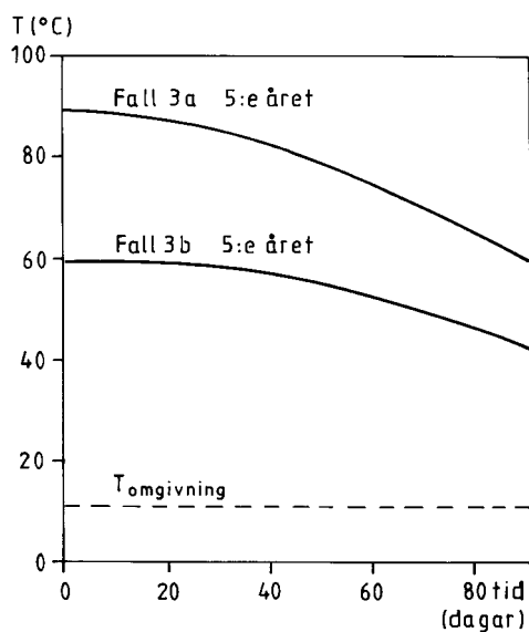
Figur 8.7.9-10. Uttagstemperatur för Alnarpsdalen, fall 2 vänster bild, och för Visingsöakviferen, fall 3 höger bild.
