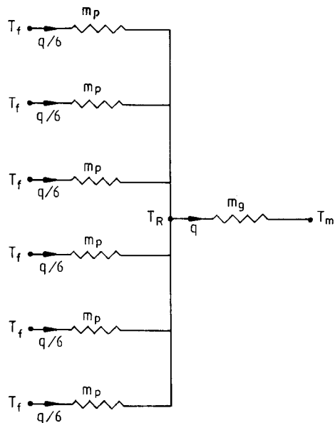
Figur 7.2.8 Värmeströmningskrets för markvärmewäxlare med sex symmetriska värmewäxlarkanalerna.
