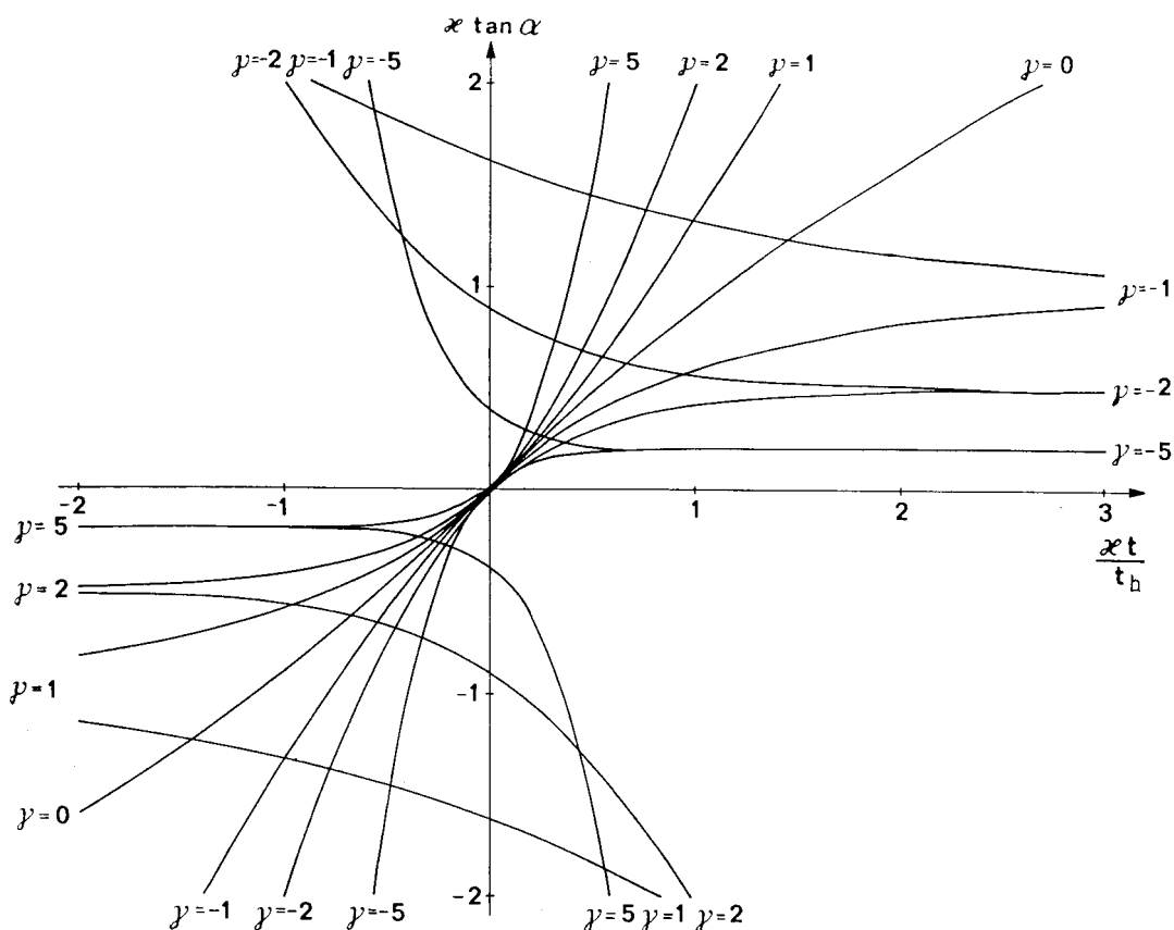
Figur 8.5.4 Samband mellan kantringsvinkeln \alpha och tiden t . Kurvorna hänförs till olika pumpflöden, vilka representeras av injektionsparametern \gamma (8.5.7), (8.5.9).
