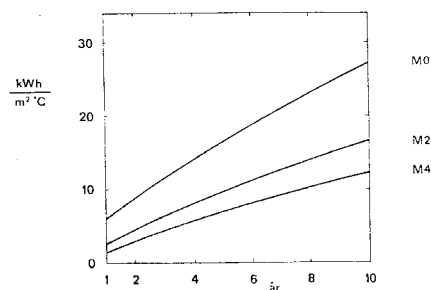
Figur 6.3.6.2 Ackumulerade värmeförluster för det större, cylindriska bergrummet.
