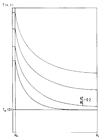
Figur 7.2.2 Temperaturfält vid konstant effektavgivning från rör till omgivande cylinderregion.
