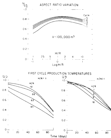
Figur 8.3.7 Variation av lagerregionens form H/R . Data enligt referensfallet (8.3.6) fränsett V_w och H .
