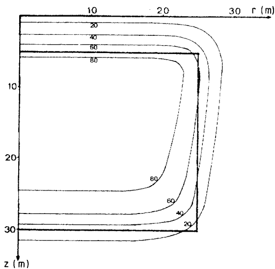
Figur 8.4.2 Temperaturfördelningen ( ^{\circ}\text{C} ) i magasin och omgivande mark efter 4 månader (3 månaders injektion och 1 månads lagring) under den första årscykeln.
