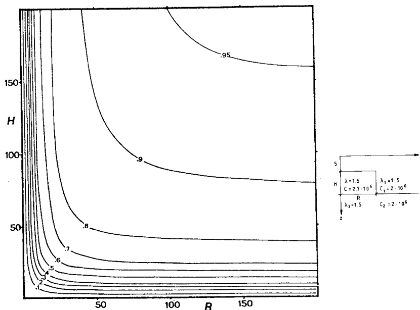
Figur 8.4.15 Energiverkningsgraden \eta_E för den femte årscykeln som funktion av magasinets höjd H (m) och radie R (m). Övriga data enligt referensfallet.
