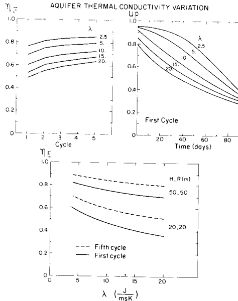
Figur 8.3.8 Variation av effektiv värmeledningsförmåga \lambda i akviferen. Data enligt (8.3.6) fränsett \lambda (övre figurerna) och \lambda , H , V_w (undre figuren).
