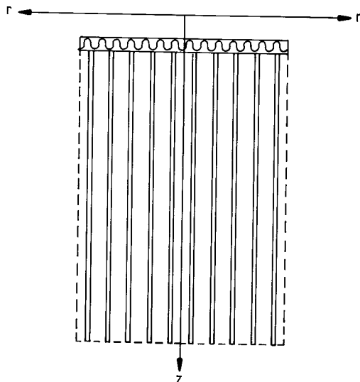
Figur 7.6.1. Skiss över markvärmelagret i Stora Skuggan.
