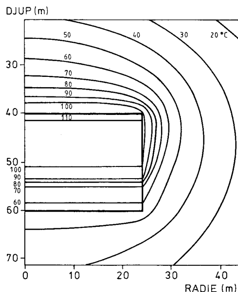
Figur 6.4.3.1 Isothermer efter tre månaders laddning är tio.
