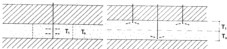
Figur 8.5.1 Akvifervärmelager med vertikal temperaturfront (t.v.) och med horisontell temperaturfront (t.h.).
