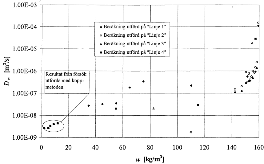
Figur 4.3. Resultat från beräkningar av transportkoefficienten D_w [ m^2/s ] utförda på Linje 1-4, se Figur 4.2. Resultaten för w < 20 \text{ kg/m}^3 är ej medtagna utan ersatta av resultat från koppförsök [8].
