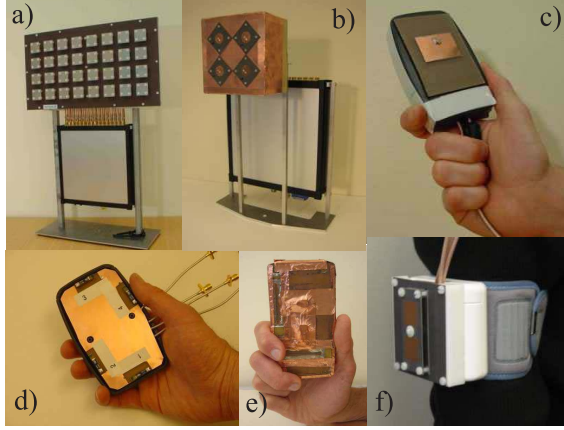
Fig. 1. The antenna devices used in the different scenarios: a) AP 2.6 GHz (middle rows used), b) AP 5.2 GHz, c) HH (Tx) 2.6 GHz, d) HH (Rx) 2.6 GHz, e) HH (Tx and Rx) 5.2 GHz, f) BW 5.2 GHz.
