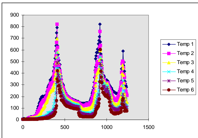
Figur 9.11, Temperatursvariation i rummet; data hämtade från ett termoelementträd som står nära initialbranden. Temp1 sitter 30 cm från taket, Temp2 sitter 60 cm från taket o.s.v.
