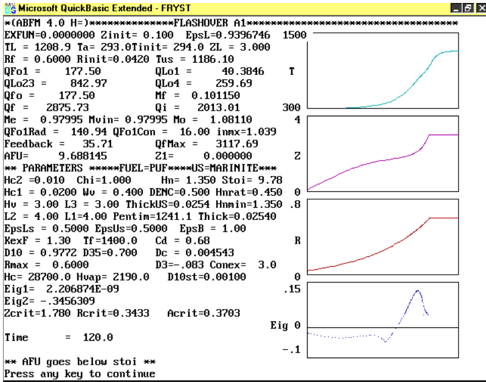
Figur E.2, Skärmbild från resultatet av en simulering med Flashover A1. Till höger syns diagram över de tre kritiska faktorerna ( T ; temperatur i brandgaslagret, Z ; brandgaslagrets tjocklek, R ; brandens radie) och under dessa ett diagram för det s.k. egenvärdet ( Eig ). I det aktuella fallet skulle övertändning alltså ske efter ca 80 s när Eig går från negativt till positivt värde (hela diagrammet motsvarar 120 s)/E.1/.
