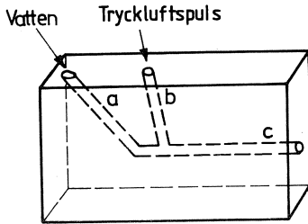
FIG. VII:11. Slagregnsmunstycke.
