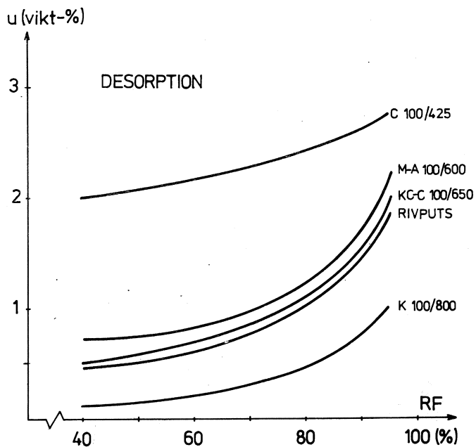
FIG. III:23. Olika putsers hygroskopiska jämviktsfuktkurvor.
