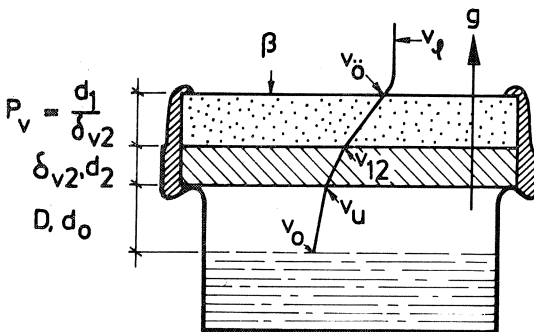
FIG. IV:10. Beteckningar vid mätning av ånggenomsläpplighetskoefficient hos puts på ett underlag.
