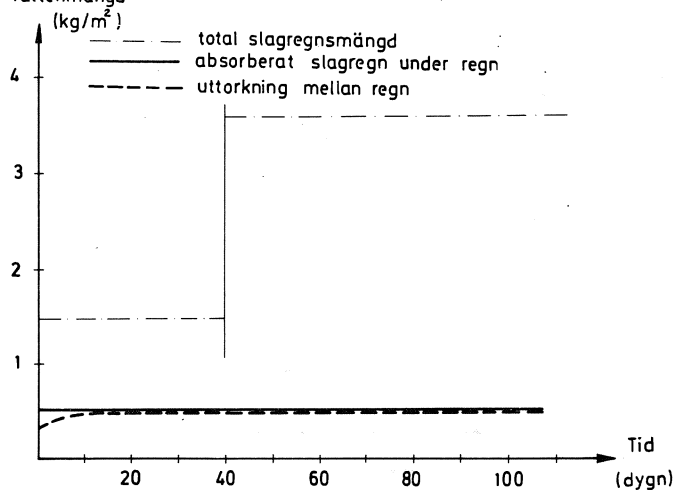
FIG. VII:57. Fuktförhållande vid cykliskt slagregn. M-A 100/600 på tegel. Moisture conditions at cyclic driving rain. Clay brick with M-A 100/600 rendering.
