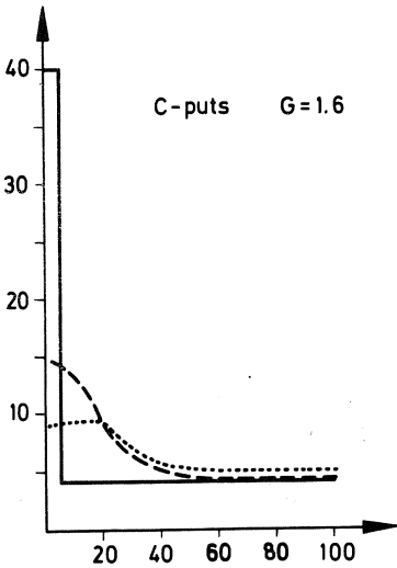
FIG. VII:39. Fuktkvotprofil under försök 1-2.
