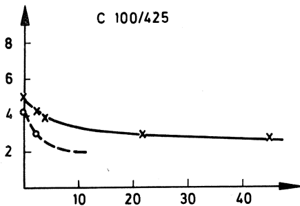
FIG. VII:34. Fuktkvot i putsen som funktion av tiden under uttorkning efter slagregn med intensiteten 0.45 \text{ kg/m}^2 \cdot \text{h} och varaktighet 3 \frac{1}{4} \text{ h} .
