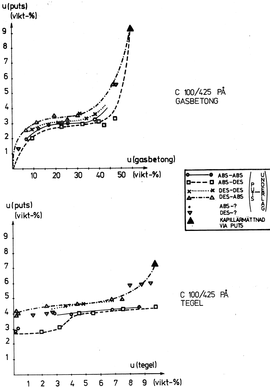
FIG. III:21. Relativa kapillära jämviktsfuktkurvor för C 100/425 på gasbetong respektive tegel.
