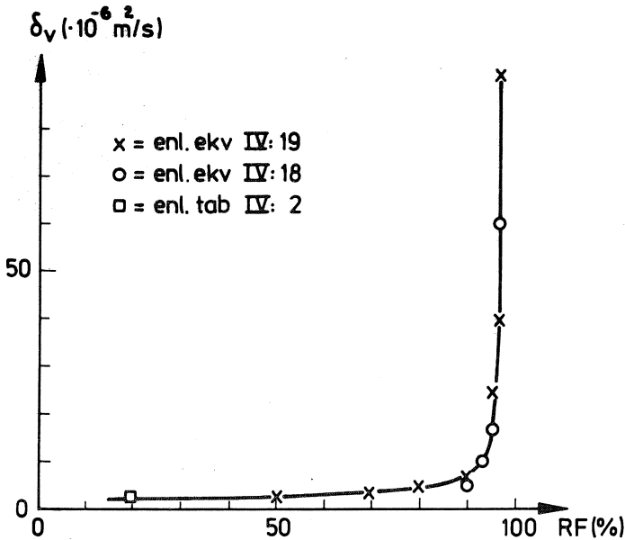
FIG. IV:9. Beräknat samband mellan ånggenomsläpplighetskoefficient i gasbetong och relativ luftfuktighet.
