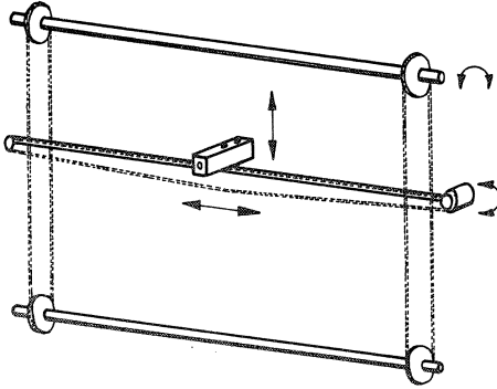
FIG. VII:13. Slagregnsapparatens rörliga delar. Movable parts of driving rain machine.
