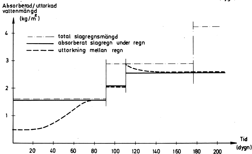
FIG. VII:47. Fuktförhållande vid cykliskt slagregn. K 100/800 på gasbetong.
