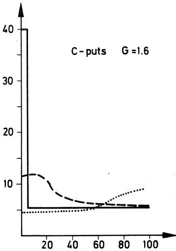
FIG. VII:40. Fuktkprofil under försök 3 — omedelbart efter regnet --- 19 h efter regnets slut ..... 5 dygn efter regnets slut
