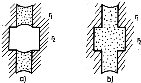
FIG. III:4. Illustration av fukttinnehåll vid fuktpotentialen p_1 med från början torrt (a) respektive fyllt (b) porsystem. Moisture content at moisture potential p_1 at absorption (a) and at desorption (b).
