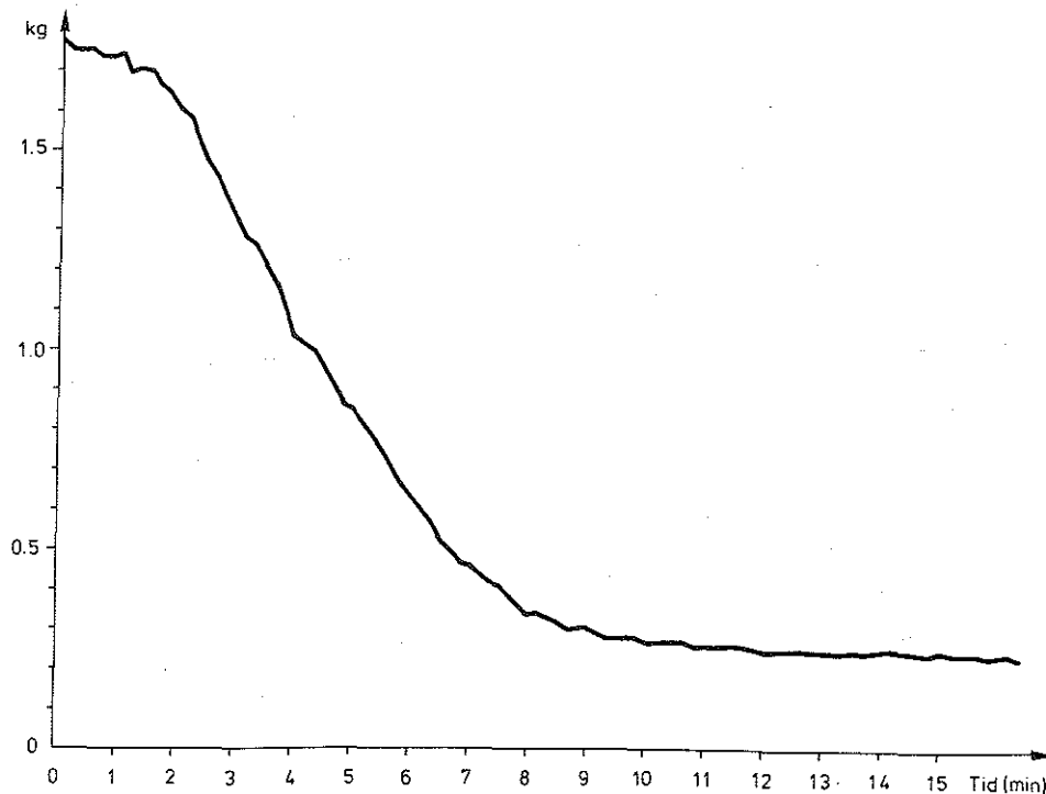
Figur 8. Viktminskningskurva för försök 46. (För material se tabell A1)
