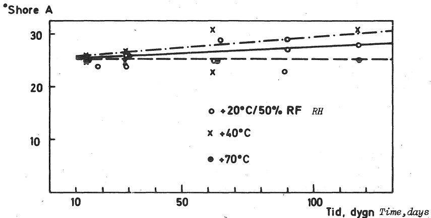
FIG 21 Härdhet i Shore A för "Material 1" som funktion av lagringstid i olika temperaturer. Initiallagring: 7 dygn i +20°C/50% RF.
