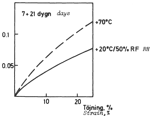
FIG 27 Arbetskurvor för "Material 3" efter värmelagring i olika klimat. Deformationshastighet: 0.001 mm/min. Provingstemperatur: +20°C.
