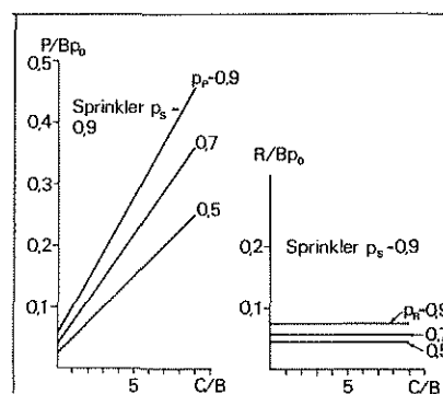
Fig 25. Maximalt tillåten kostnad för sektionering P och brandmotstånd R för att kostnaden inte skall överstiga förväntad skadereduktion som en följd av resp åtgärd, när sprinkler med en funktions-sannolikhet p_s=0,9 är installerade [36]
