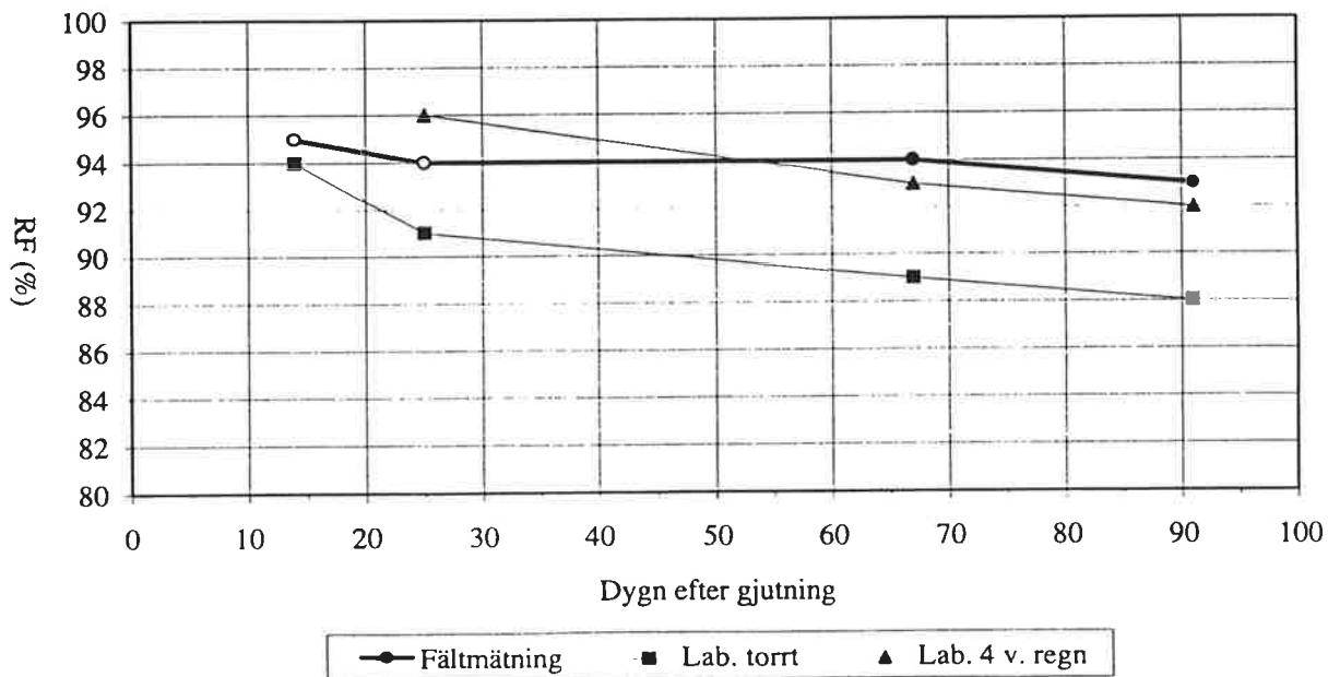
Studie 4 - Uttorkningsförlopp för betong med vct 0,63 (lab. vct 0,60)
