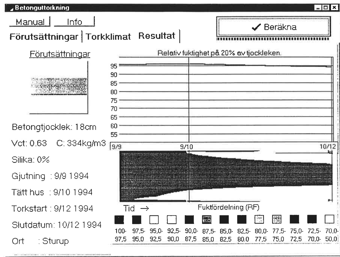
Studie 4 - Uttorkningsförlopp för betong med vct 0,63 (lab. vct 0,60)
