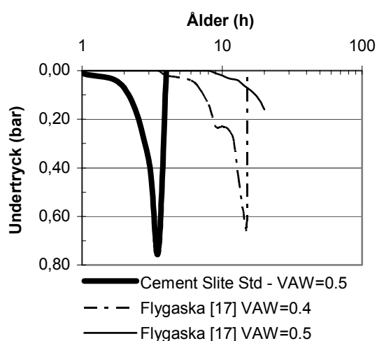
Figur 2.3 - Undertryck i blandningar med varierande volymandel vatten, VAW. Måtdjup = 40.
