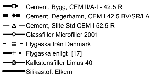
Figur 2.2 – Partikelfördelning hos cement Slite Std, Degerhamncement, flygaska och silikastoft
