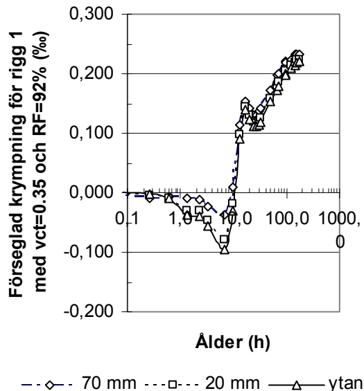
Figur 4.8 - Förseglad krympning för rigg 1 med betong med vct=0.35 och RF=92% (‰).
