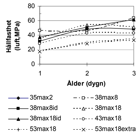
Figur 4.4 - Hållfasthet (luft,MPa).
