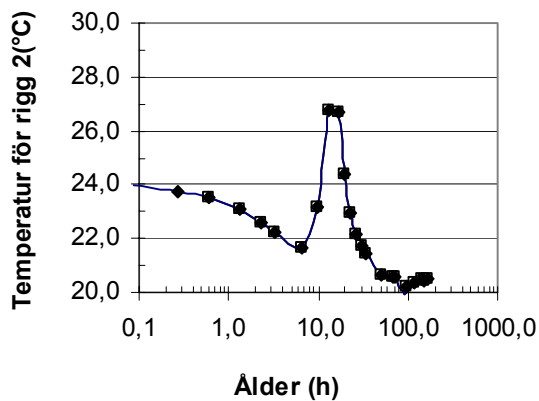
Figur 4.10 - Temperatur för rigg 2 (°C).
