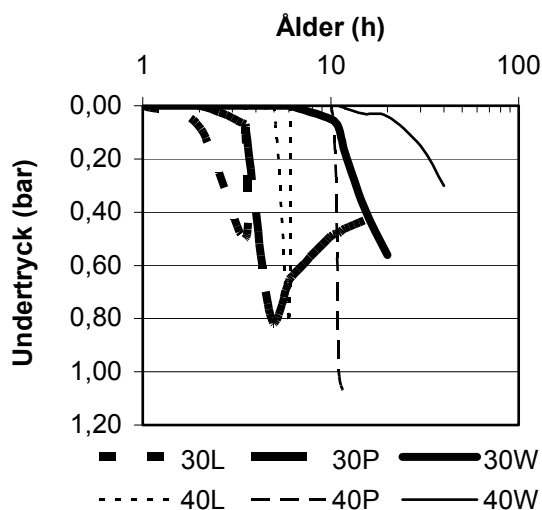
Figur 2.4 - Undertryck i blandningar med varierande vbt och härdningsbetingelser. L = luft, RF = 50%, P = paraffinolja, W = vatten. Måtdjup = 40 mm.
