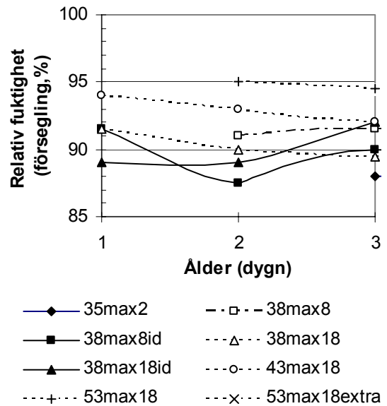
Figur 4.3 - Relativ fuktighet (försegling,%).
