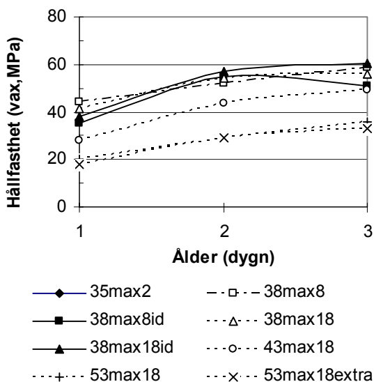
Figur 4.6 - Hållfasthet (vax,MPa).
