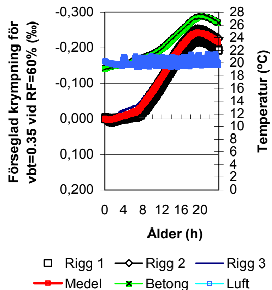
Figur 5.1 – Förseglad 1-dygnskrympning för betong 35max8 preparerad i RF = 60%. Beteckningar: 35 = vbt (%), max8 = ballast 8 mm.
