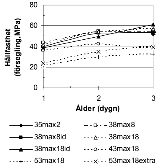
Figur 4.2 - Hållfasthet (försegling,MPa).
