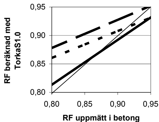
Figur 2.42 - RF enligt TorkaS1.0 versus uppmätt RF. RF enligt TorkaS1.0 (tunn linje) stämde med uppmätt RF vid självuttorkning
