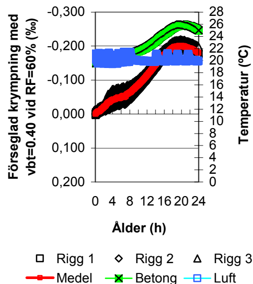
Figur 5.2 - Förseglad 1-dygnskrympning för betong 40max8 preparerad i RF = 60%. Beteckningar: 40 = vbt (%), max8 = ballast 8 mm.
