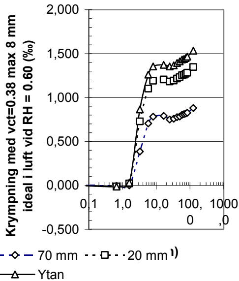
Figur 4.22 – Krympning, vct=0.38 max 8 ideal i luft vid RH = 0.60.
