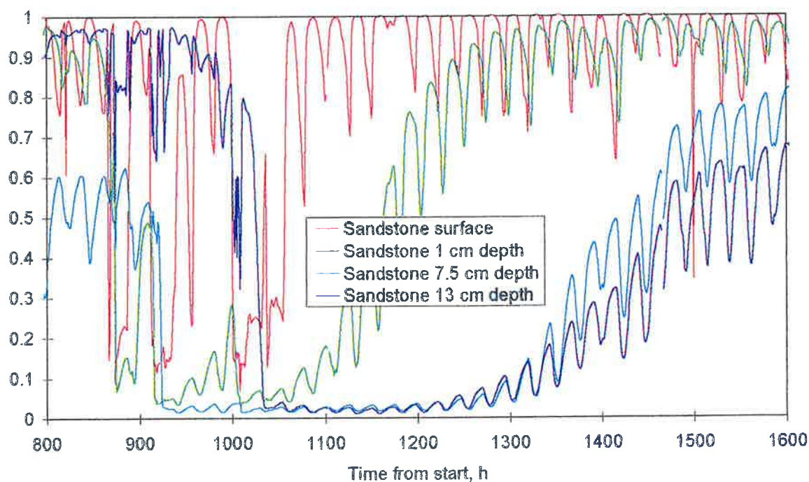
Figur B2. Givarutslag på olika avstånd från ytan som funktion av tid för sandsten, 800 - 1600 timmar efter start.
