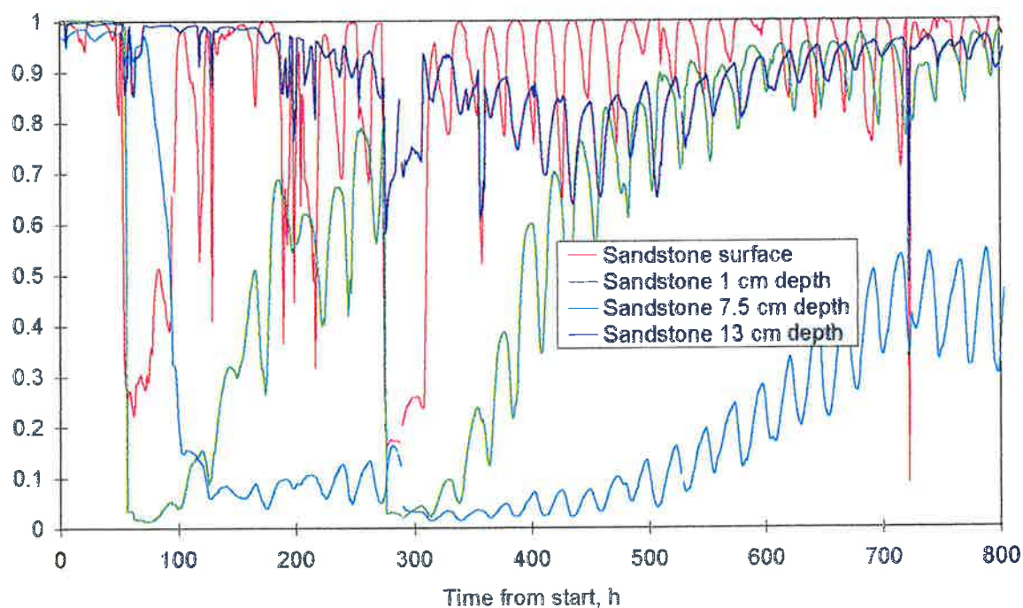
Figur B1. Givarutslag på olika avstånd från ytan som funktion av tid för sandsten, 0 - 800 timmar efter start.
