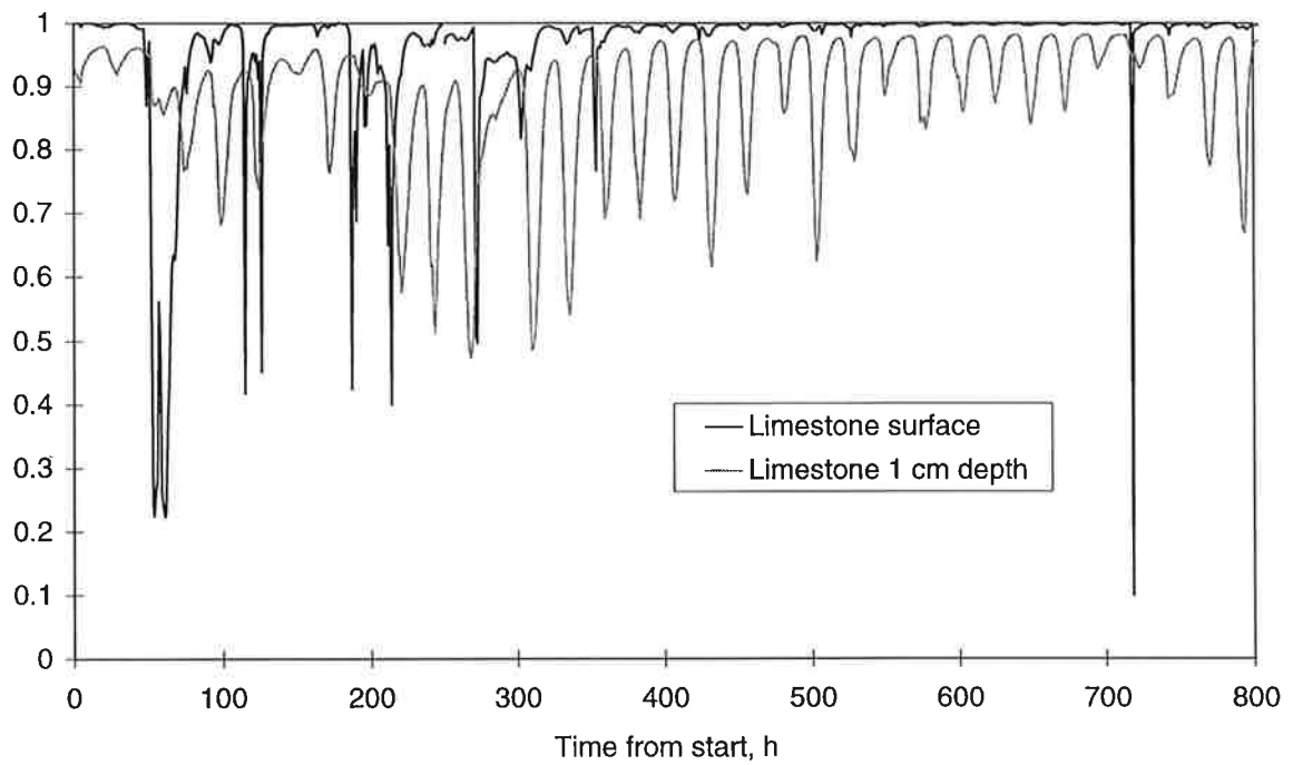
Figur B4. Givarutslag på olika avstånd från ytan som funktion av tid för kalksten, 0 - 800 timmar efter start.
