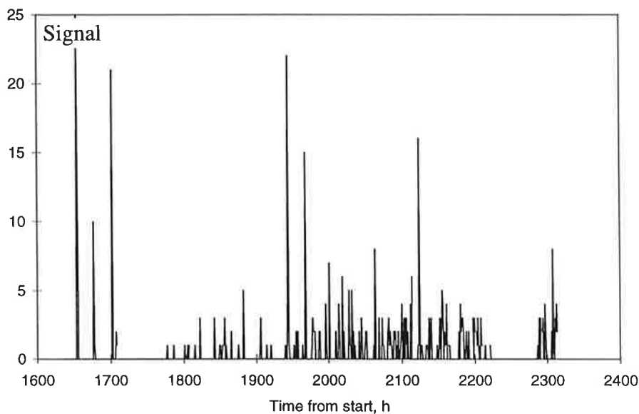
Figur 5. Resultat från slagregnmätare.
