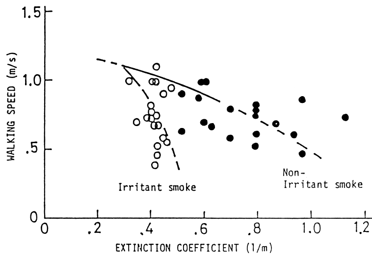
Figur 1 Förhållandet mellan gånghastighet och röktäthet enligt Jin (1978).
