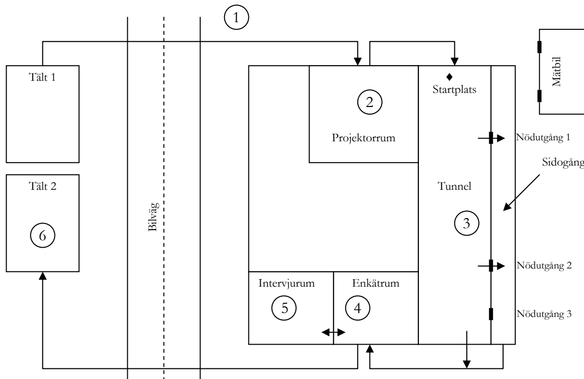
Figur 7 Försöksuppställning. Nödutgång 3 saknade förbindelse till sidogången och var endast illustrerad som utrymningssväg. Siffrorna anger försöksordningen.
