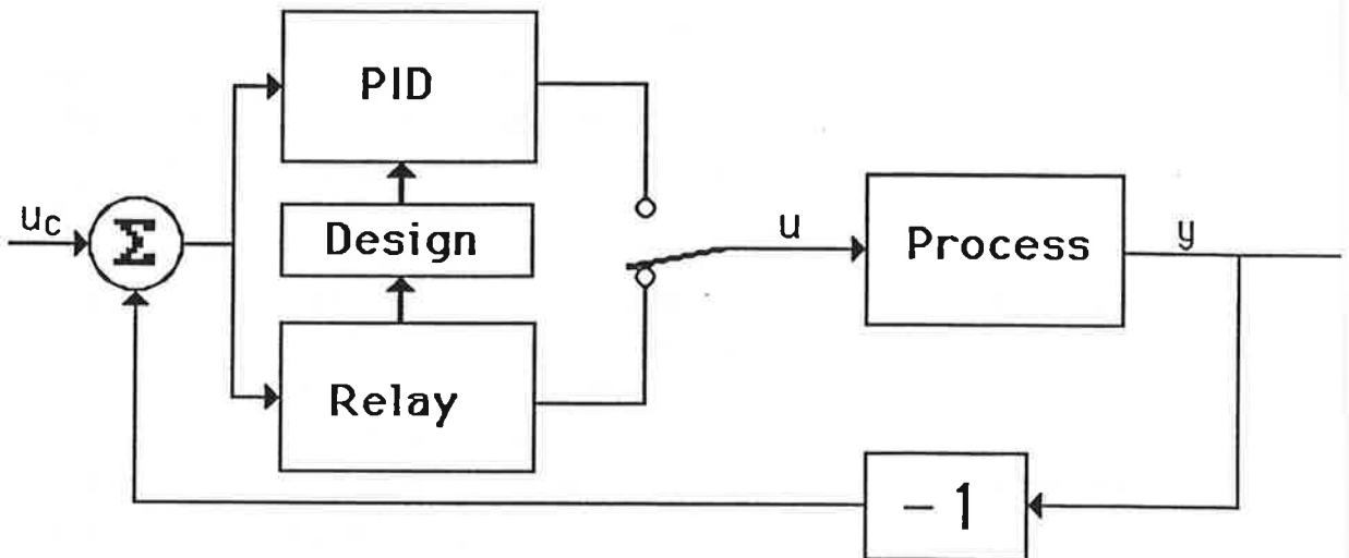
Figur 2. Blockdiagram för automatinställare med relä.
