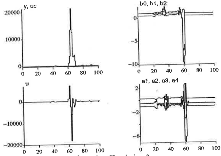
Figur 3. Simulering 3
