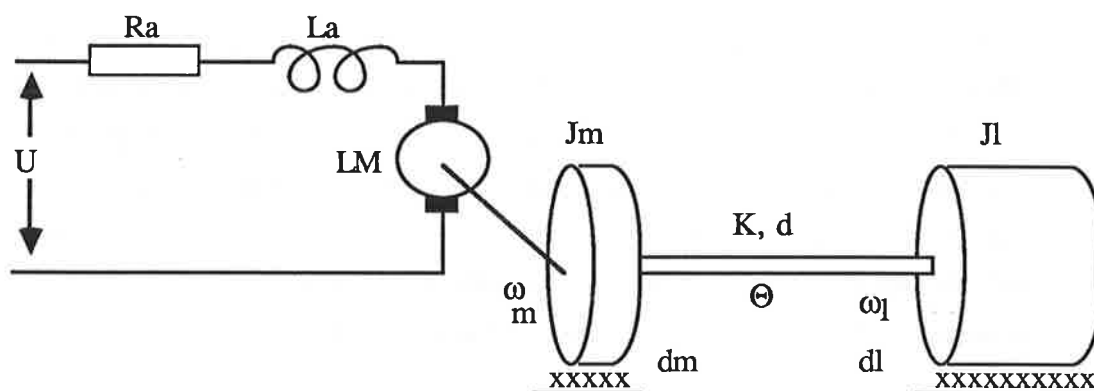
Figur 2.1 Beskrivning av en relativt noggrann modell för en likströmsmotor som är sammankopplad till en stor massa via en vev axel.
