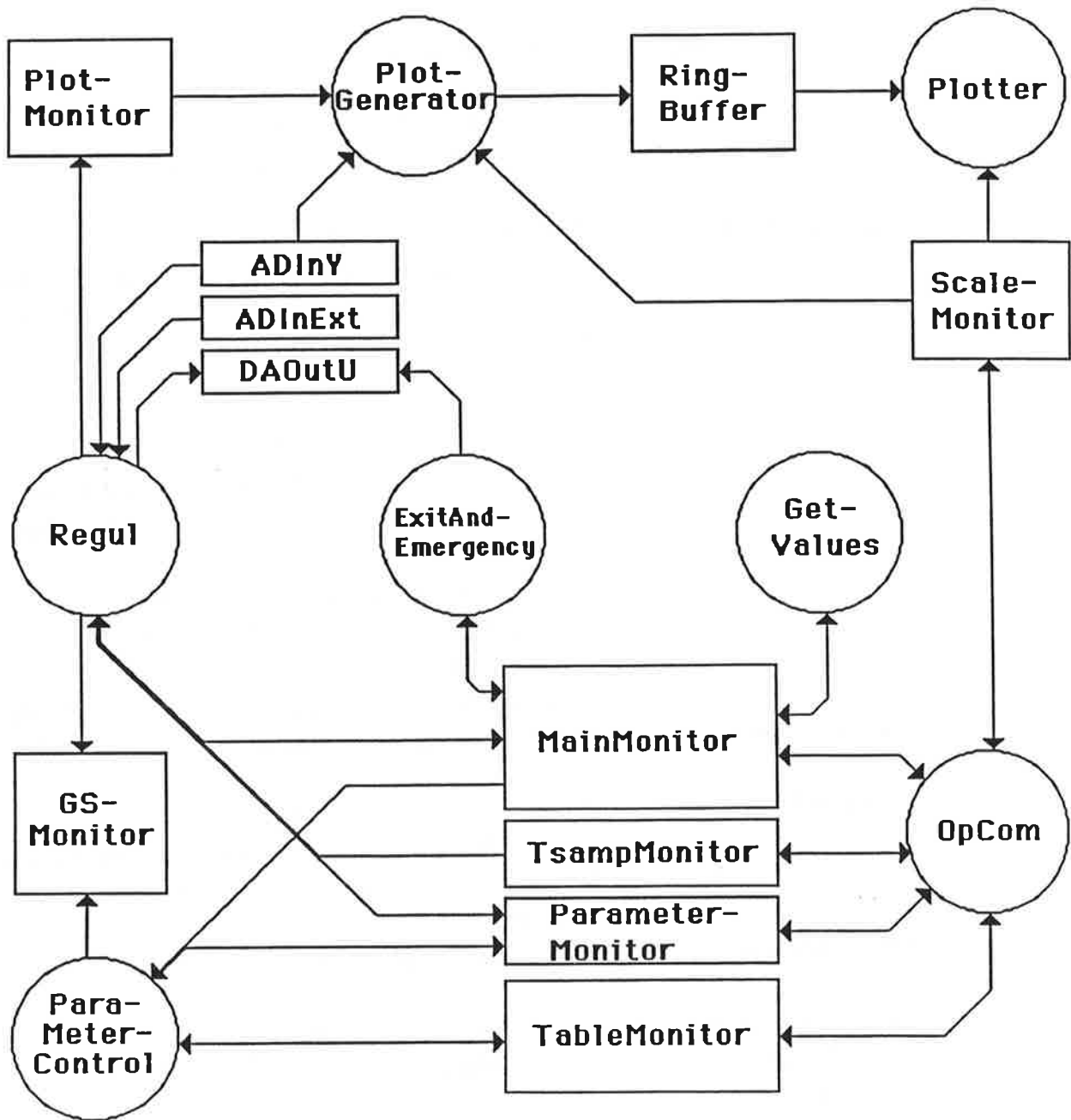
Figur 1. Processgraf.
