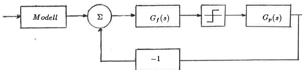
Figur 2. Grundprincip för reläsvängningsmetoden.
