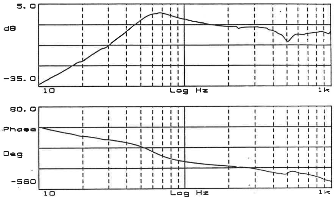
Figur 1.1 Frekvens- och faskurvor för konventionell bashögtalare.
