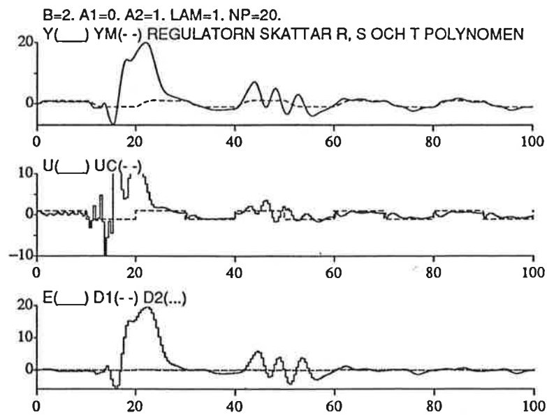
Figur 6.10 Direkt STR polerna på imaginära axeln
