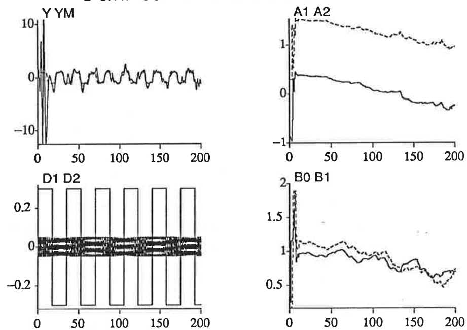
Figur 5.3 Simulering med en självinställande regulator, där en laststörning och mätbrus lagts på.
