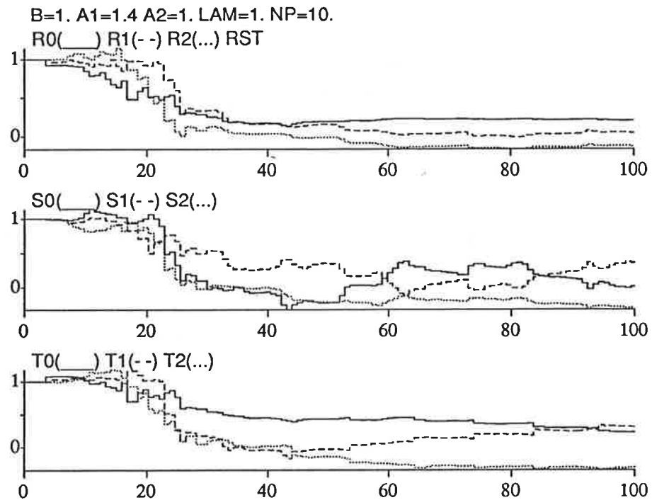
Figur 6.6 Direkt STR långsammare sampling
