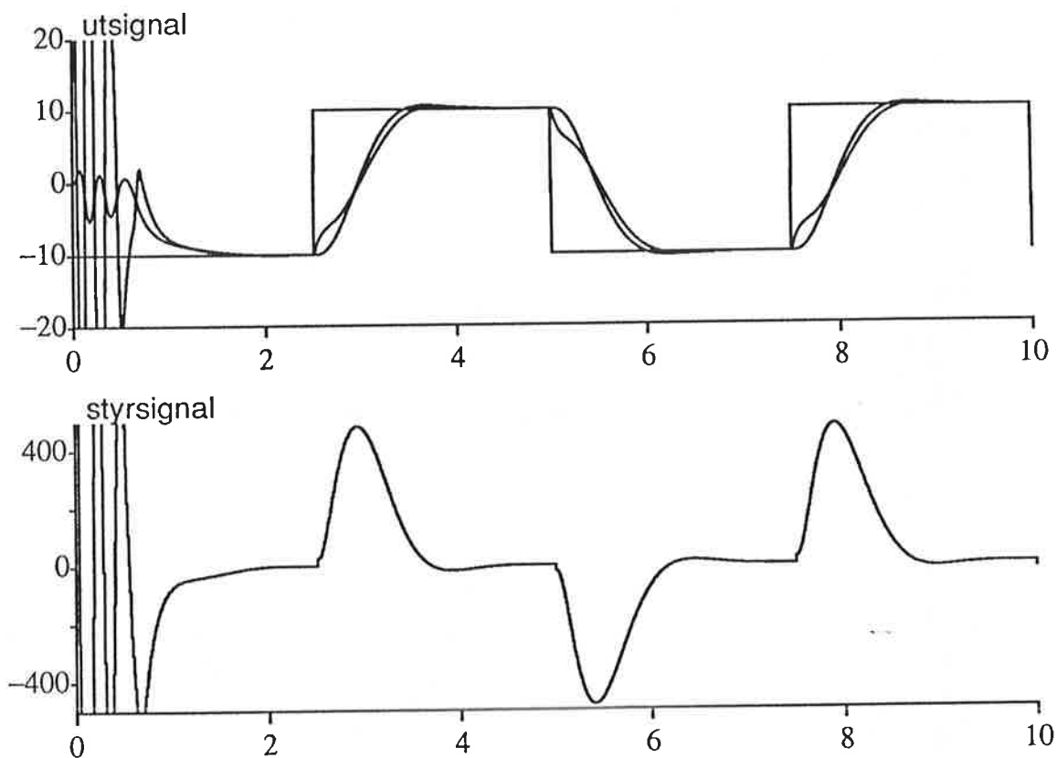
Figur 4.1 Simulering där parameterskattaren skattar tre parametrar och dämpningen i processen är noll.
