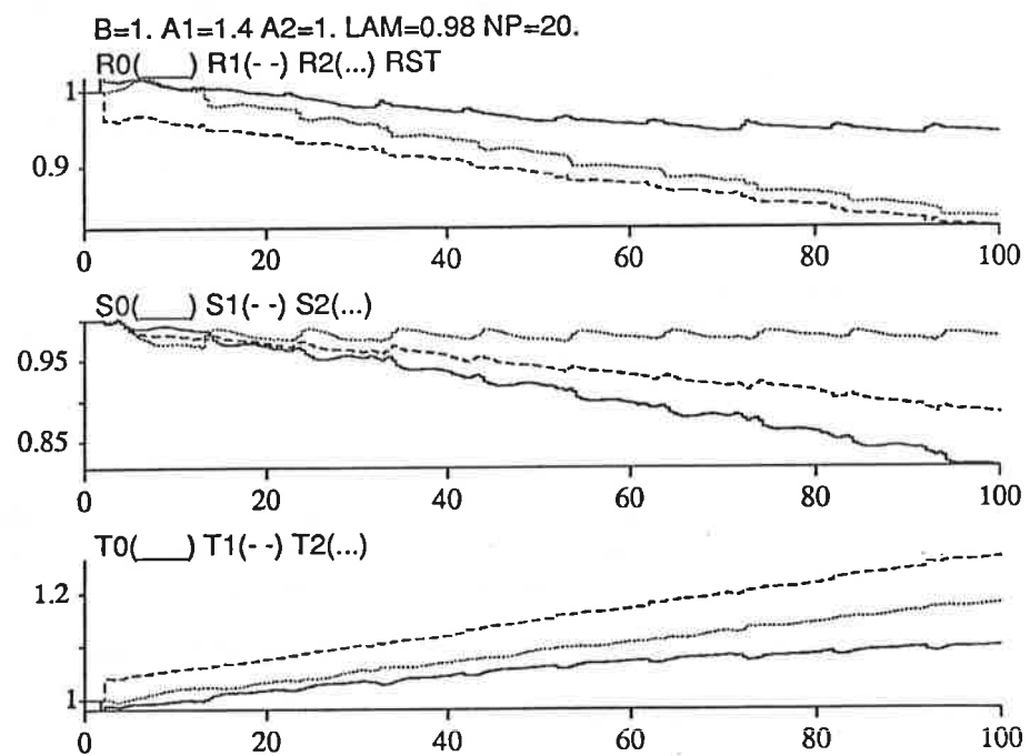
Figur 6.3 Direkt STR ,parametrarna
