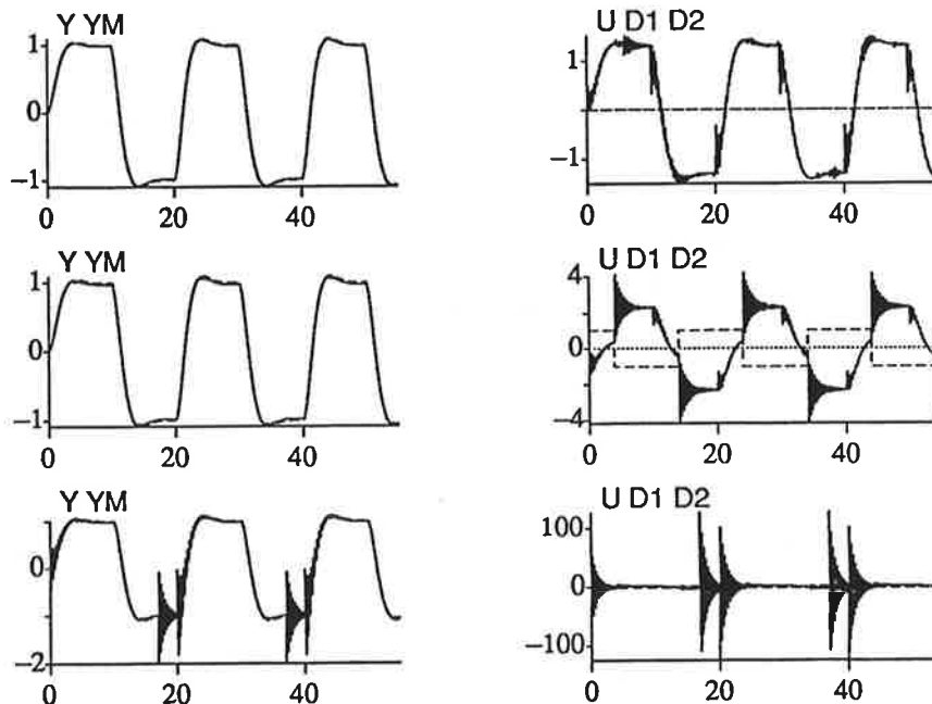
Figur 2.2 Simuleringar med High-Gain reglering. Överst utan störningar, i mitten med laststörning och nederst med både last- och mätstörningar.
