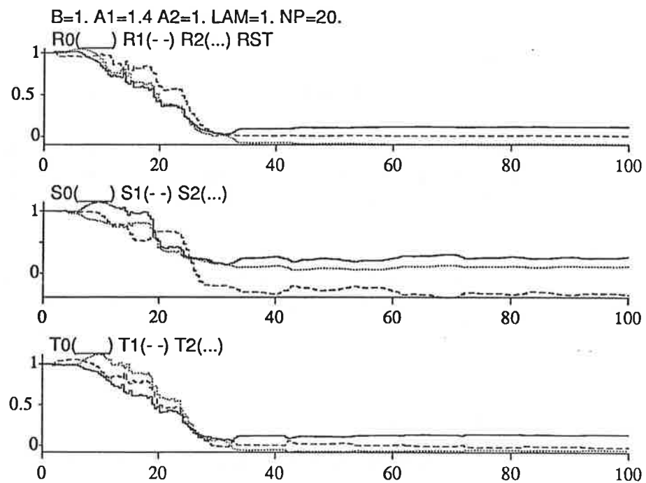
Figur 6.5 Direkt STR glömskefaktorn är ett
