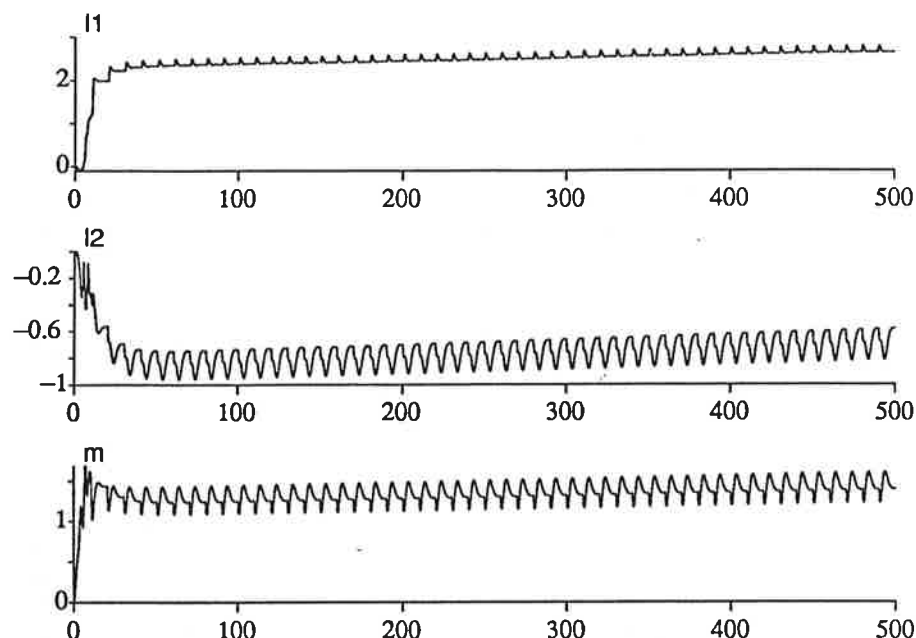
Figur 4.4 Simulering med ett modellreferenssystem med uppdatering enl. Lyapunov. x_1 rekonstrueras med en lågpassfiltrerad derivering av y .
