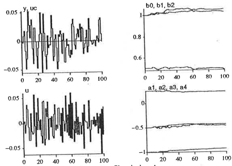
Figur 4. Simulering 4
