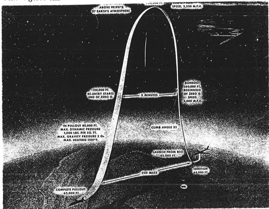
Figur 1. Exempel på en X-15 flygning.
