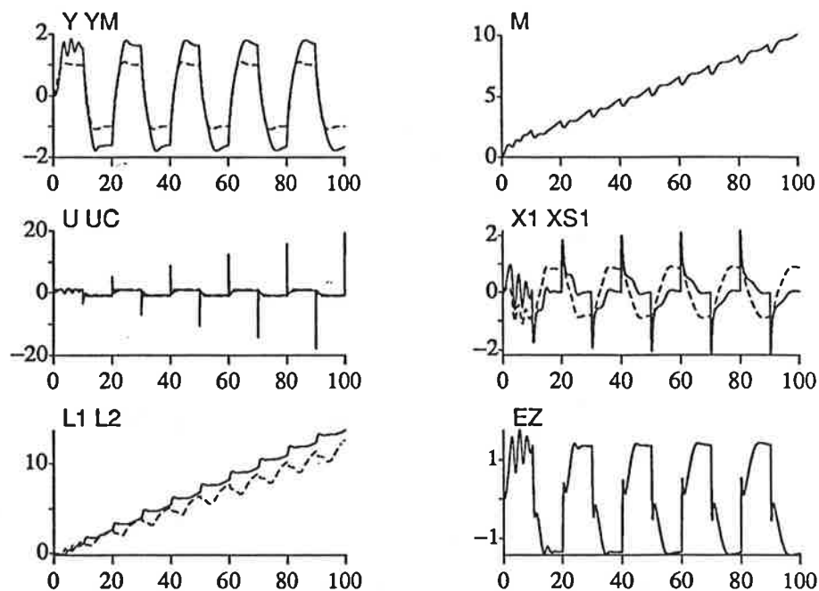
Figur 4.2 Simulering med ett modellreferenssystem med uppdatering enl. Lyapunov. x_1 rekonstrueras med en Luenberger observerare.
