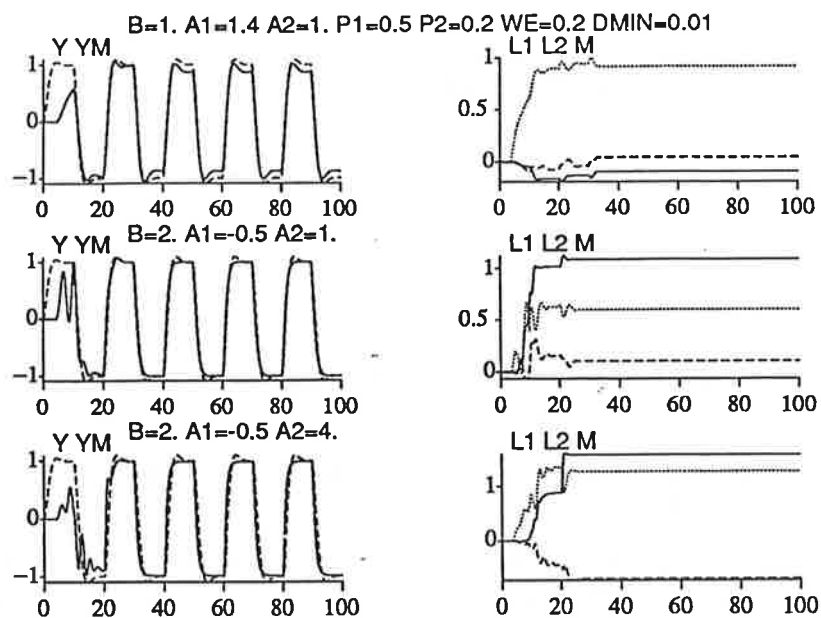
Figur 4.5 Simulering med ett modellreferenssystem med uppdatering enl. Lyapunov. På uppdateringen finns en "död-zon" d_{min} .
