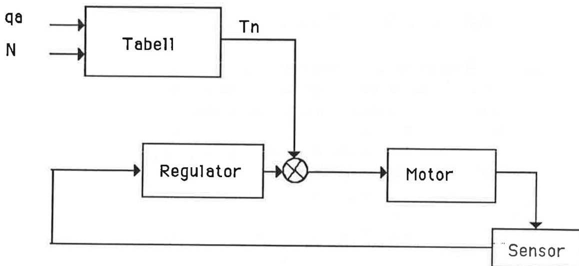
Figur 3 Reglering med lambda-sond
