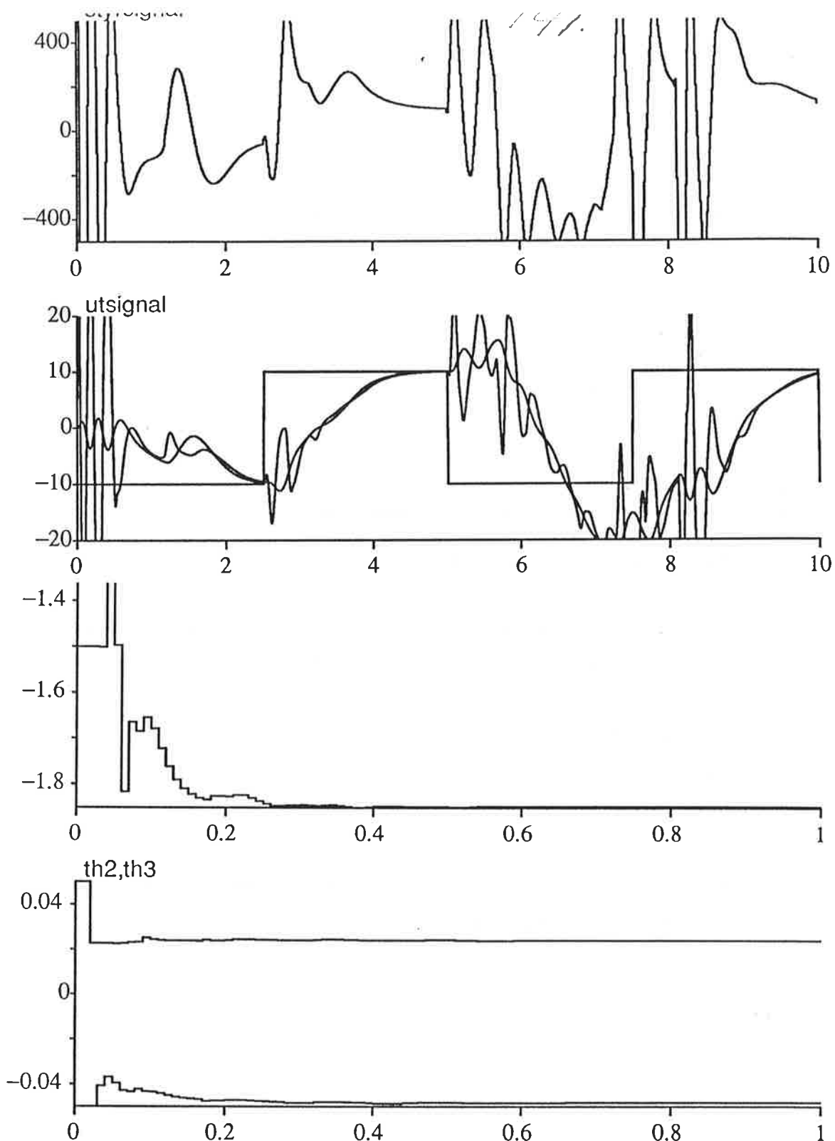
Figur 4.5 Simulering där dämpning har lagts in i processen. Regleringen blir inte längre speciellt bra.
