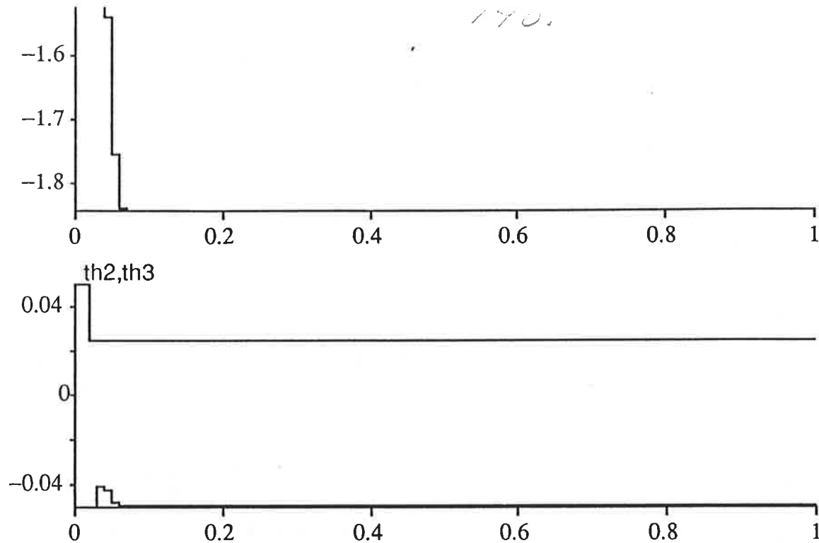
Figur 4.4 Parameterskattaren skattar fortfarande rätt.
