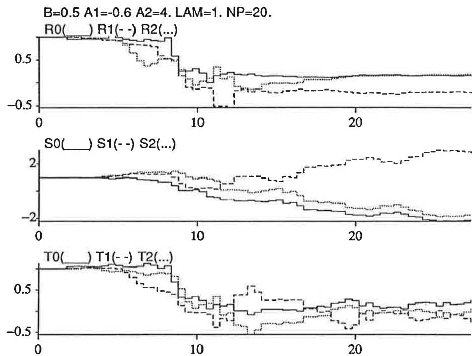
Figur 6.13 Direkt STR polerna i HHP, parametrarna
