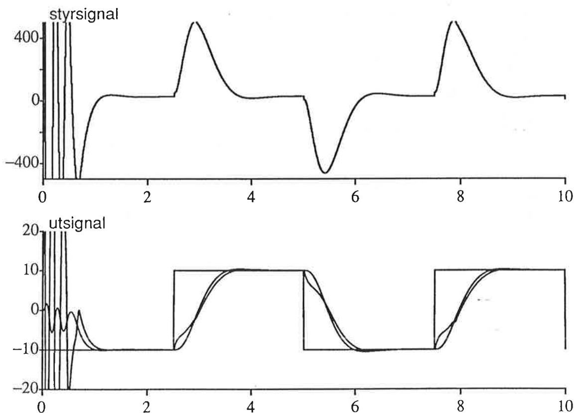
Figur 4.3 Simulering där ett motmoment har lagts på lasten. Regleringen blir utmärkt.
