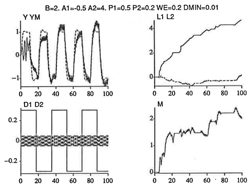
Figur 4.6 Samma simulering som nederst i fig 4.5 ovan men med en laststörning d_1 och mätbrus d_2 .
