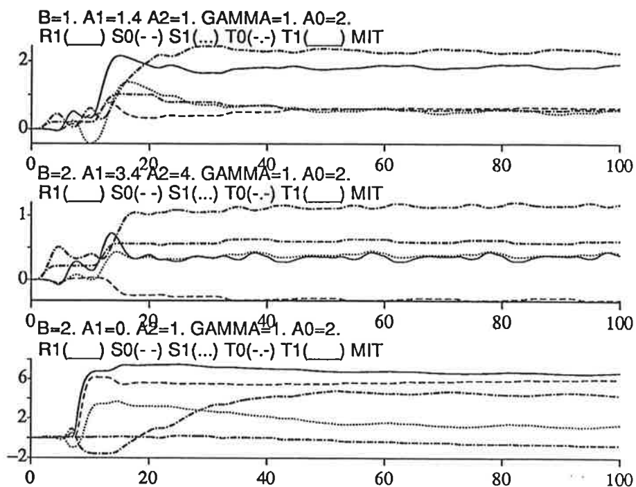
Figur 3.8 Parametrans uppförande från figur 1 till figur 3
