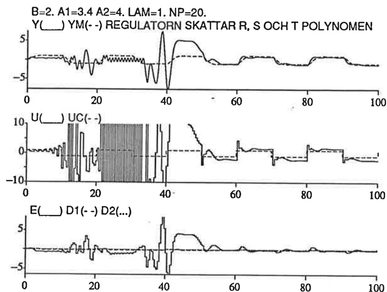
Figur 6.8 Direkt STR polerna i VHP
