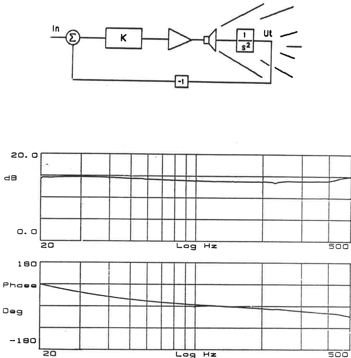
Figur 2.3 Blockschema samt amplitud- och fäsgång vid "optimal" loop förstärkning.
