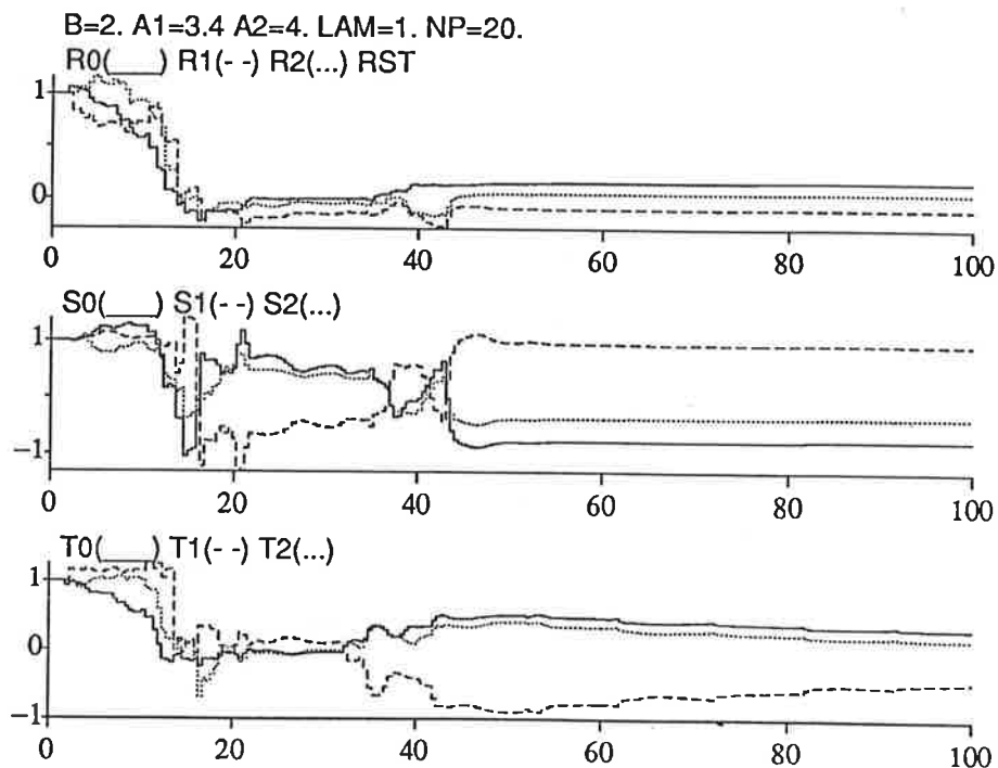
Figur 6.9 Direkt STR polerna i VHP, parametrarna
