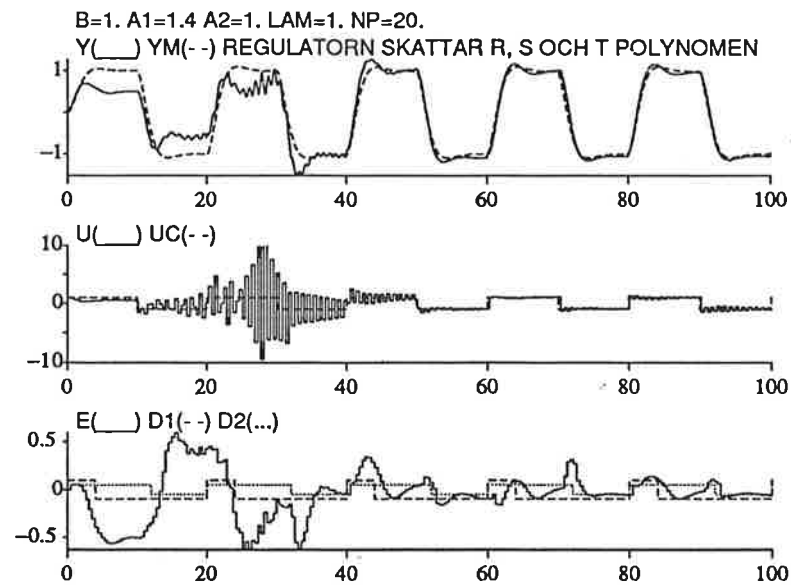
Figur 6.4 Direkt STR glömskefaktorn är ett
