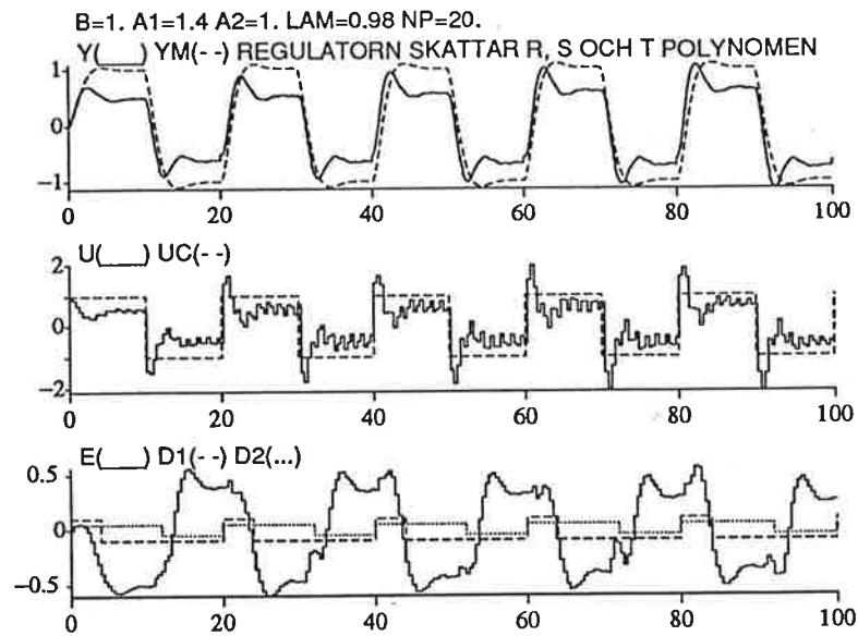
Figur 6.2 Direkt STR
