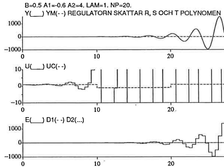
Figur 6.12 Direkt STR polerna i HHP
