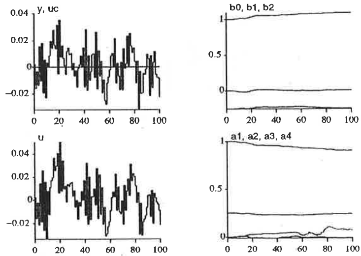
Figur 8. Simulering 8
