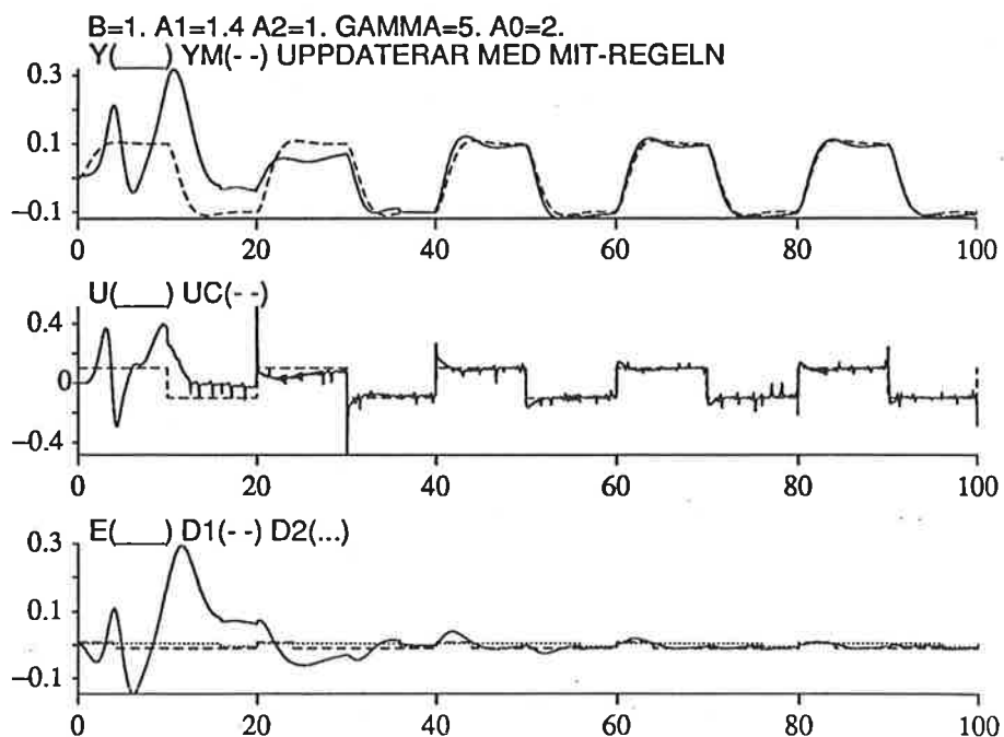
Figur 3.7 MIT-regulator gammas påverkan på systemet
