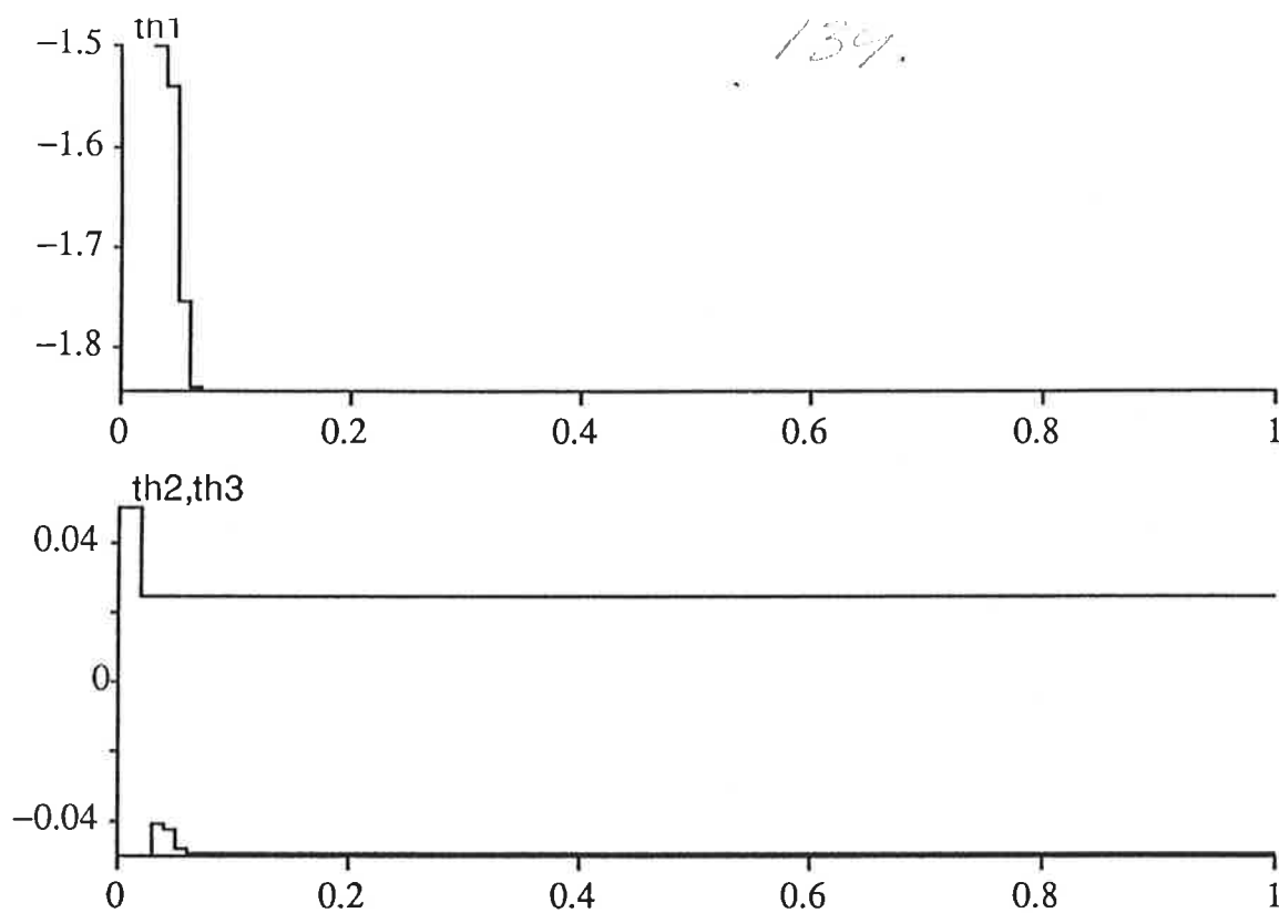
Figur 4.2 Parameterskattaren svänger in sig snabbt och utsignalen följer referensvärdet mycket bra.
