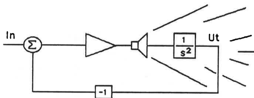
Figur 2.1 Blockschema för Philips MFB-högtalare.
