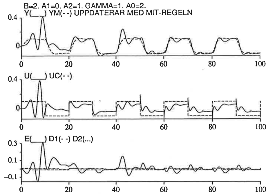
Figur 3.4 MIT-regulator polerna på imaginära axeln
