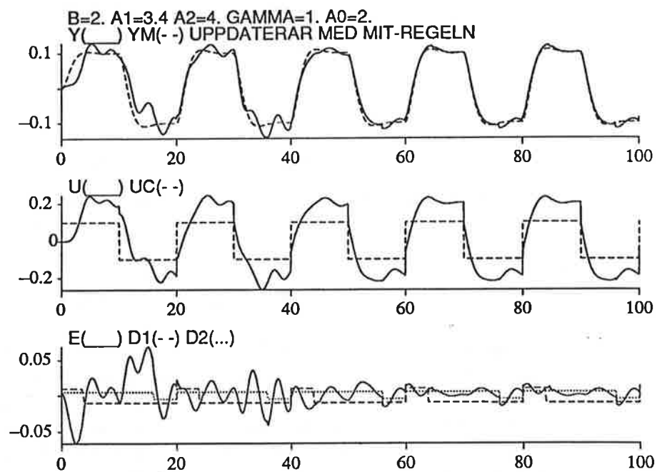
Figur 3.3 MIT-regulator polerna i VHP
