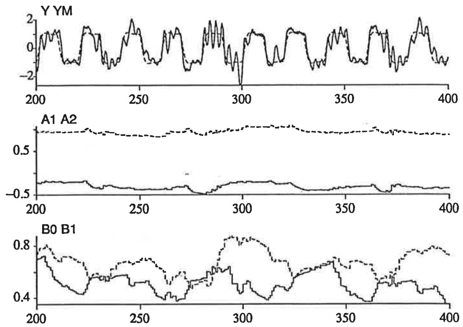
Figur 5.4 Fortsättning på simuleringen i fig 5.3
