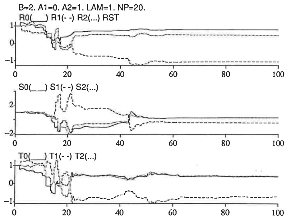
Figur 6.11 Direkt STR polerna på imaginära axeln, parametrarna
