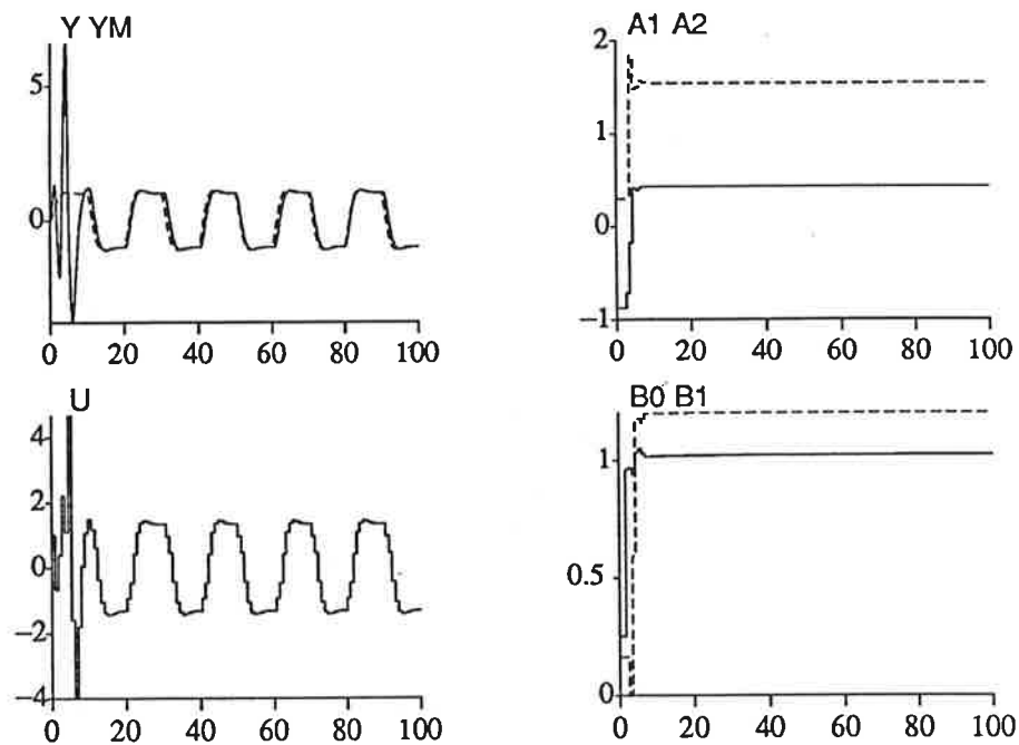
Figur 5.2 Simulering med en självinställande regulator.
