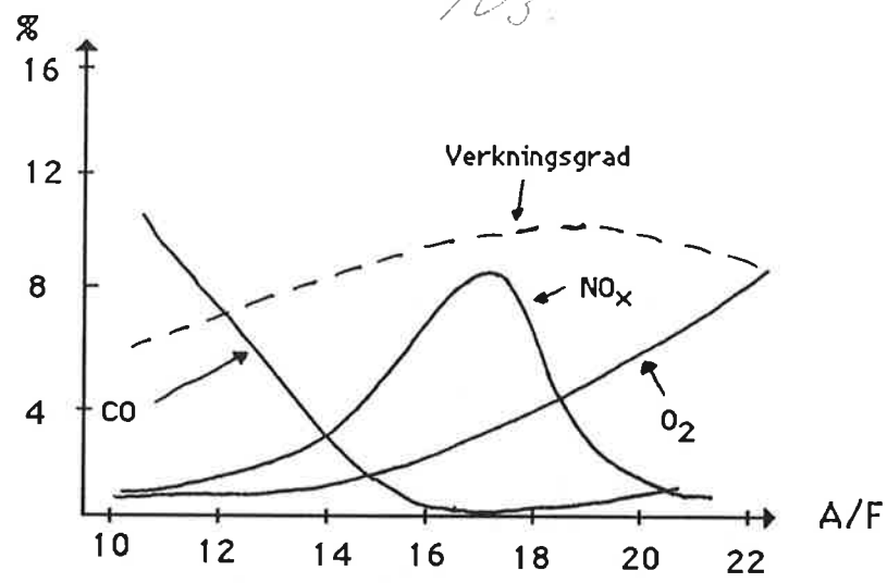
Figur 1 Avgasernas beroende av A/F
