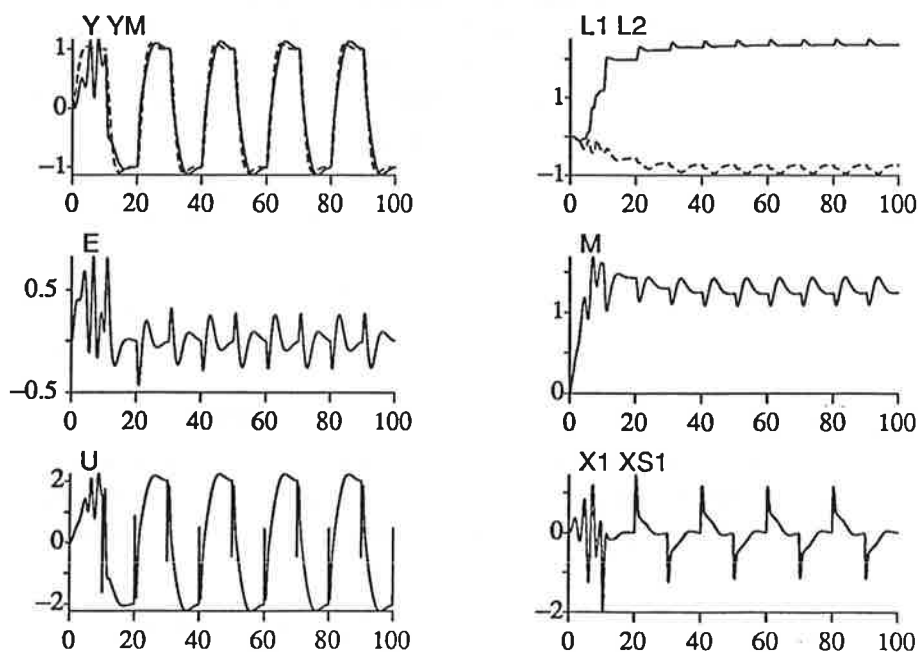
Figur 4.3 Simulering med ett modellreferenssystem med uppdatering enl. Lyapunov. x_1 rekonstrueras med en lågpasfiltrerad derivering av y .
