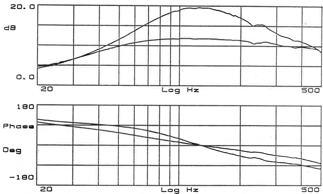
Diagram 2.2 Amplitud- och faszång open / closed loop.
