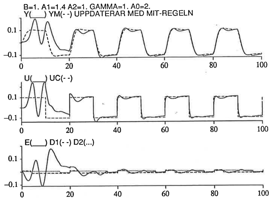
Figur 3.2 MIT-regulator processen är lika med modellen
