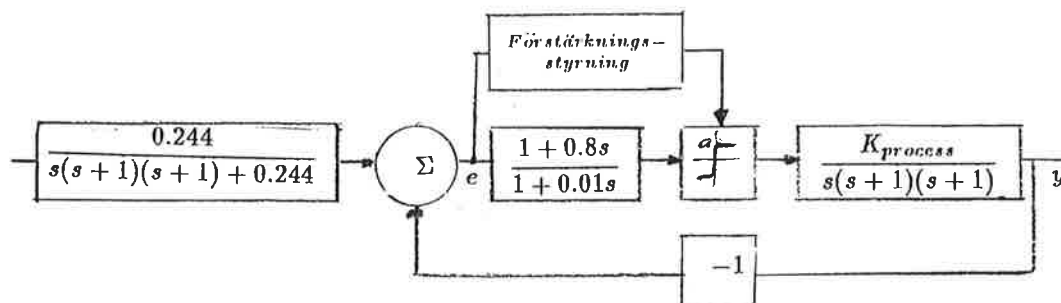
Figur 3. Förenklad modell med variabel reläamplitud.
