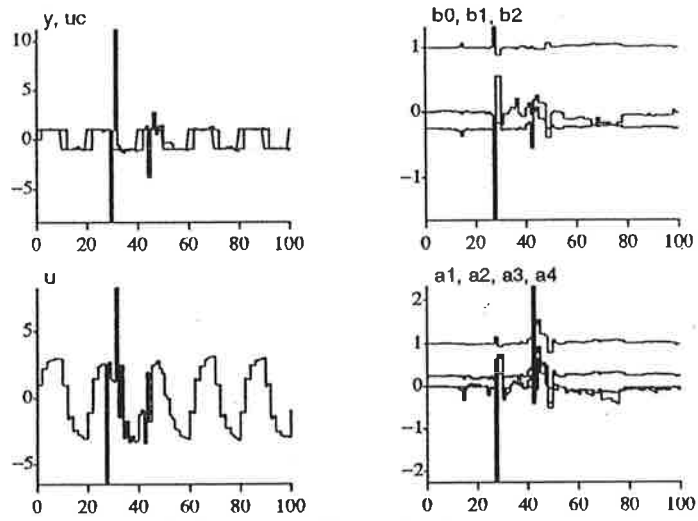
Figur 7. Simulering 7
