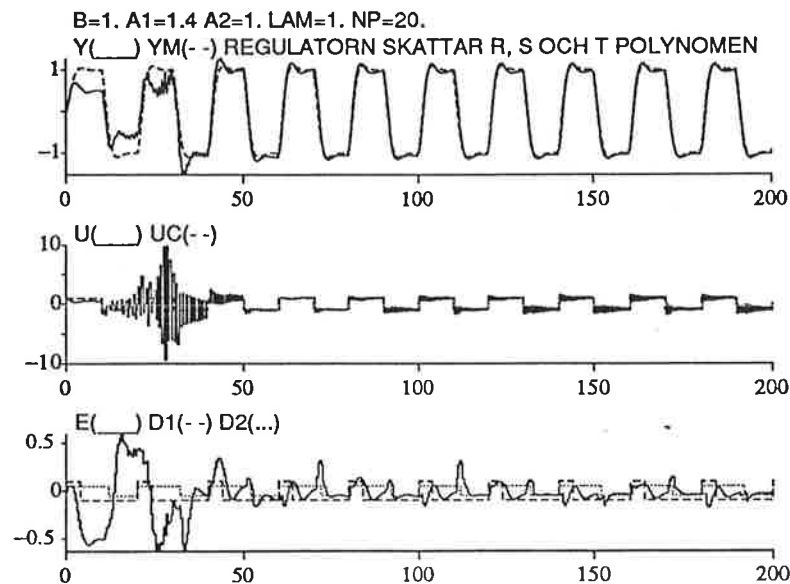
Figur 6.7 Direkt STR ringningar i styrsignalen
