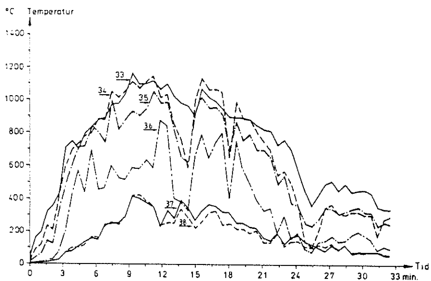
Figur 6.4.1 Temperaturfördelning som funktion av tiden i fönsteröppningen vid brandbelastning av typ A, försök 1. Numrering över fönsterhöjden uppifrån och ner
