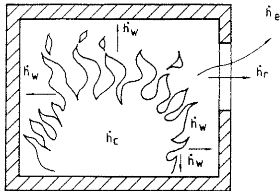
Figur 6.2.1 Den fullt utvecklade rumsbrandens energibalans
