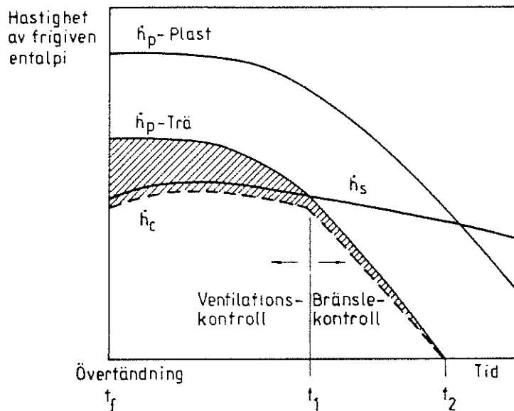
Figur 6.2.2 Möjliga tidkurvor för hastigheten av frigiven entalpi vid en fullt utvecklad rumsbrand med två olika bränsletyper - trä och plastmaterial [18]
