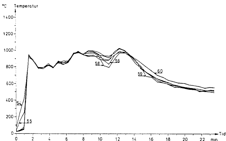
Figur 6.3.3 Tidsvariationen av temperaturfördelningen längs en vertikal genom brandcellens centrum vid försök 2. Brandbelastning typ B. Testfönster med karm och båge av PVC. Termoelementens placering framgår av fig 5.4.2
