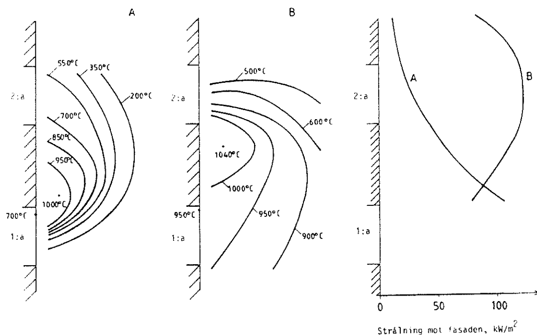
Figur 1.1 Den externa flammans längd och form och tillhörande termisk fasadpåverkan, karakteriserad av isotermerna och fördelningen av strålning mot fasaden vid tiden för maximal temperatur närmast fasaden
