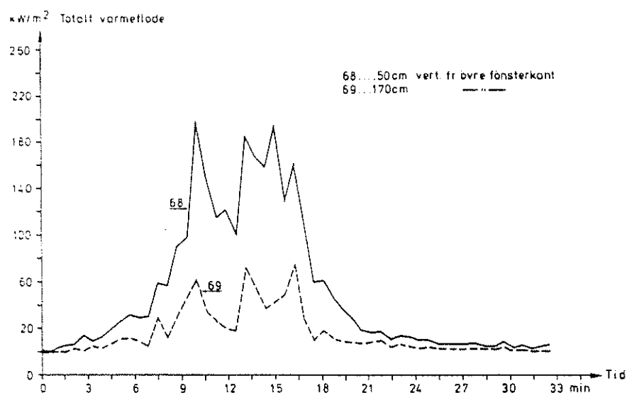
Figur 6.6.1 Tidsvariationen av totalt värmefflöde mot fasaden på höjdnivåerna 50 cm och 170 cm ovanför överkanten av brandrummets fönsteröppning. Brandbelastning av typ A, försök 1
