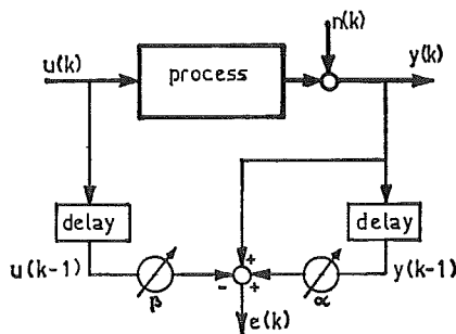
FIG. 5. Parameter estimation using a generalized model.
