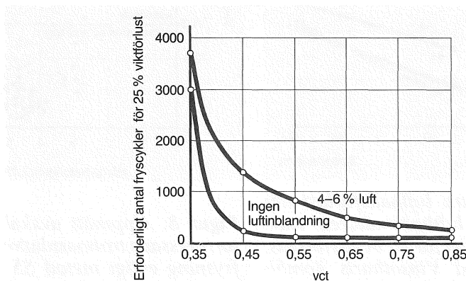
Figur 6. Samband mellan frostbeständighet och vattencementtal, US Bureau of Reclamation (1955).
