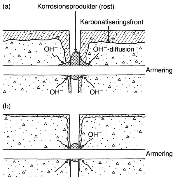
Figur 53. Korrosion i sprickor utan klorider. Återalkalisering. (a) Høgt vattencementtal (b) Lågt vattencementtal
