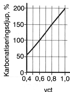
Figur 38. Vattencementtalets betydelse för relativa karbonatiseringsdjupet, Meyer et al (1967).
