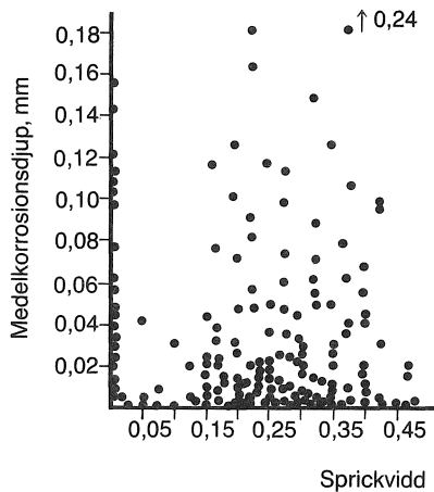
Figur 52. Uppmätta korrosionsdjup som funktion av sprickvidden efter 10 års exponering i kloridfri miljö, Schiessl (1975).
