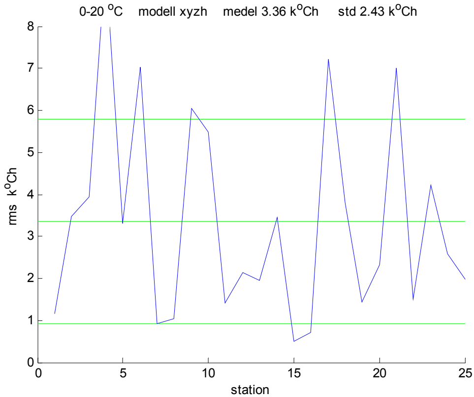
Figur 5.38 Rms i k°Ch för gränstemperatur 0-20 °C för modell (5.8) med övriga stationer.
