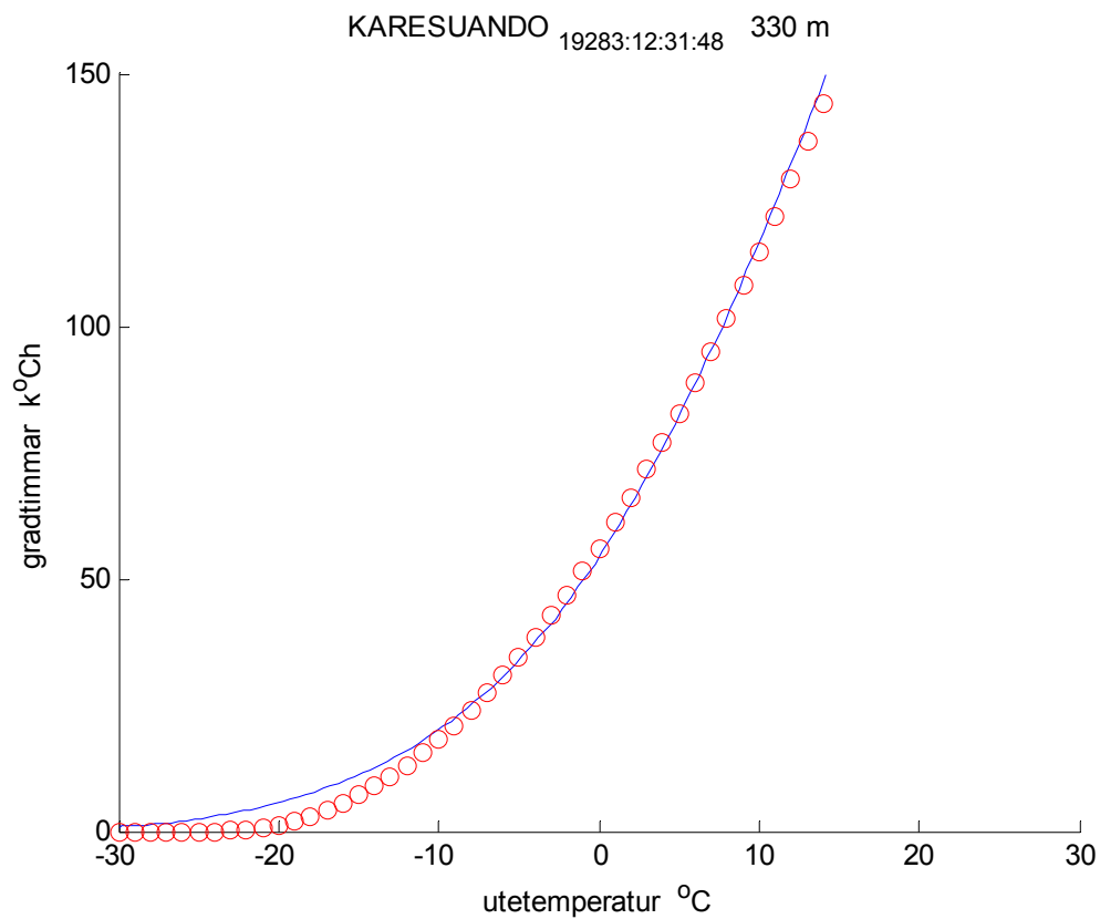
Figur 4.50 Uppmätt och förenklad gradtimmemfunktion enligt (4.1-6) för Karesuando.
