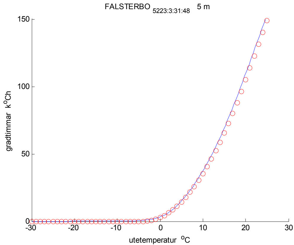
Figur 4.49 Uppmätt och förenklad gradtimmemfunktion enligt (4.1-6) för Falsterbo.
