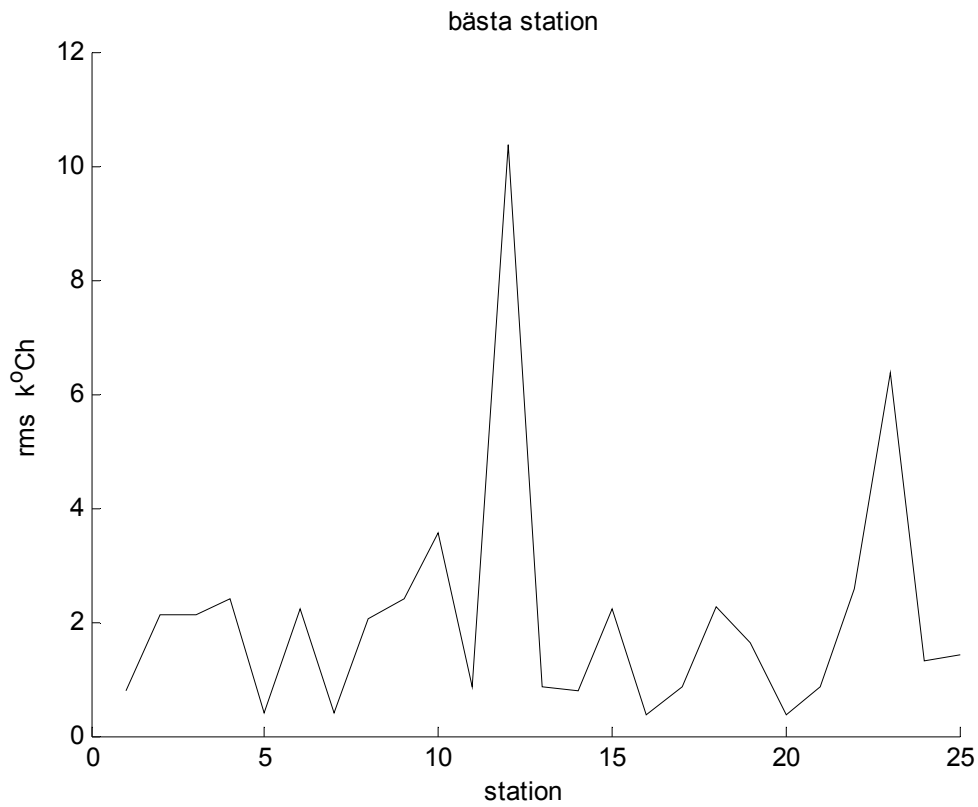
Figur 5.26 Rms i k^{\circ}Ch för bästa station, urval 0-25 ^{\circ}C och olika stationer.
