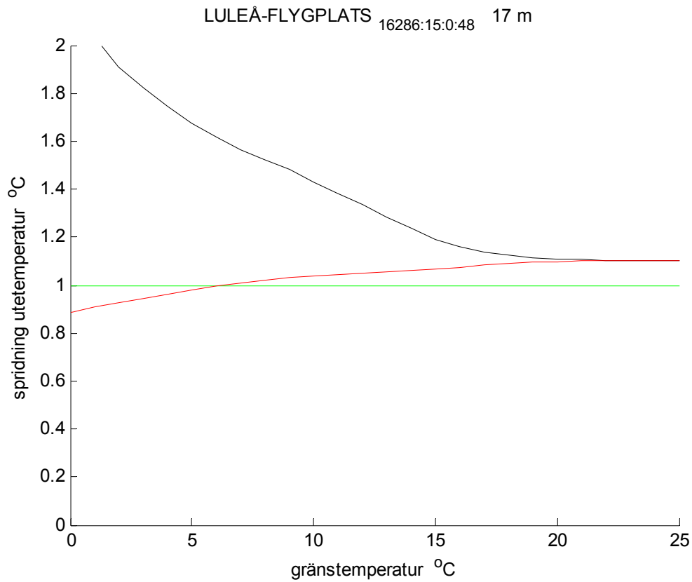
Figur 4.30 Spridning i utetemperatur beräknad med gradtimmar och drifttid eller 8760 h.
