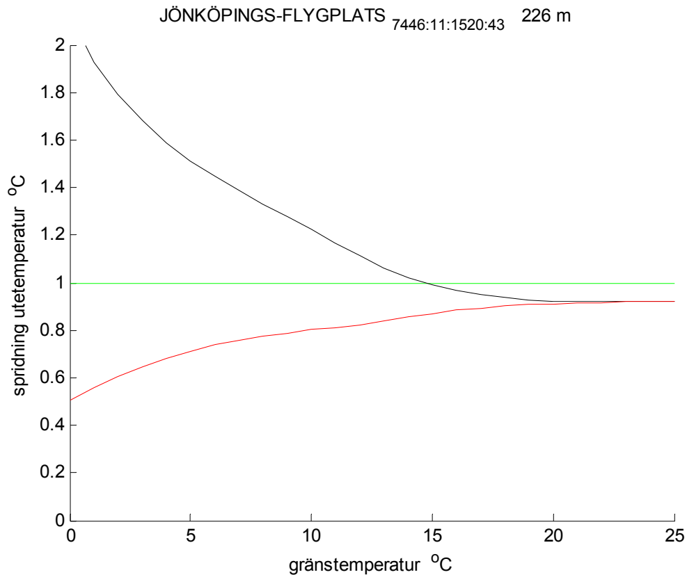
Figur 4.22 Spridning i utetemperatur beräknad med gradtimmar och drifttid eller 8760 h.
