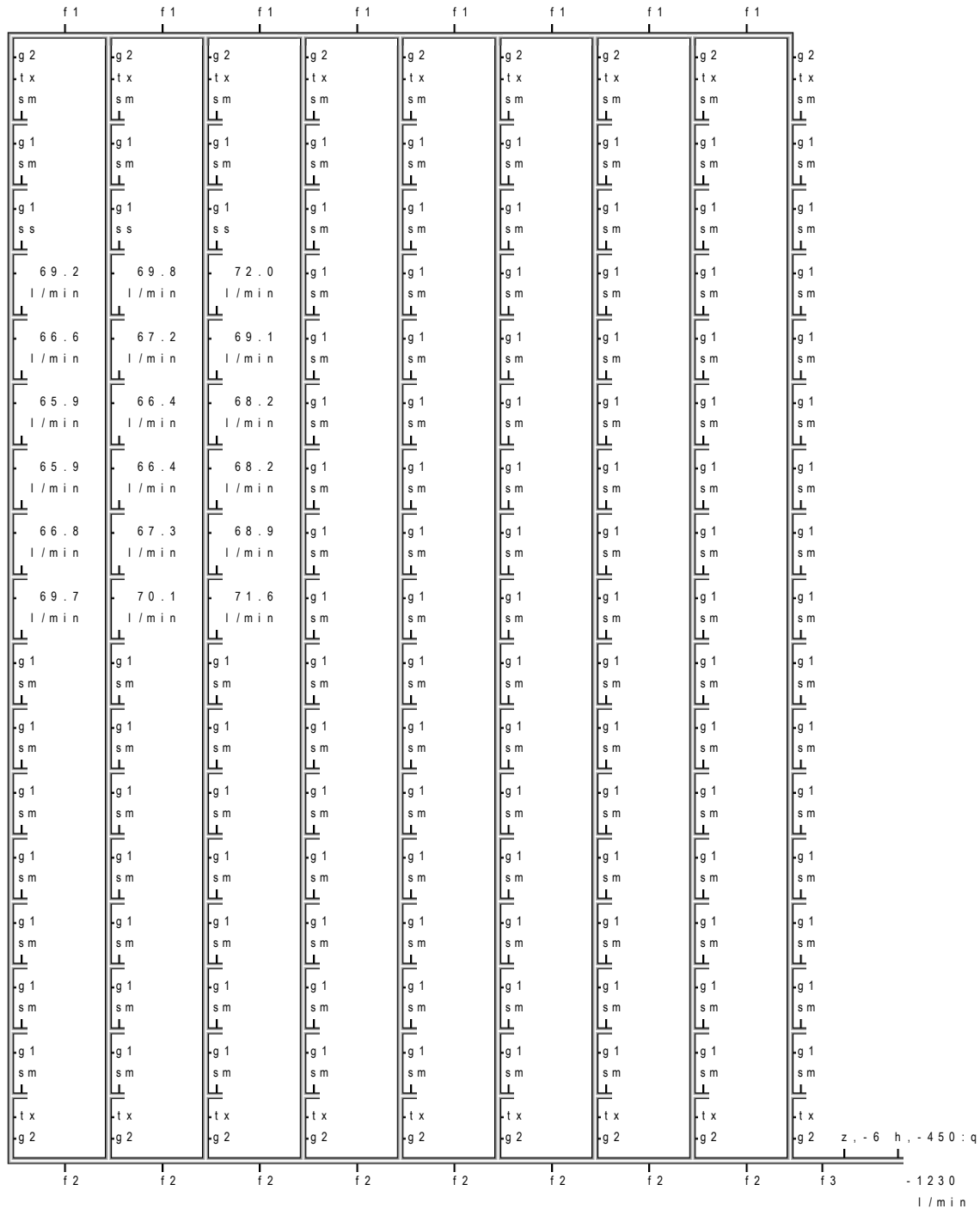
Figur 3.5 Gridrörssystem med en aktiv verkningsyta med arton sprinkler.
