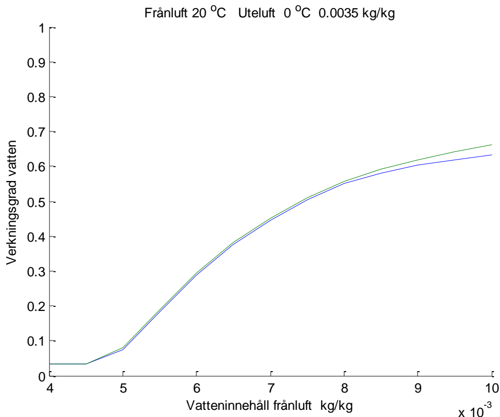
Figur 4.3 Fuktverkningsgrad som funktion av vatteninnehåll för frånluft.
