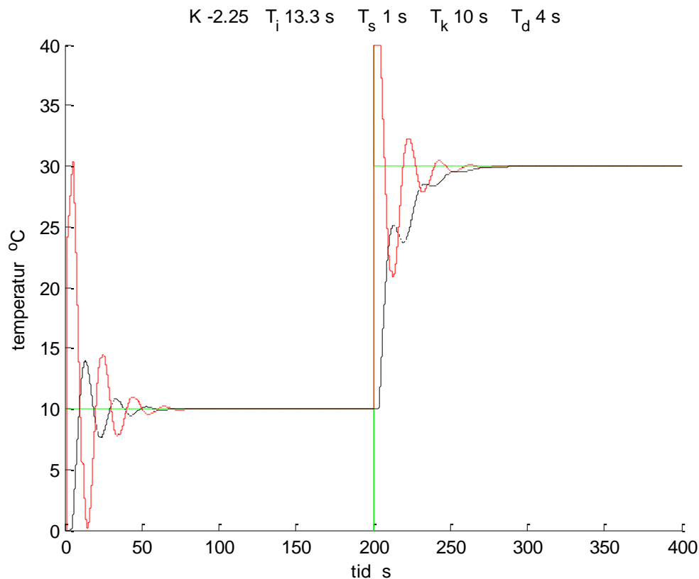
Figur 10.3 Tidsförlopp för PI-regulator inställd enligt stegvarsmetoden.
