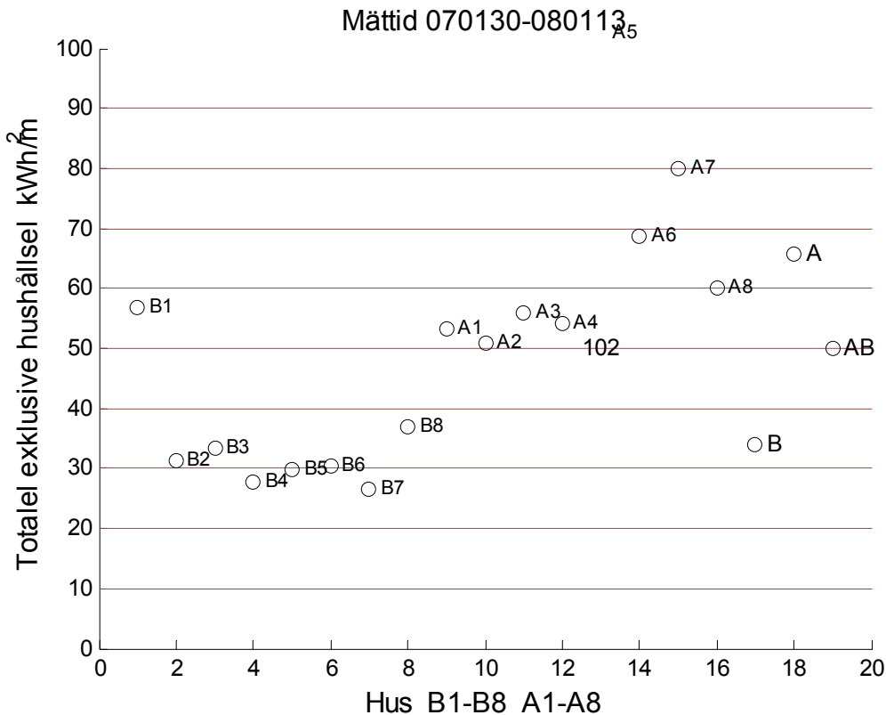
Figur 6.1 Totalelet exklusive hushållsel kWh/m 2 som funktion av husnummer.
