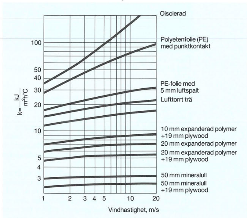
Figur 31. Ytöverföringstal som funktion av vindhastigheten för några olika isoleringsmaterial, anbringade på en betongyta /36/.
