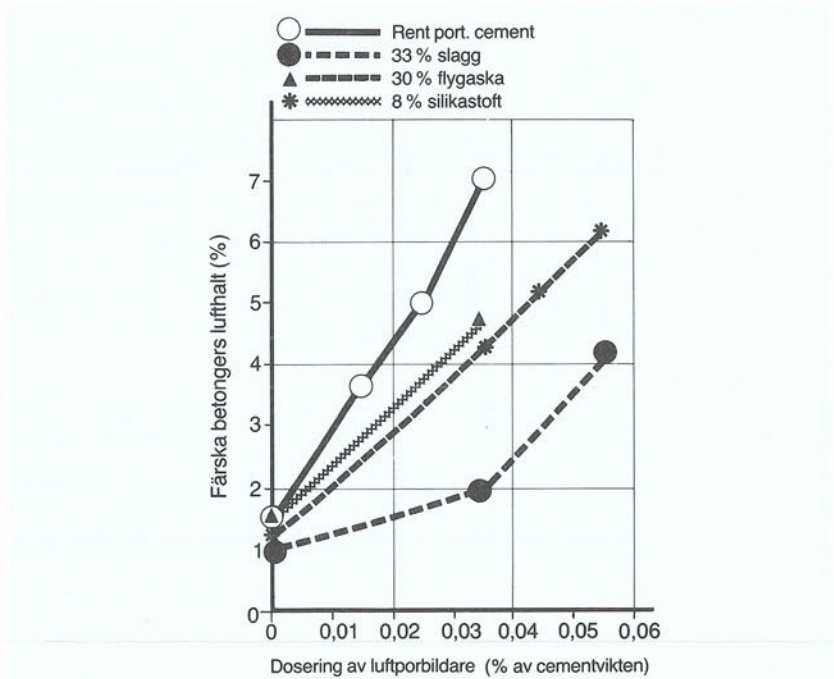
Figur 5. Exempel på inverkan av mineraliska tillsatsmaterial på behovet av luftporbildare. (Halten tillsatsmedel anges i relation till total bindemedelshalt) /11/.
