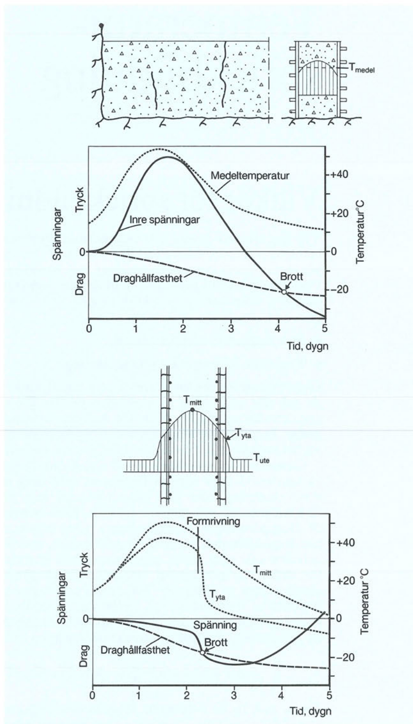
Figur 26. Olika typer av avsvainingssprickor. (a) Genomgående sprickor förorsakade av yttre fastlåsning. (b) Ytsprickor förorsakade av temperaturdifferenser över tvärsnittet.
