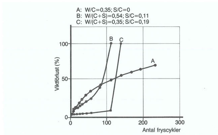
Figur 6. Saltfrystest av lufttillsatta betonger med och utan silikastoft, W=vatten, C=portlandcement, S=silikastoft /12/.
