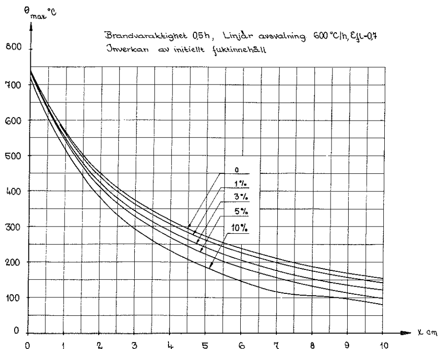
FIG. 26 c) \theta_{max} - x -kurvor vid \frac{1}{2} h brandvaraktighet, linjär av svalning 600°C/h, emissionsstal för flammorna \epsilon_{fl} = 0,7 och varierande initialt fukthåll, angivet i viktprocent.
