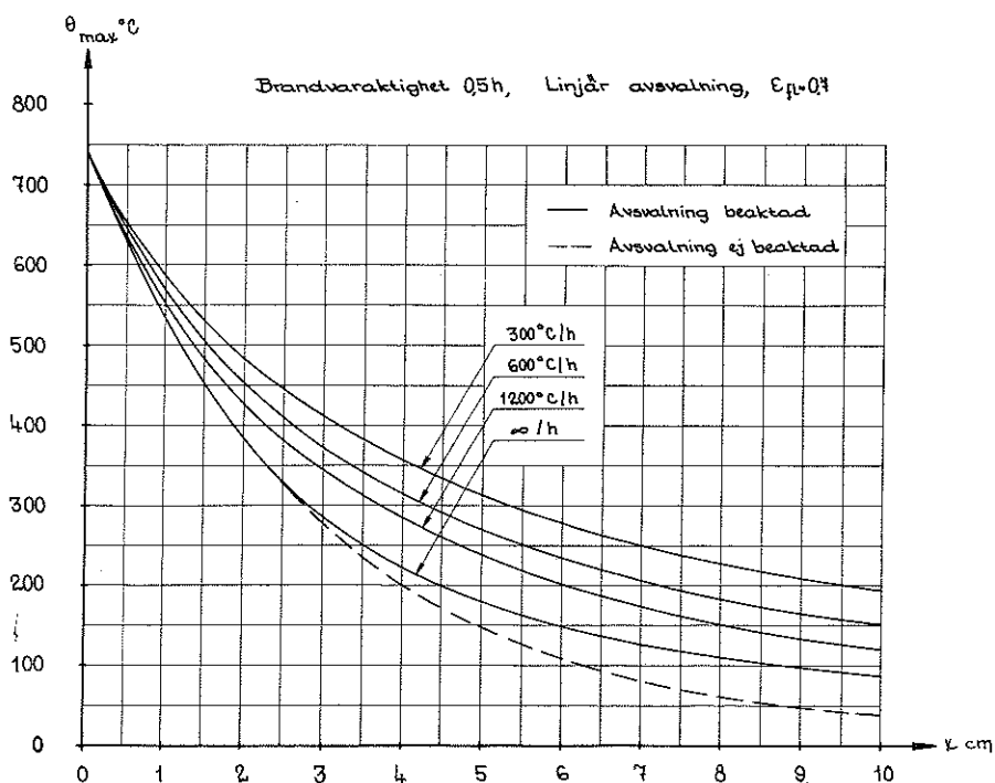
FIG. 26 b) \theta_{max} - x -kurvor vid \frac{1}{2} h brandvaraktighet, linjär av- svalning med varierande avsval- ningshastighet och emissionstal för flammorna \epsilon_{fl} = 0.7 för dels alternativet avsvalningsfasen beaktad (—) och dels alterna- tivet avsvalningsfasen ej be- aktad (---).
