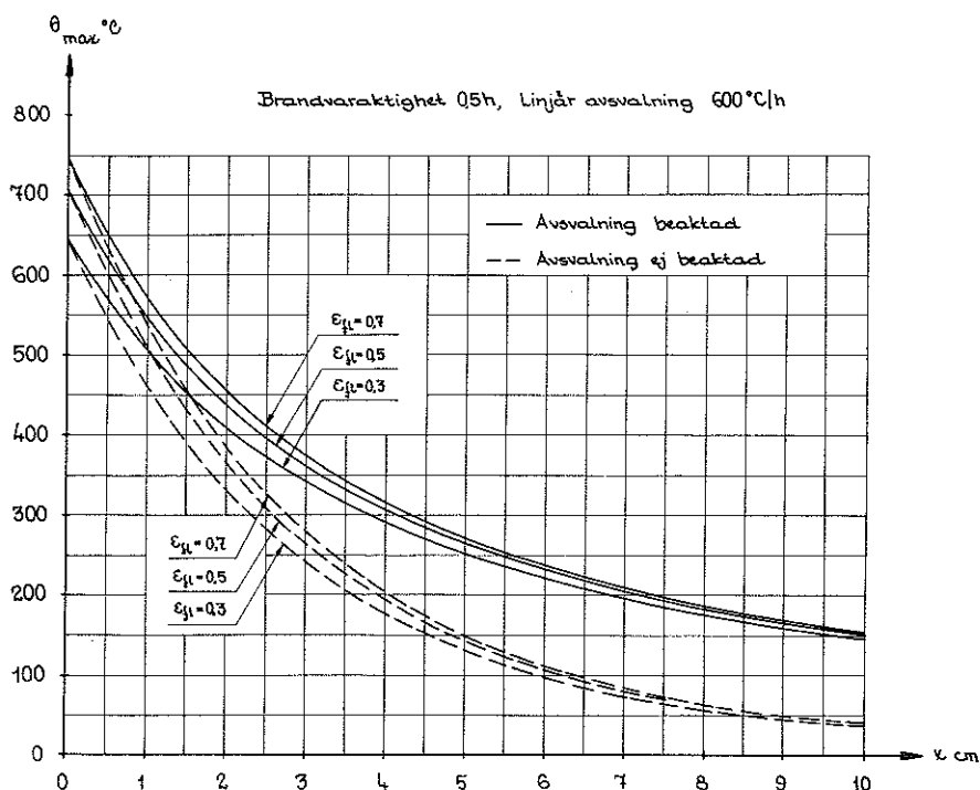
FIG. 26 a) \theta_{max} - x -kurvor vid \frac{1}{2} h brandvaraktighet, linjär av- svalning 600° C/h och varierande emissionstal för flammorna \epsilon_{fl} för dels alternativet avsval- ningsfasen beaktad (—) och dels alternativet avsvalningsfasen ej beaktad (---).
