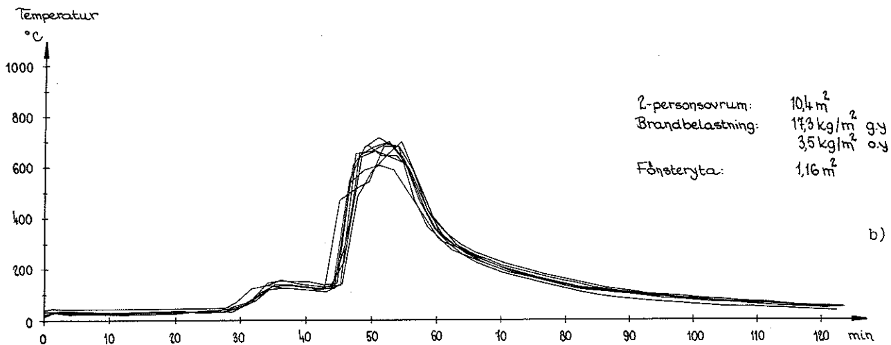
FIG. 6a och b. I olika punkter av tvåpersons sovrums med rums- och inredningskarakteristika enligt fig. a bestämd tidsvariation för gastemperaturen (fig. b) [Sjölin].
