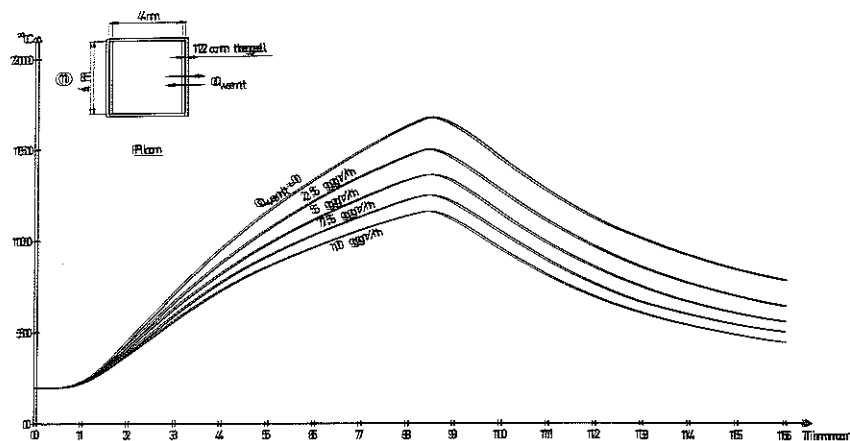
FIG. 19. Inverkan på temperatur-tidförloppet i en arkivlokal av varierande luftomsättning vid brand med varaktigheten 8 timmar mot en väggyta.
