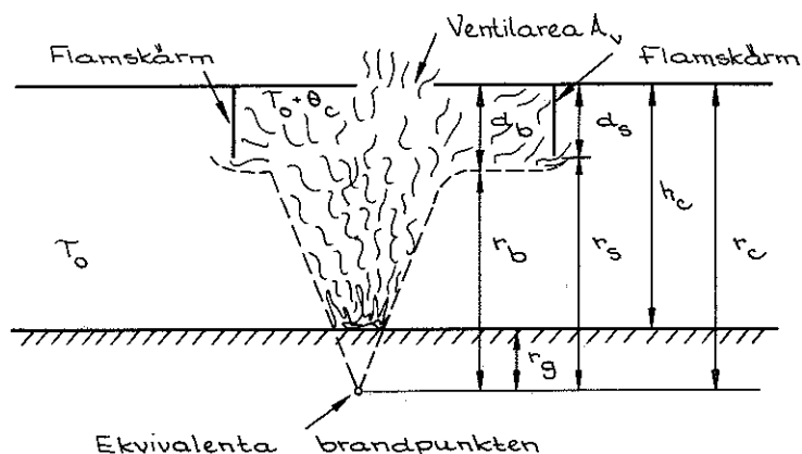
FIG. 15. Principfigur för brandventilation, definierande bl.a. ekvivalent brandpunkt, öppnings- eller ventilarea A_v , flamskärm samt brandgasskiktets tjocklek d_b [9].
