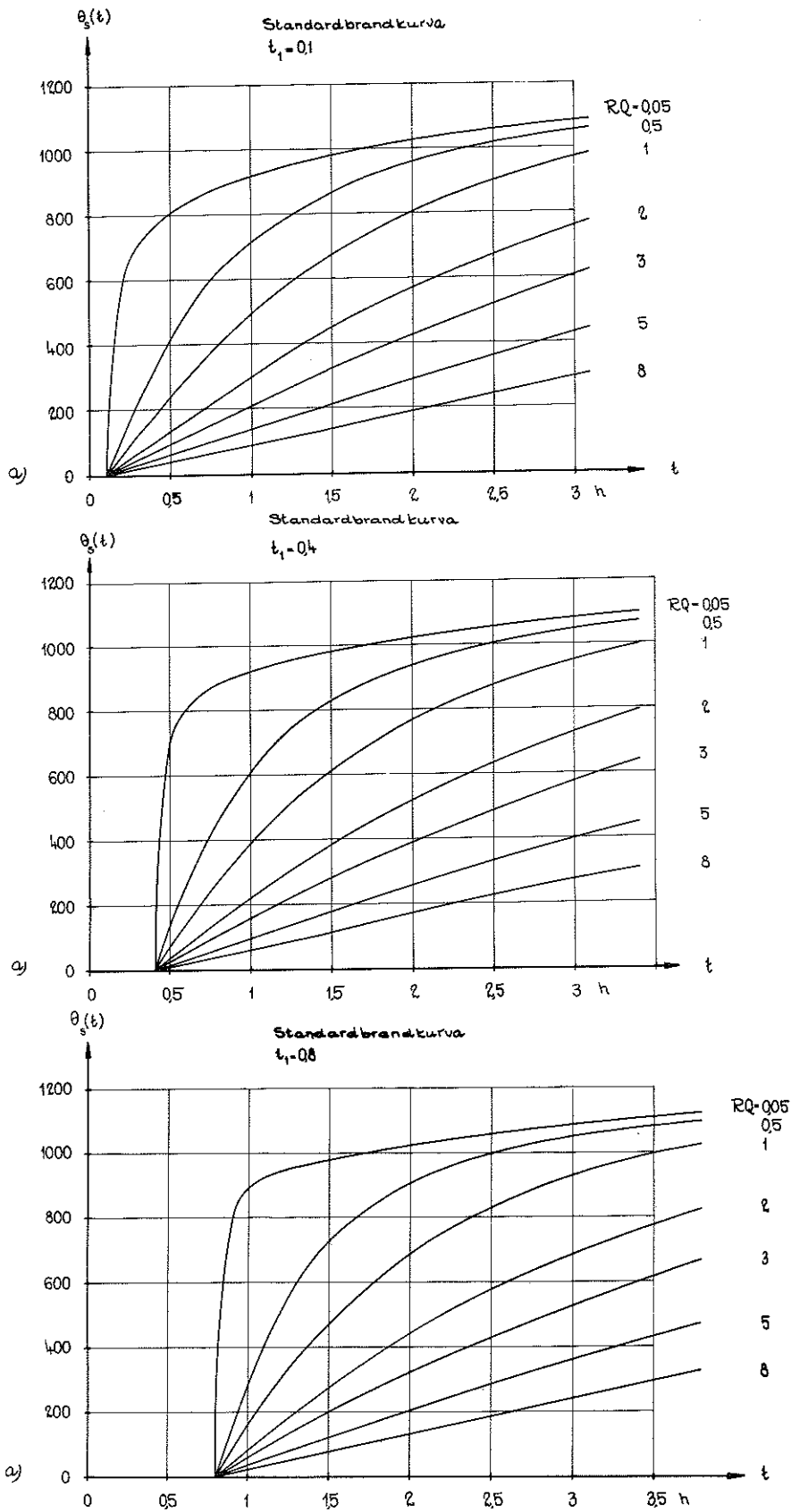
FIG. 28a och b. Teoretiskt beräknat samband mellan metalltemperatur \Theta_s och brandtid t för isolerat, metalliskt bärverk, utsatt för brandpåverkan med gas-temperatur-tidkurva enligt ekv. (4), fig. 28a, eller enligt den i fig. 21 för öppningsfaktorn A\sqrt{h}/A_c = 0,02 angivna kurvan, fig. 28b. Valda parametrar t_1 och RQ definieras ur ekv. (5) - (10) [16].
