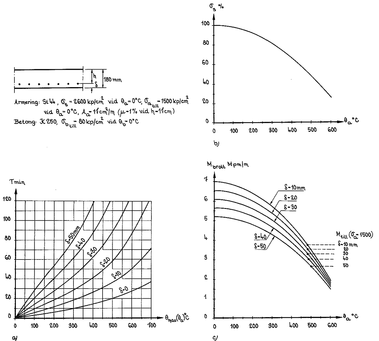
FIG. 27a-c. a) Beräknat samband mellan armeringsstångstemperatur \theta_{max}(\theta_a) och brandvaraktighet T vid varierande avstånd \delta mellan armeringsstångscentrum och brandutsatt yta för 18 cm tjock betongplatta, ensidigt brandpåverkad vid karakteristika, som approximativt överensstämmer med de för konventionell, normenlig brandteknisk provning gillande. b) För mjukt armeringsstål gällande, experimentellt bestämt samband mellan varmsträckgräns \sigma_s och temperatur \theta_a . c) För enkelspänd, enkelskiktad betongplatta med tjocklek 18 cm beräknat samband mellan brottböjmoment M_{brott} och armeringsstångstemperatur \theta_a vid varierande armeringsstångsnivå \delta . Sambandet förutsätter betong av kvaliteten K 250 och armering av St 44 med sträckgräns \sigma_s = 2600 \text{ kp/cm}^2 ( 260 \text{ N/mm}^2 ) vid \theta_a = 0^\circ\text{C} och armeringsmängd 1 % vid den effektiva höjden h = 17 \text{ cm} . I figuren markeras också för temperaturen 0^\circ\text{C} tillåtet böjmoment M_{till} vid tillåten betongtryckspänning \sigma_b = 80 \text{ kp/cm}^2 ( 8 \text{ N/mm}^2 ) och tillåten armeringsdragspänning \sigma_a = 1500 \text{ kp/cm}^2 ( 150 \text{ N/mm}^2 ).
