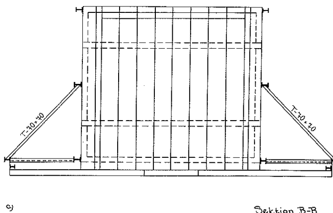
FIG. 11. Utformning av försöksbhus för studium av brand- och rökspridning längs fasad och vertikal ventilationskanal vid brand i en viss våning i en flervåningsbyggnad.
