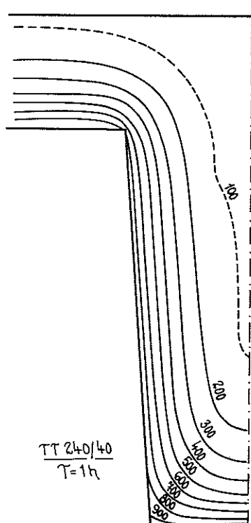
◀ FIG. 24. Beräknat temperaturfält i underifrån brandutsatt TT-platta enligt fig. 22 vid en timmes standardiserat brandprov.
