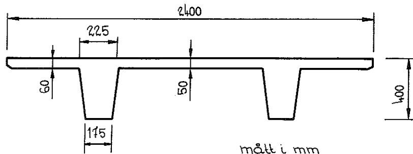
FIG. 22. Exempel på tvärsnittsutförande av TT-platta av betong. Example of cross section of a double T concrete slab.
