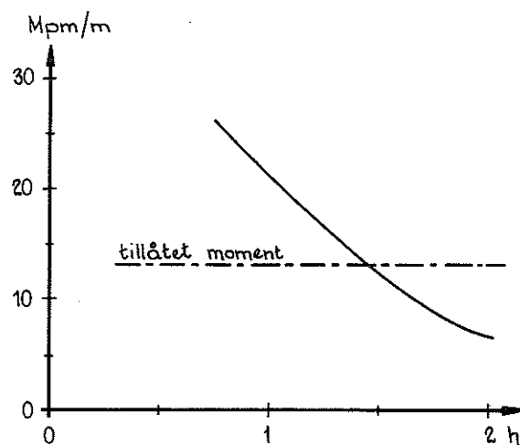
▲ FIG. 25. Beräknat samband mellan brandprovningstid och böjmomentkapacitet för TT-platta enligt fig. 22.
