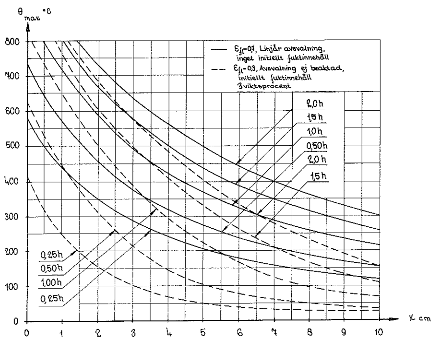
FIG. 26 d) \theta_{max} - x -kurvor vid varierande brandvaraktighet, linjär av svalning 600°C/h, emissionsstal för flammorna \epsilon_{fl} = 0,7 och inget initialt fukthåll (—), jämförda med motsvarande \theta_{max} - x -kurvor vid emissionsstalet för flammorna \epsilon_{fl} = 0,3 , 3 viktprocent initialt fukthåll och av svalningsfasen ej beaktad (---) [18].
