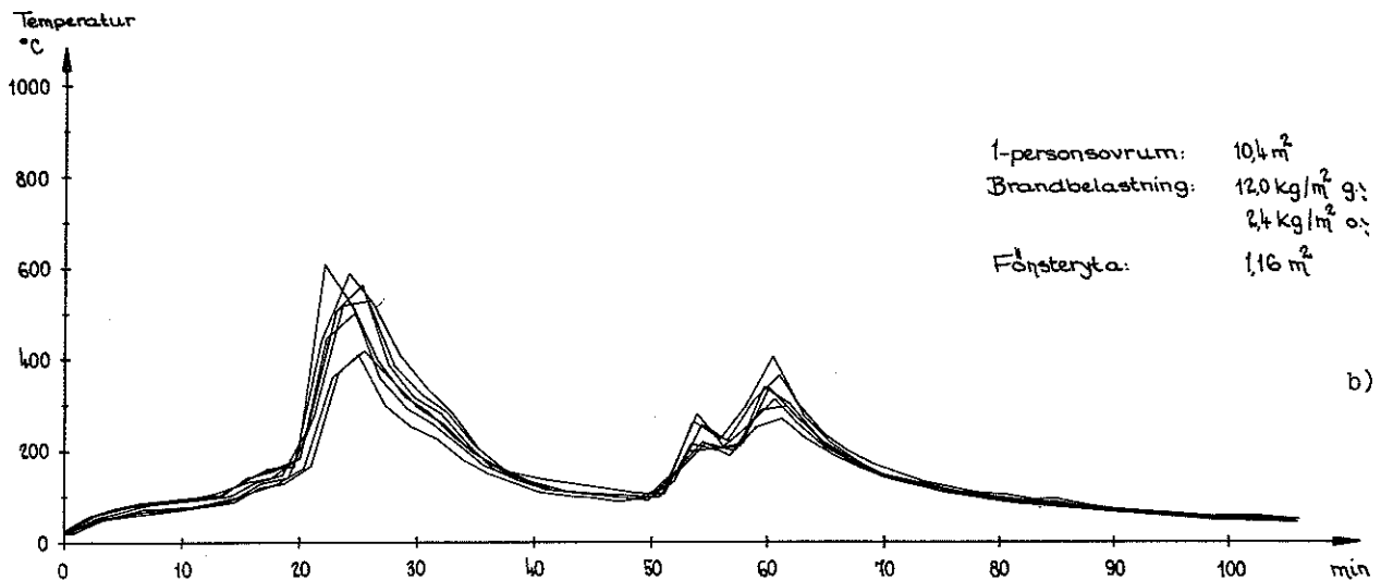
FIG. 9a och b. I olika punkter av en persons sovrums med rums- och inredningskaraktistika enligt fig. a bestämd tidsvariation för gastemperaturen (fig. b) [Sjölin].
