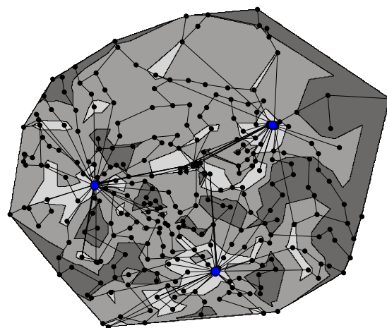
Figur 3. Sårbarhetskarta som, i tre nivåer, visar hur sårbar elförsörjningen är olika områden av elnätet. De ljusare områdena är mindre sårbara än de mörkare. De blå noderna är inmatningspunkter och de svarta är noder med kunder kopplade till sig.
