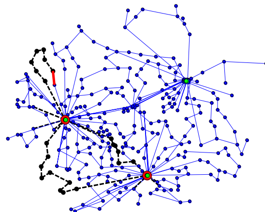
Figur 4. Exempel på identifikation utav kritiska komponenter. I figuren har tre komponenter ur funktion markerats i röd färg, vilket ger konsekvensen 5870 kunder utan elförsörjning (15 MW icke-levererad effekt). De noder och länkar som är utan elförsörjning är markerade i svart färg. De gröna noderna är inmatningsnoder till elnätet.
