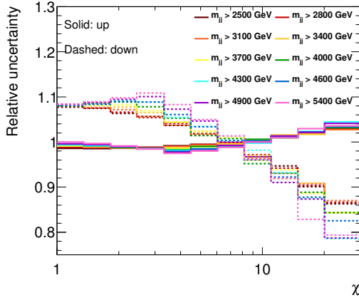
(b) \sqrt{s} = 13 \text{ TeV}
