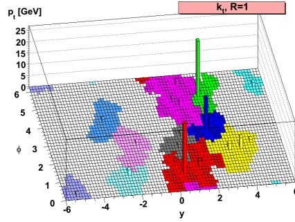
(a) k_t
