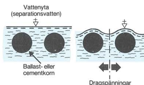
Plastiska krympsprickor.
