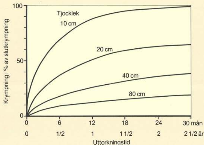
Samband mellan konstruktionstjocklek och uttorkningskrympning.
