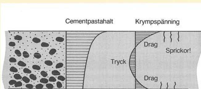
Stenseparation kan medföra ytsprickbildning.
