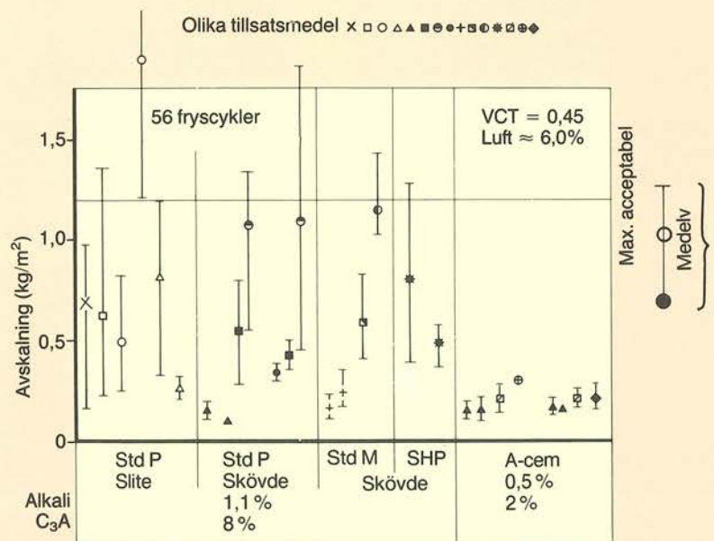
Inverkan av cementsorten på saltfrostbeständigheten /10/. (vct = 0,45 och lufthalten = 6 % i alla betonger.)
