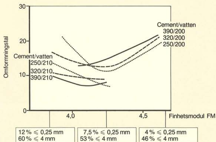
Mätningar vid Betongcentrum i Malmö /4/. Betong utan tillsatsmedel, Std P, 16 mm stenstorlek
