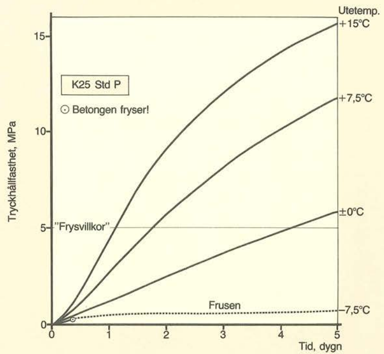
(b) 16 cm bjälklag, oisolerad plywoodform, gjuttemperatur +15 °C
