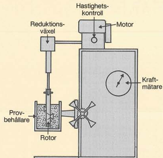
Vridmoment
