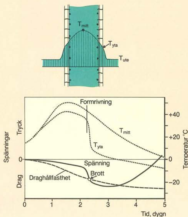
Ytsprickbildning.
