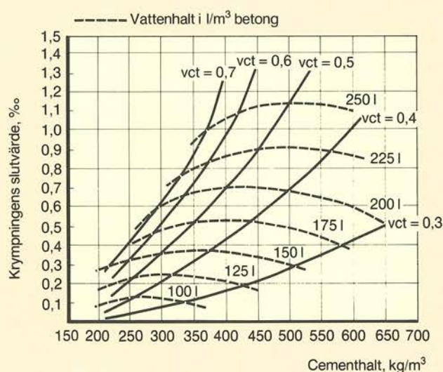
Samband mellan krympning vid 50 % relativ fukt och mängden blandningsvatten /21/.
