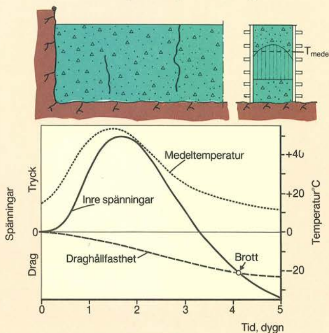
Genomgående sprickbildning.
