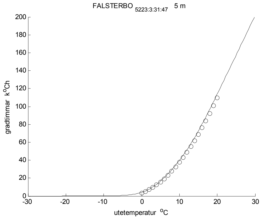
Figur 4.59 Uppmätt och förenklad °Ch-funktion för utemperaturen för Falsterbo.
