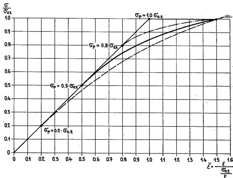
Fig 4. \sigma - \varepsilon -kurvor, valda som utgångspunkt för ett studium av knäckningsspänningens \sigma_k variation med materialets proportionalitetsgräns \sigma_p
