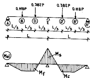
Fig 7. Balk- och belastningsutformning för experimentellt gränslaststudium av statiskt obestämmd aluminiumbalk. För elastiska förhållanden gällande kvot mellan stödmoment M_s och maximalt fjälmoment M_f uppgår till 2,25
