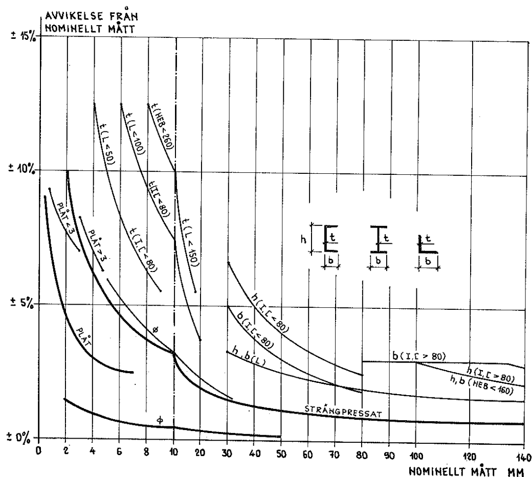
Fig 14. För formvaror av aluminium (—) och stål (—) representativa dimensionstoleranser
