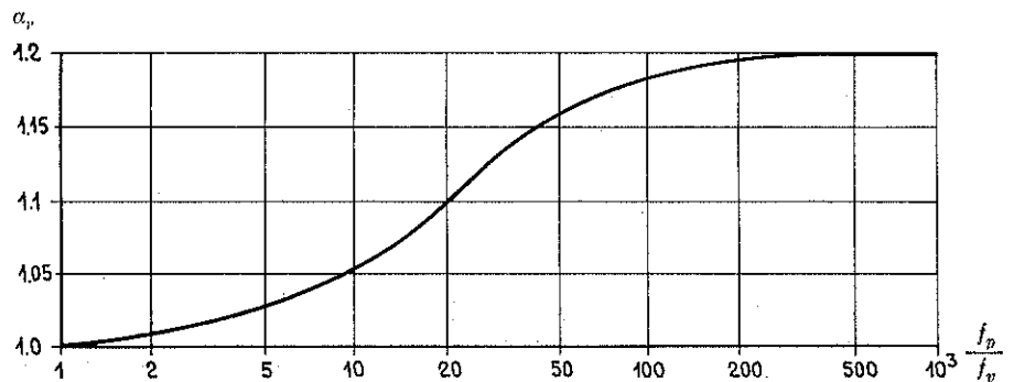
Fig 12. Förhållande \alpha_v mellan genom provning bestämd och till verkligt belastningsfall hörande dynamisk brottspänning som funktion av förhållandet mellan provningsmaskinens frekvens f_p och verkligt belastningsfalls frekvens f_v
