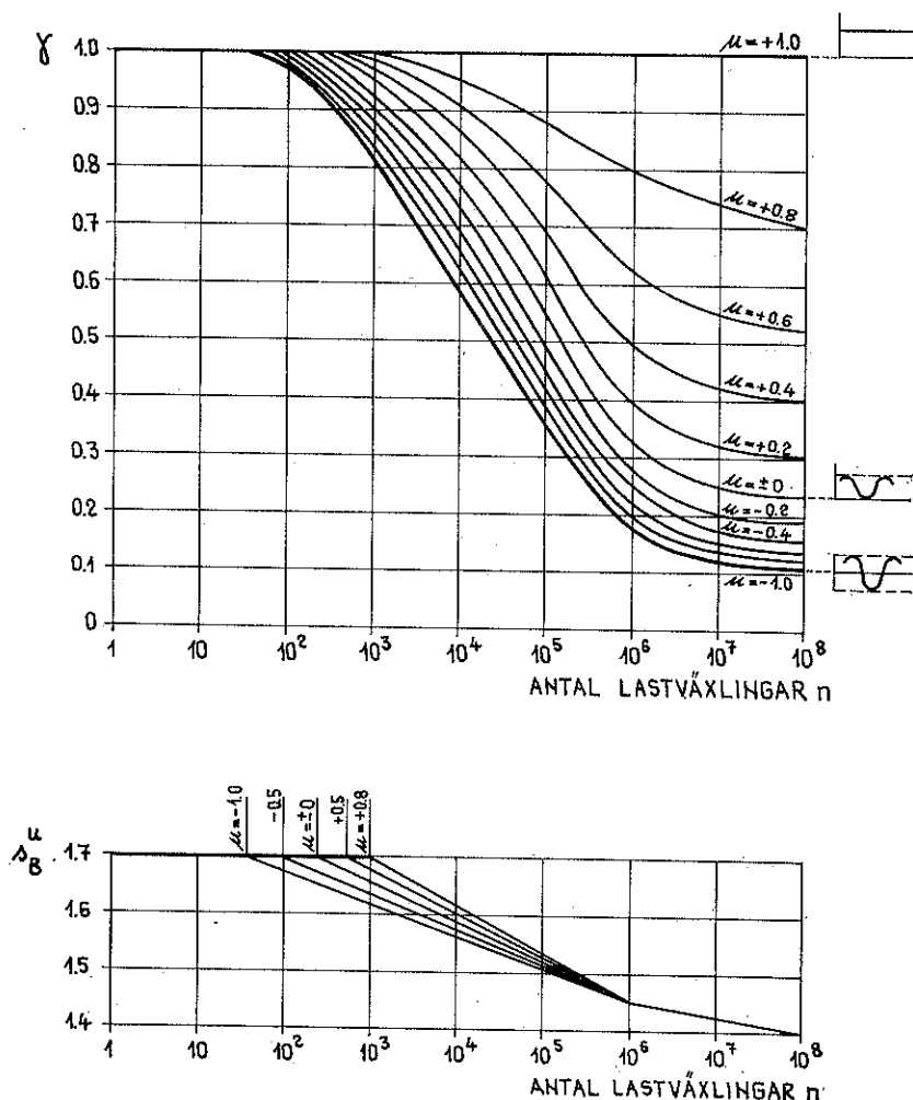
Fig 16. Reduktionsfaktor \gamma = \sigma_{Bn} / \sigma_{B_{N=1}} och säkerhetsfaktor s_B^u för grundmaterial av legeringen AlZn4Mg. \mu = \sigma_{\min} / \sigma_{\max} ; \tau_{\min} / \tau_{\max} . Provningsmaskinens frekvens = 110 p/s
