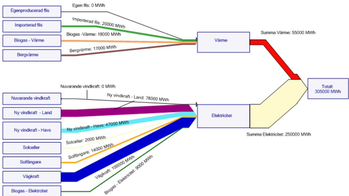
Figur A7. Sankey-diagram över energitillförsel för scenario Intensiv om de gamla vindkraftverken byts ut. En större mängd elektricitet kan tillföras från land och färre vindkraftverk behöver placeras till havs.
