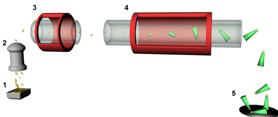
Figur 2. Illustration av tillverkningstekniken Aerotaxi där nanotrådar växer utan ett substrat. Det börjar med att guldpartiklar förångas (1) och storlekssorteras (2). Efter detta skickas de genom en ugn för att få en jämn rund form (3) innan växtmaterial tillförs i växtkammaren(4) och trådarna bildas. Efteråt kan nanotrådarna deponeras på ett valfritt substrat (5).
