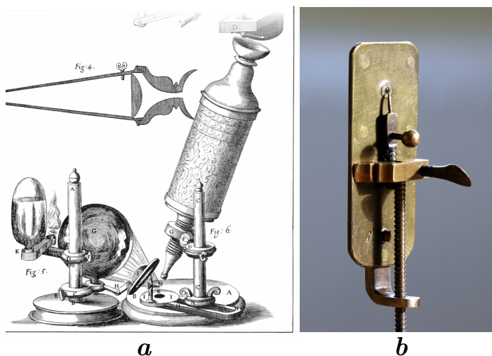
Figur 1: (a) Robert Hookes egna skiss av sitt mikroskop, från boken Micrographia [138]. Instrumentet var ca 30 cm högt. (b) Replika av Antonie van Leeuwenhoeks lupp, som är ca 5 cm hög. Foto Jeroen Rouwkema, licens Creative Commons BY-SA.
