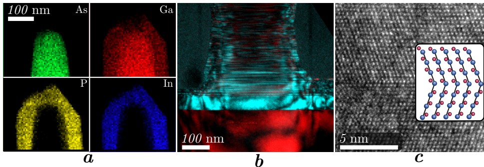
Figur 8: Olika transmissionselektronmikroskopitekniker applicerade på tvärsnitt av nanostrukturer för granskning i sidovy [I]. (a) Kartläggning med hjälp av energiuppplöst röntgenspektroskopi av olika grundämnen som finns i toppen av en nanostruktur. (b) Gränssytan mellan nanostrukturen och substratet avbildad i mörkfältsläge där det går att skilja mellan olika kristaller (blått och rött i bilden). (c) En liten del av samma gränssyta avbildad med högupplöst transmissionselektronmikroskopi. De två kristallerna möts mitt i bilden och en modell av kristallerna är infogad till höger i bilden.
