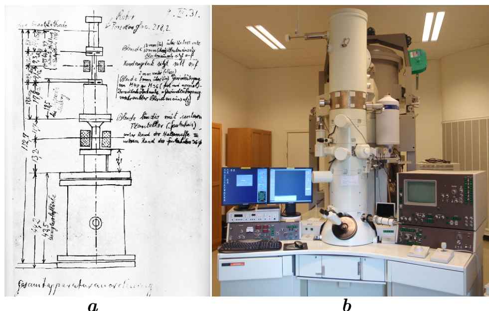
Figur 2: (a) Ernst Ruskas egen skiss av ett tänkt transmissionselektronmikroskop, daterad den 9 mars år 1931. © The Nobel Foundation 1986. (b) Ett transmissionselektronmikroskop av modell 3000F, tillverkat av JEOL (ursprungligen Japan Electron Optics Laboratory). Mikroskopet finns vid National Center for High Resolution Electron Microscopy (nCHREM) i Lund. Instrumentet är ca 2.5 m högt.
