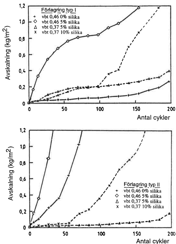
Figur 13.5:7. Saltavskalning hos betong med olika vbt och olika mängd silikastoft förbehandlade på två olika sätt; Hammer & Sellevold (1990). Betong 65 och 65S; vbt=0,46 . Betong 95 och 95S; vbt=0,37 . "Curing condition I": 1 månad i luft+1 månad i havsvatten. "Curing condition II": Förseglad i formen 1 månad+1 månad i havsvatten.
