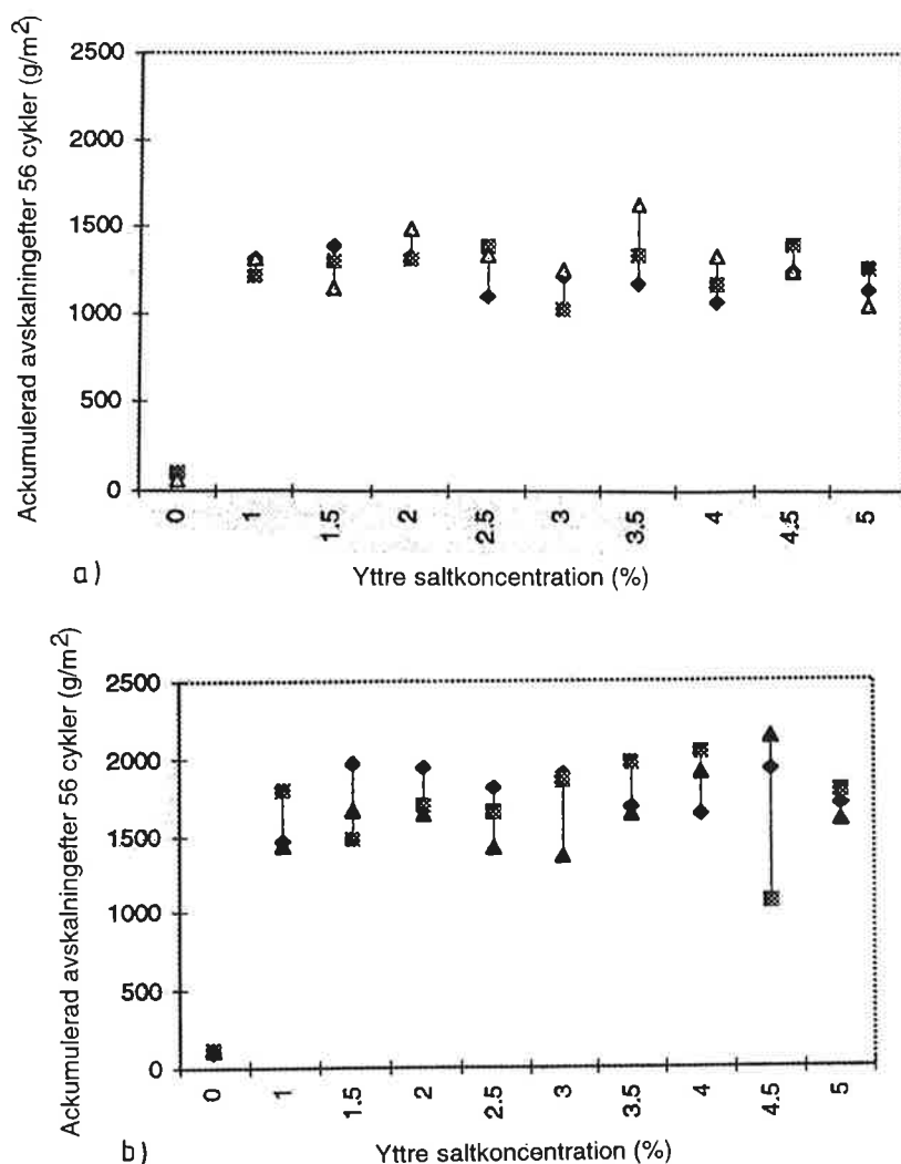
Figur 13.5:4. Inverkan av yttre salthalt på saltavskalningen hos betong med vbt=0,34 och 5% sili-kastoft; Lindmark (1995). (a) Prover som aldrig torkats. (b) Prover som utsatts för en enda uttork-nings-uppfuktningscykel.
