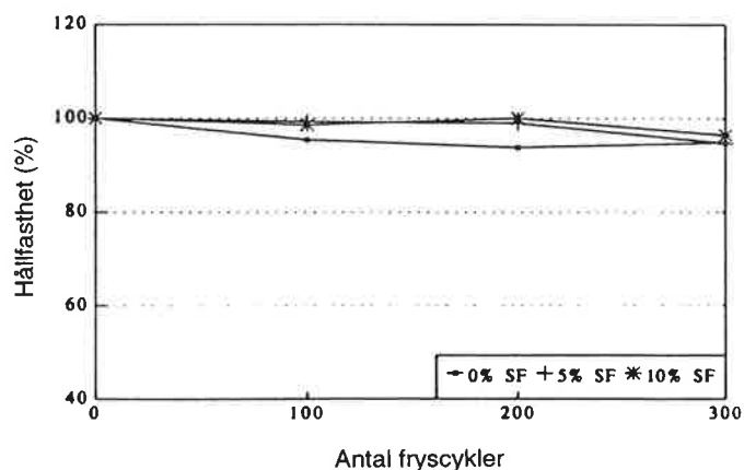
Figur 13.6.5. Inverkan av mängden silikastoft på frostbeständigheten hos betong med konstant w/b=0,24 ; Li et al (1994). Frysprovning av typ ASTM C 666, Metod A. Figure 13.6.5. Influence of the amount of silica fume on the frost resistance of concrete with constant water-binder ratio 0.24. Test method ASTM C 666 Method A. Li et al (1994).
