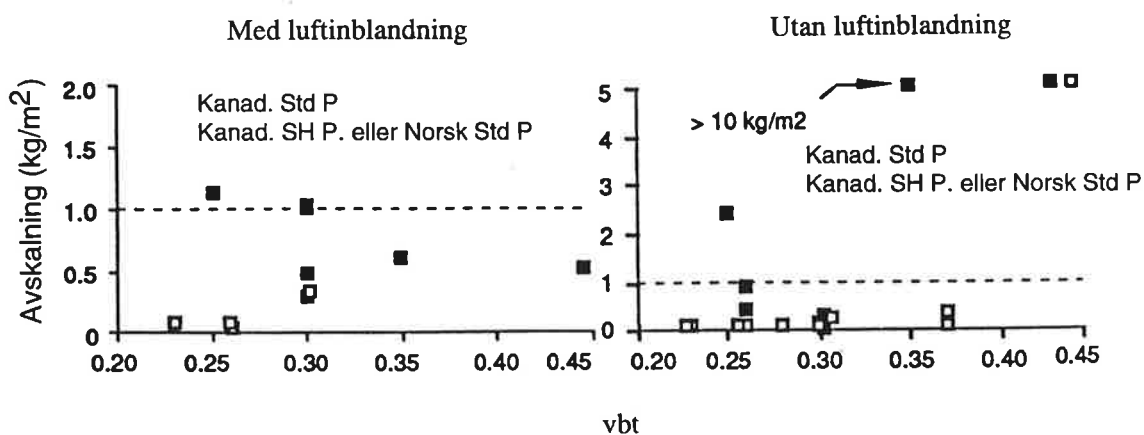
Figur 13.5:11. Sammanställning av resultat av saltfrysprovning av betong med olika vct och med 5 % till 10 % silikastoft; Gagné & Marchand (1997). Resultat efter 100 cykler.
