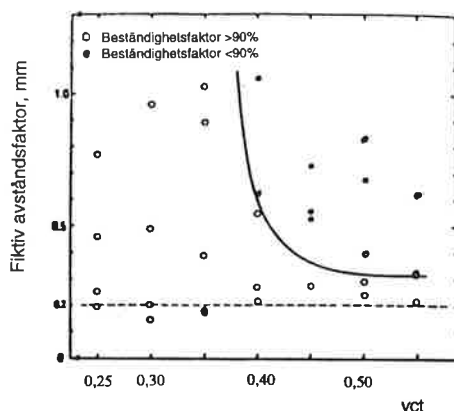
Figur 13.3:1. Samband mellan den kritiska fiktiva avståndsfaktorn och vct ; Okada et al (1981). Resultat efter 300 cykler med frysprovningmetod ASTM C 666.
