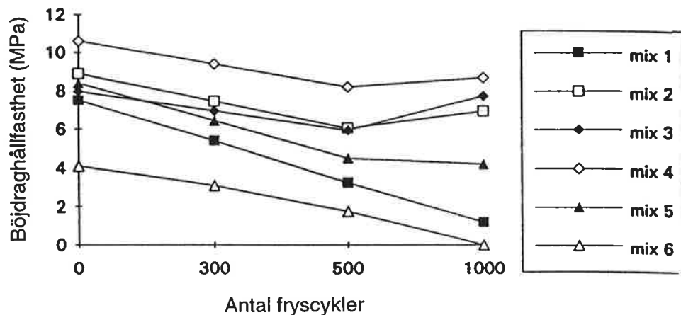
Figur 13.6.2.: Böjdraghållfasthet hos icke lufttillsatt betong med olika v_{ct} som funktion av antalet fryscykler; Kukko (1995). Frysprovning av typ ASTM C 666, Metod B. Beträffande olika "Mixer" se tabell 13.6.2.
