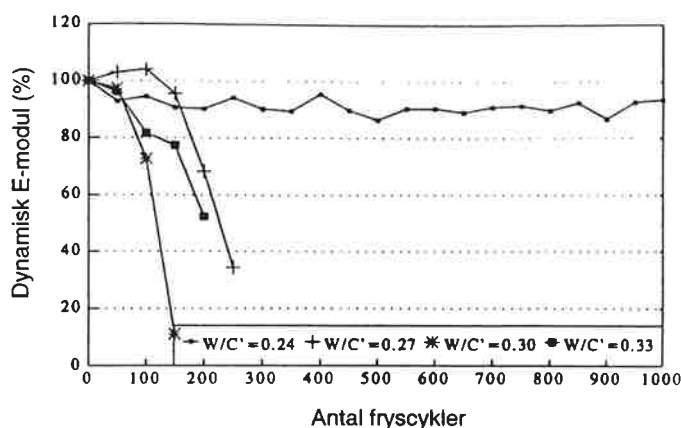
Figur 13.6.4. Dynamisk E-modul som funktion av antalet fryscyklar hos icke lufttillsatt betong med olika w/c och utan silikastoft; Li et al (1994). Frysprovning av typ ASTM C 666, Metod A. Figure 13.6.4. Dynamic E-modulus as function of the number of freeze-thaw cycles of non-air-entrained concrete with various water-cement ratio and no silica fume. Test method ASTM C 666 Method A. Li et al (1994).
