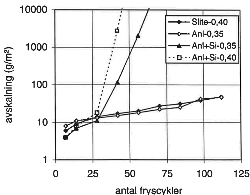
Figur 13.5:13. Saltfrysprovning av icke lufttillsatt betong som utsatts för en naturlig åldring under tre år. Olika cementsorter (Slite Std och Anläggningscement) och olika v_{bt} (0,35 och 0,40). Med och utan silikastoft (Si). Åldrad yta utgör frysyta i testen. Petersson (1995).
