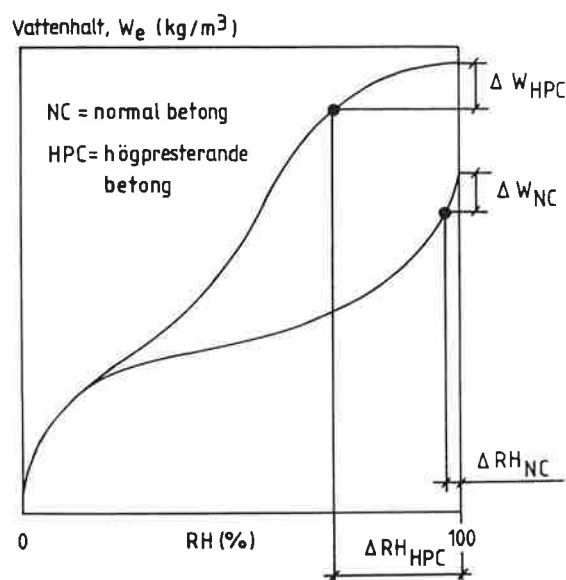
Figur 13.4:6. Principiellt utseende hos sorptionsisotermen hos normalbetong och högrepresterande betong. Inverkan av självuttorkningen på RH. \Delta RH är självuttorkningen förorsakad av hydratationen \Delta W . NB är normalbetong. HPB är högrepresterande betong.
