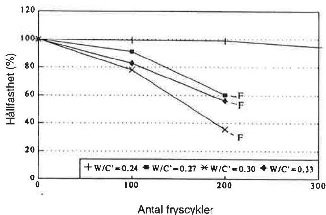
Figur 13.6.3. Tryckhållfastheten som funktion av antalet fryscyklar hos icke lufttillsatt betong med olika w/c och utan silikastoft; Li et al (1994). Frysprovning av typ ASTM C 666, Metod A. Figure 13.6.3. The compressive strength as function of the number of freeze-thaw cycles of non-air-entrained concrete with various water-cement ratio and no silica fume. Test method ASTM C 666 Method A. Li et al (1994).
