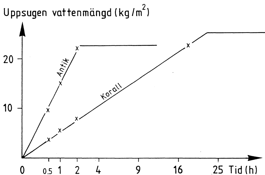
FIGUR 3.1:1. Teglets kapillärsugningsegenskaper.
