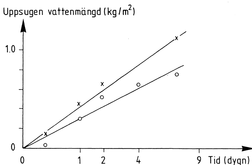
FIGUR 3.4:1. Vattenupptagning då impregnering gjorts med utspädda preparat på blöta ANTIK-stenar.
