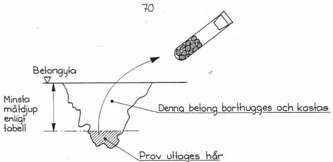
Fig 9.1 Principiellt provtagningsförfarande.
