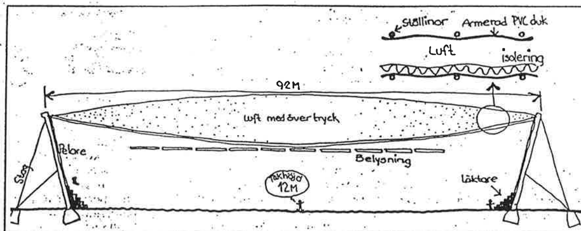
Figur 4.1. Takkonstruktion med ställinor och armerad PVC-duk för stora spännvidder [13].
