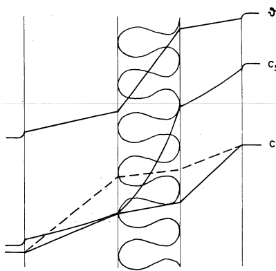
Fig. 42. Kondensation i en sandwichkonstruktion.
