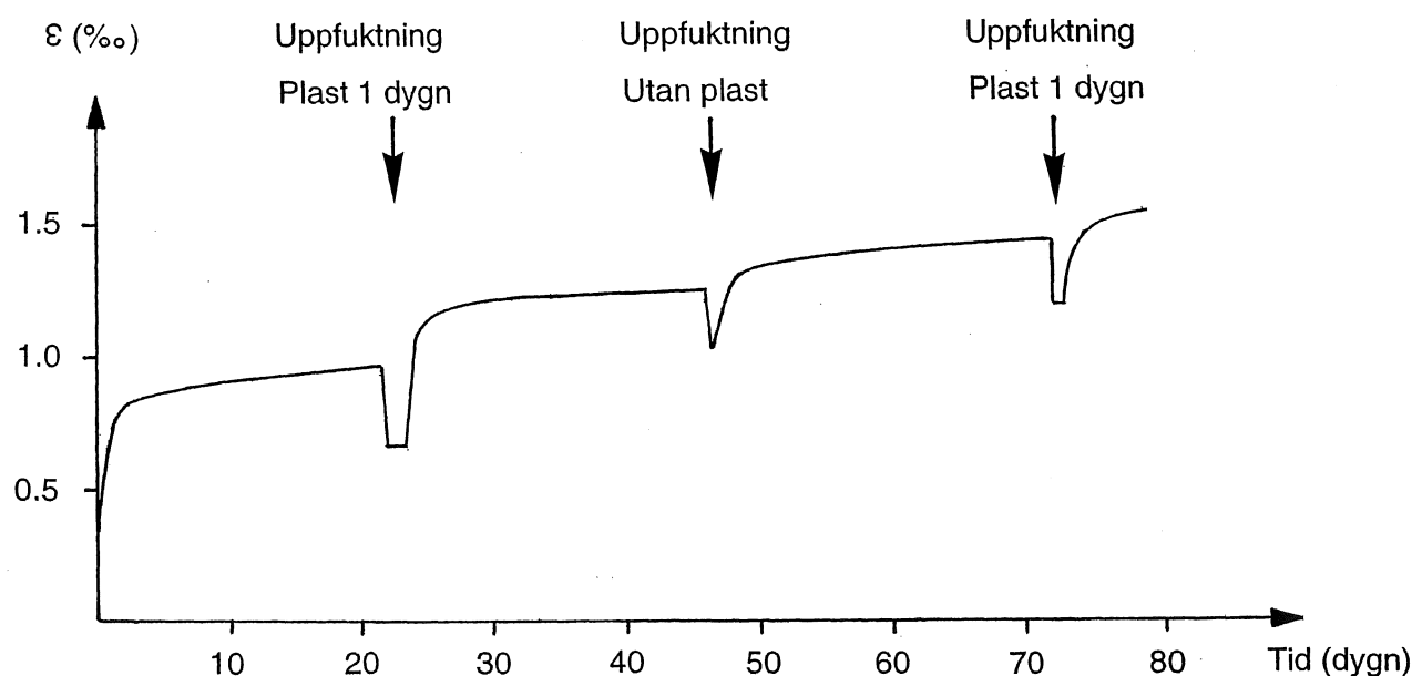
FIGUR 19. Krympning under hela mätperioden, SERPO 136.
