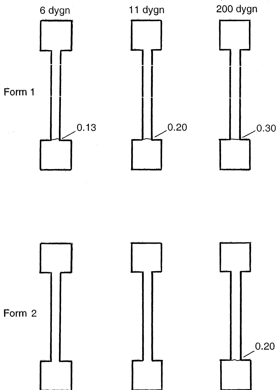
FIGUR 14. Spricktillväxt i plexiglasformar FGB 8500 MF.
