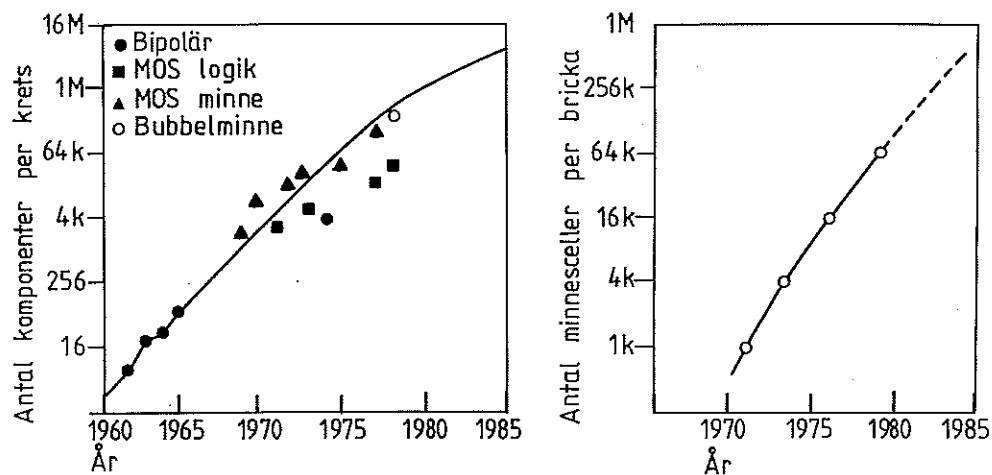
Fig. 1 - Utveckling av packningstätheten för mikroelektronik.
