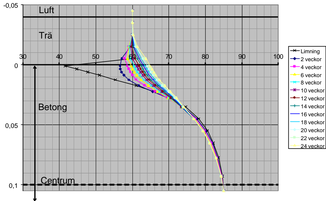
Figur 6. Omfördelning av kvarvarande byggfukt då trägolvs direktlimmas på byggfuktfri betong som först torkat 24 veckor.
