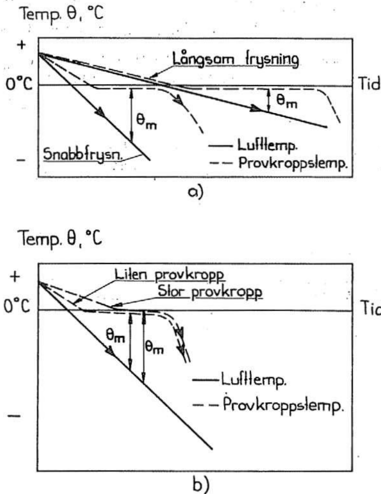
FIG 58 Principiell inverkan av provkroppsstorlek och temperatursänkningshastighet på temperaturdifferens luft-provkroppsytta. Influence of specimen size and rate of temperature lowering on temperature difference air-specimen.
