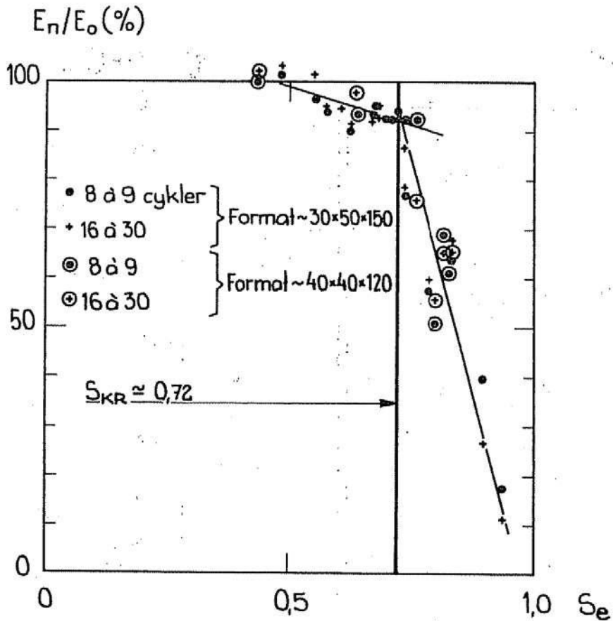
FIG 149 Material nr 15. Sarabondbruk vct=0,488. Cement mortar w/c-ratio=0,488.
