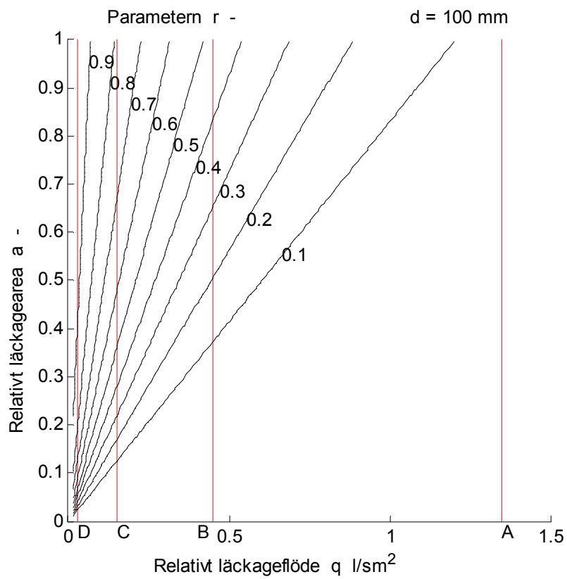
Figur 4.8 Kvoten U_d/U_s för 100 mm isolering.
