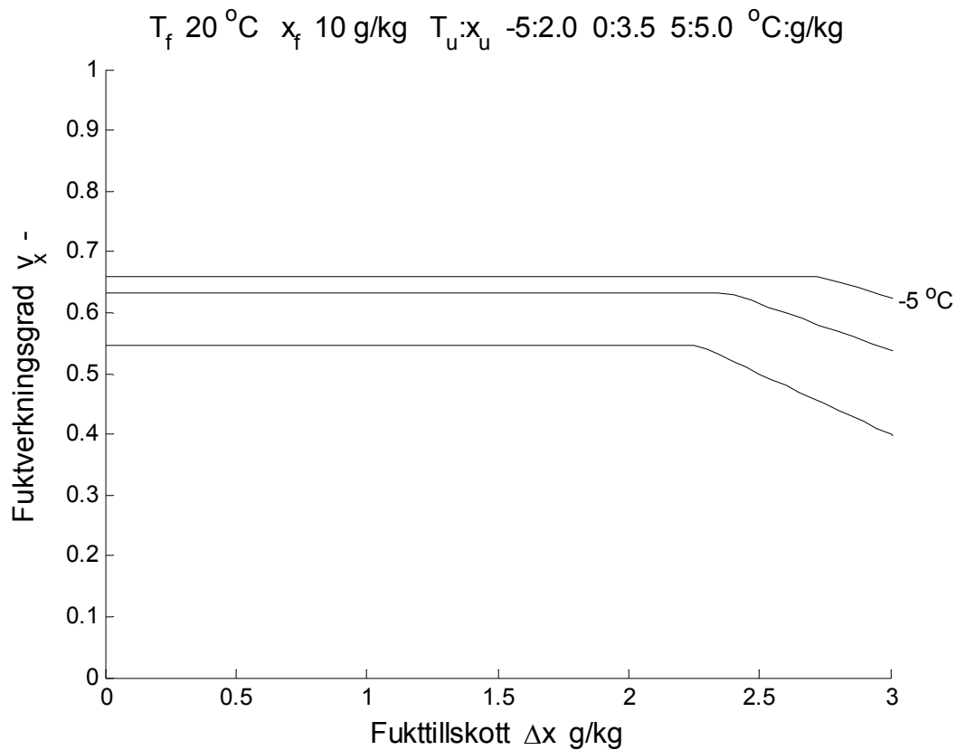
Figur 10.2 Fuktverkningsgrad v_x - som funktion av fukttillskott för x_f 10 g/kg olika klimat.
