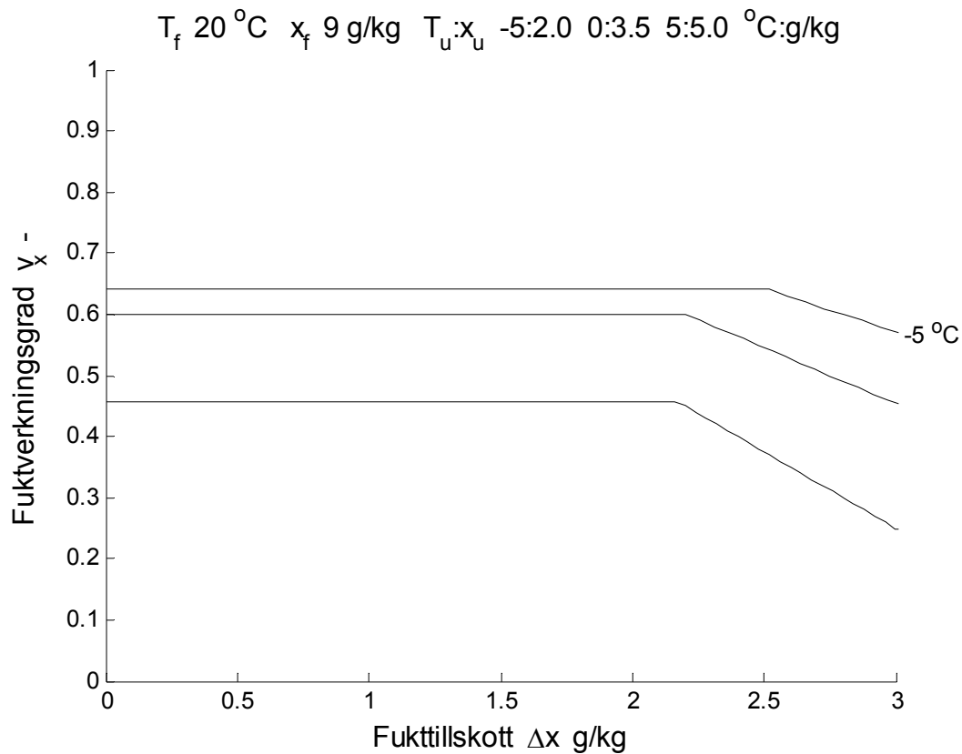
Figur 9.2 Fuktverkningsgrad v_x - som funktion av fukttillskott för x_f 9\text{ g/kg} olika klimat.
