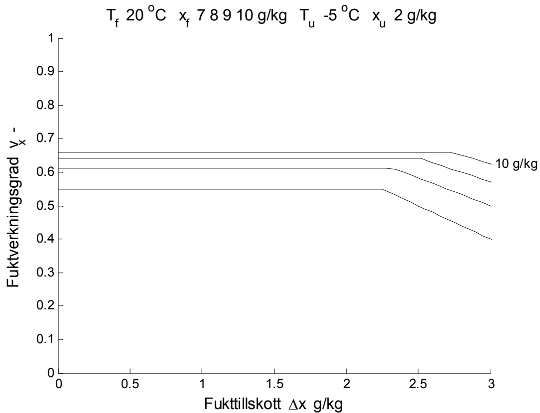
Figur 4.2 Fuktverkningsgrad v_x - som funktion av fukttillskott för x_f 7, 8, 9 och 10 g/kg.
