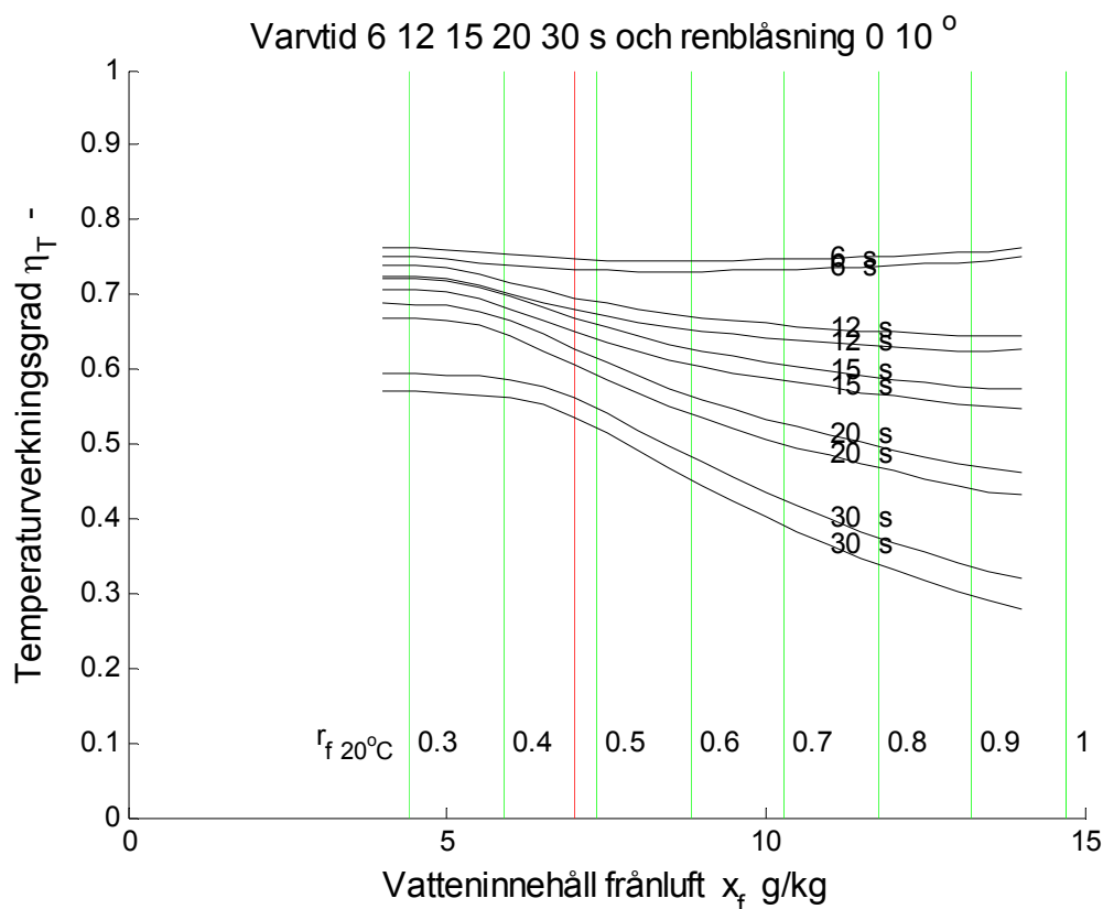
Figur 3.1 Temperaturverkningsgrad \eta_T – som funktion av x_f\text{ g/kg} och olika varvtid.
