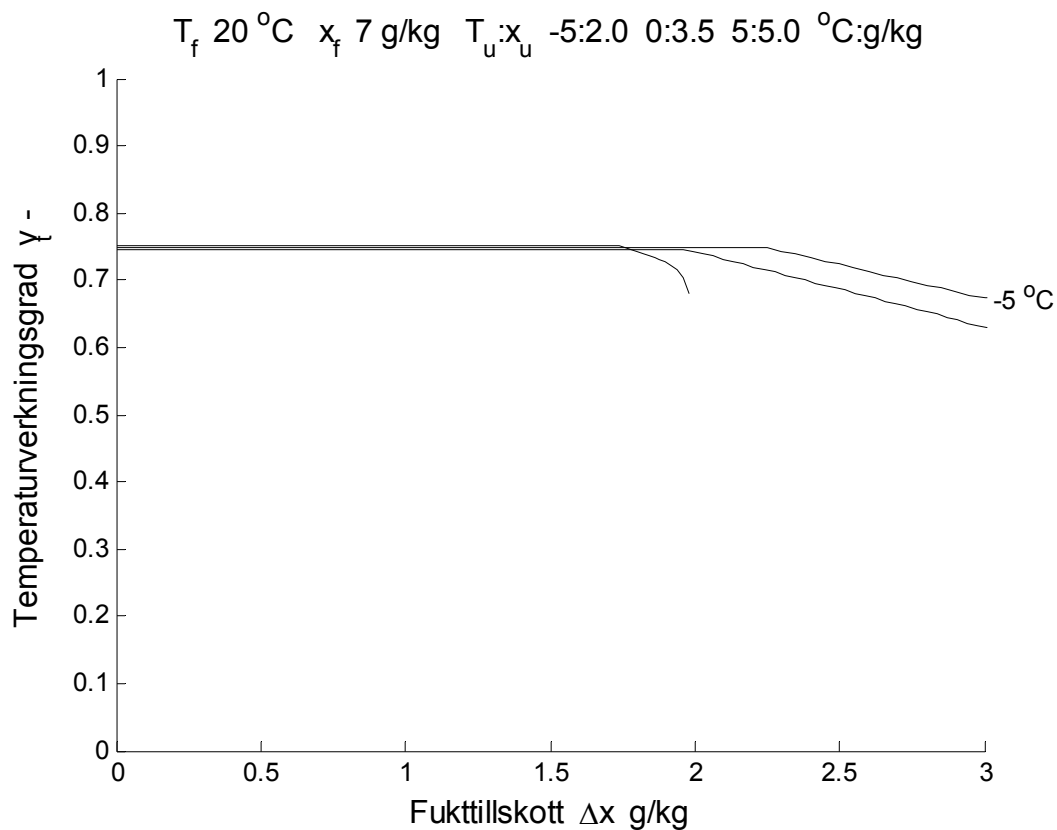
Figur 7.3 Verkningsgrad v_t - som funktion av fukttillskott för x_f 7 g/kg och olika klimat.
