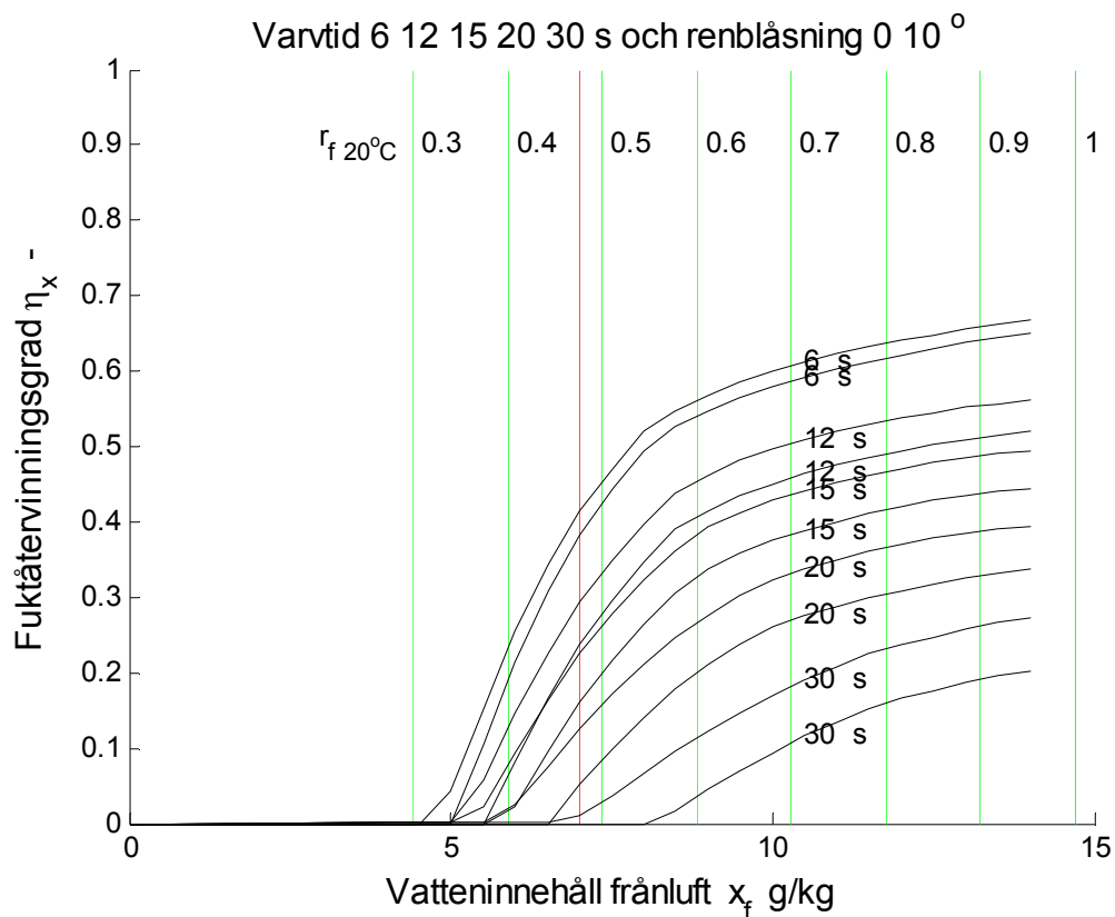
Figur 3.2 Fuktverkningsgrad \eta_x – som funktion av x_f g/kg och olika varvtid.
