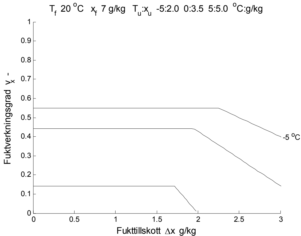
Figur 7.2 Fuktverkningsgrad v_x - som funktion av fukttillskott för x_f 7 g/kg olika klimat.
