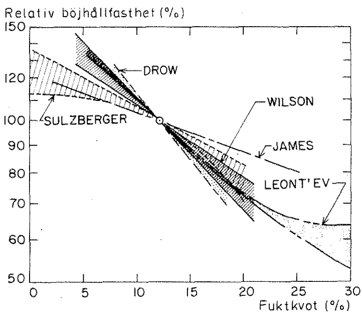
Figur 5.3 Effekt av varierande fuktkvot på böjhållfastheten vid 20 o C. 100% vid fuktkvoten 12% /5.1/
