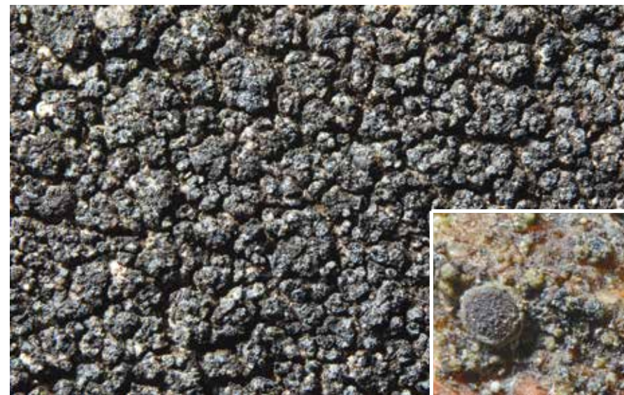
Fig. 4. Halecania giraltiae , ny för Skandinavien. Små mörkt blågrå soralar är typiska. Apothecierna (infälld bild) är sällsynta men fanns också fläckvis. Foto U. Arup.
