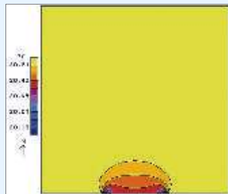
Figur 4: Global operativ temperatur.
